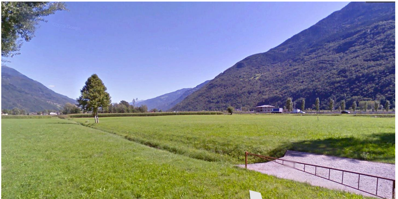
FOTO 7 – Tratta 1: vista del tratto di connessione della VS03 con la viabilità RFI in progetto. In questo tratto è previsto l'adeguamento con sezione Tipo A.
