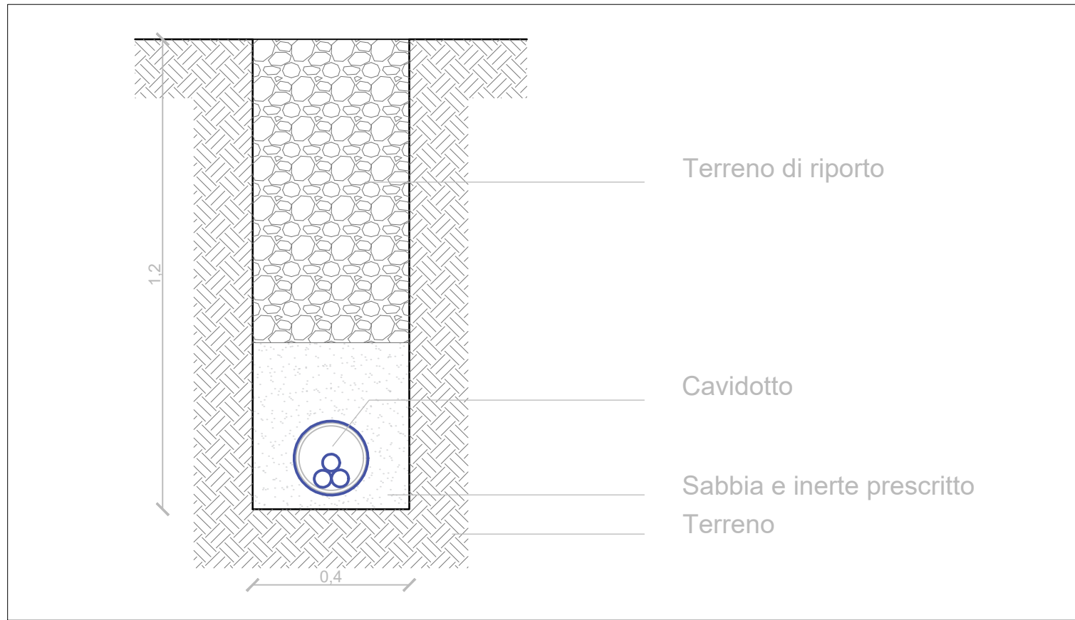
SEZIONE CAVIDOTTO
