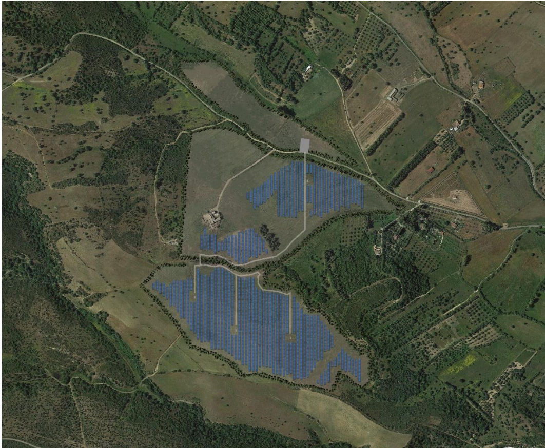
Fig 1: Planimetria impianto in fase di esercizio.
