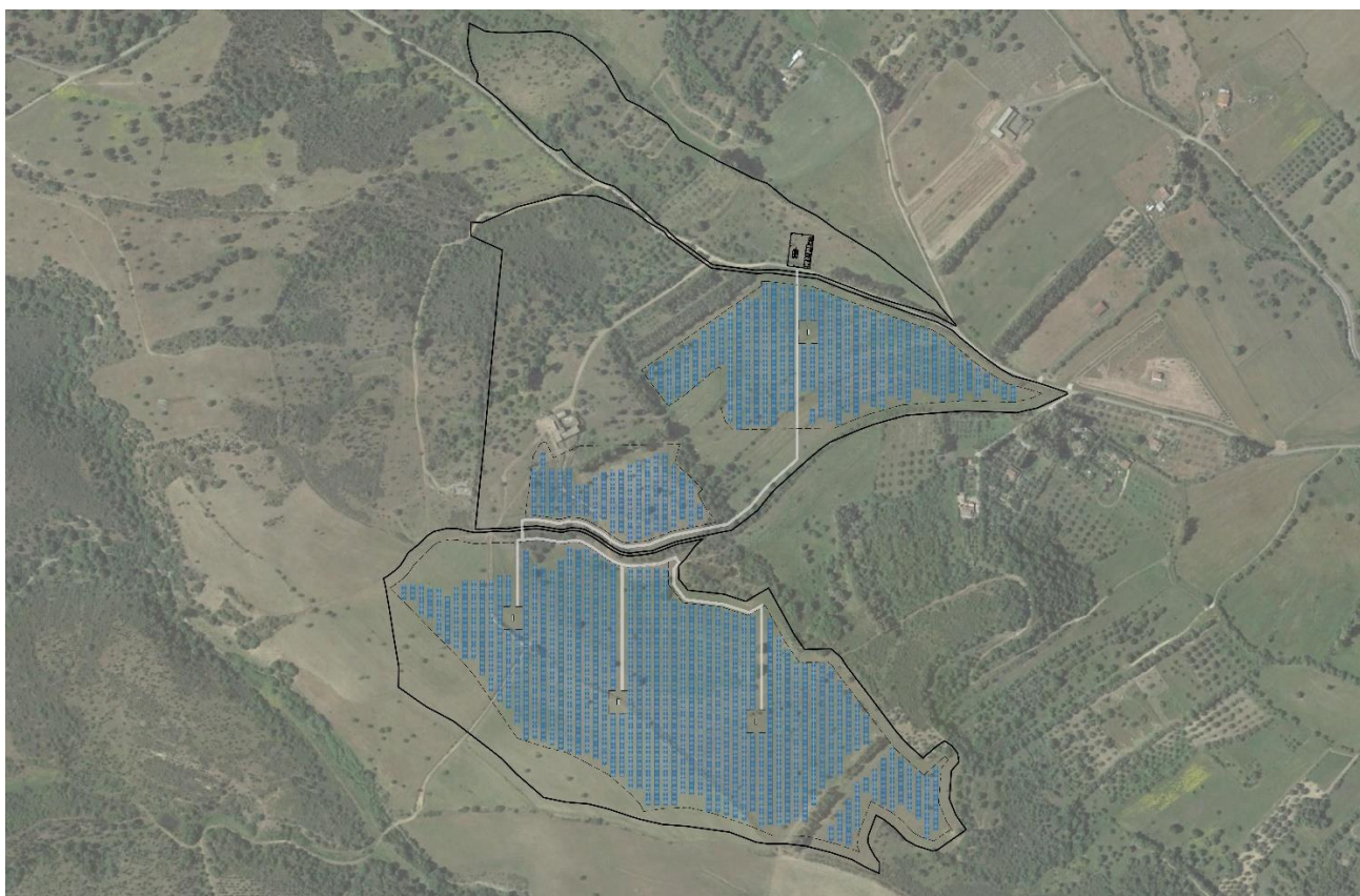
Fig. 8: Area di intervento con layout.
