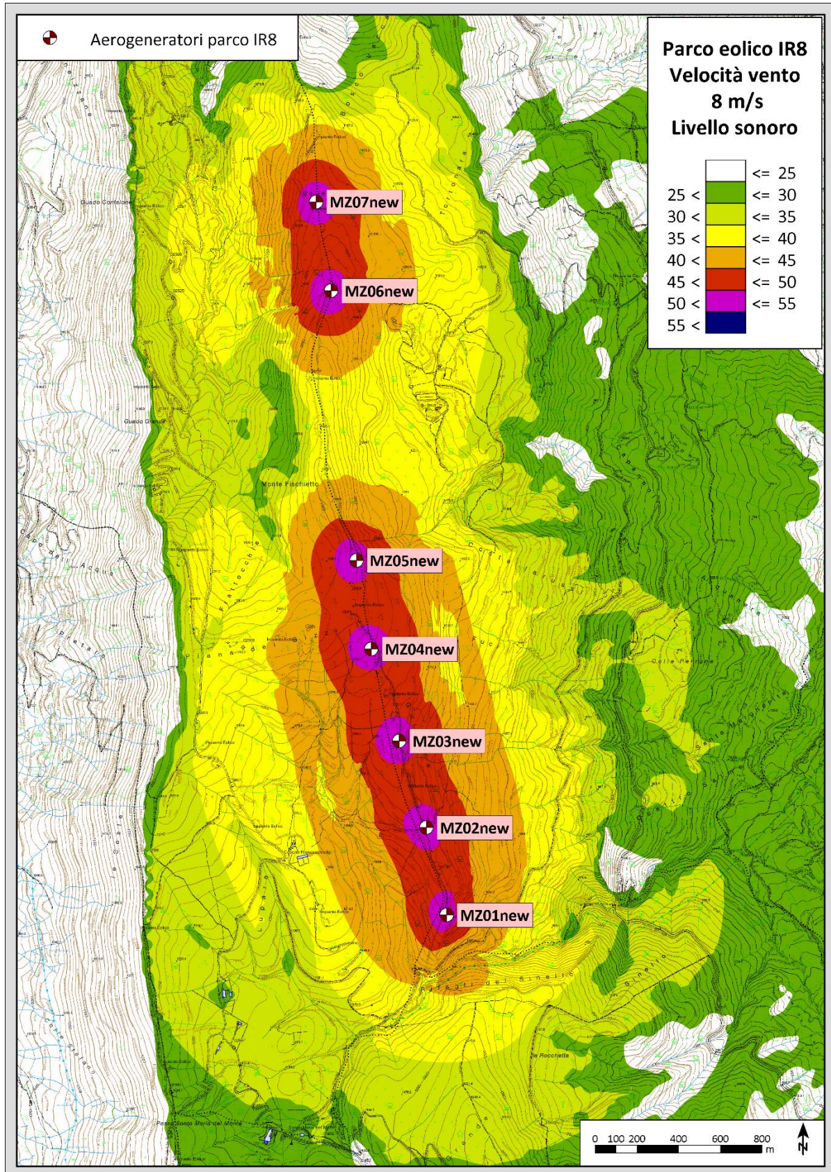
Figura 14- Parco eolico di Montazzoli IR8: curve isofoniche di immissione specifica degli aerogeneratori con V_{hub} = 8 m/s.
