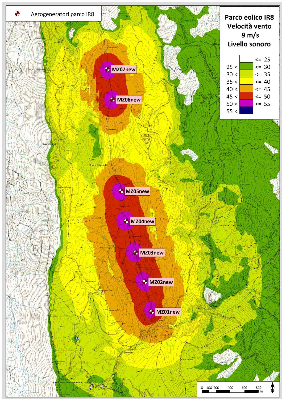
Figura 15- Parco eolico di Montazzoli IR8: curve isofoniche di immissione specifica degli aerogeneratori con V_{hub} = 9 m/s– Massimo livello emissivo.
