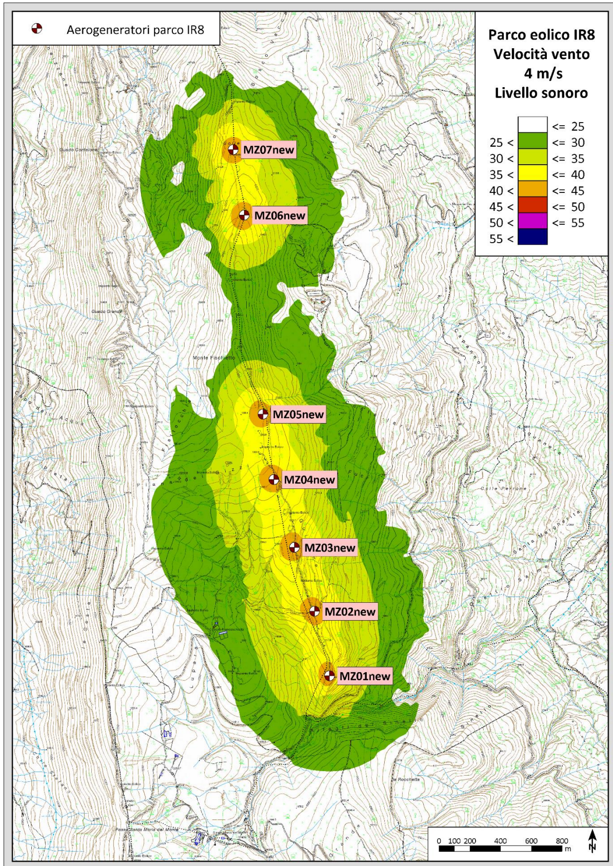
Figura 12- Parco eolico di Montazzoli IR8: curve isofoniche di immissione specifica degli aerogeneratori con V_{hub} = 4 m/s.
