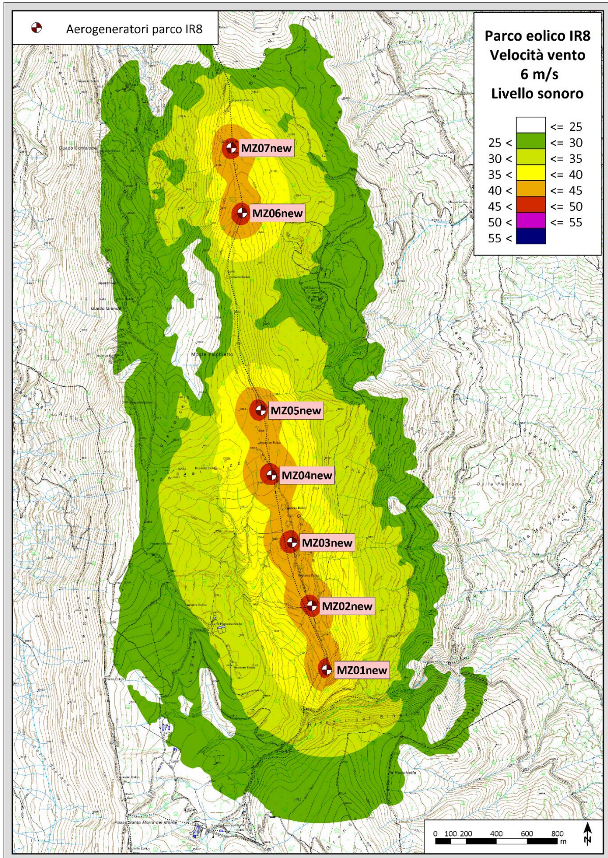
Figura 13- Parco eolico di Montazzoli IR8: curve isofoniche di immissione specifica degli aerogeneratori con V_{hub} = 6 m/s.
