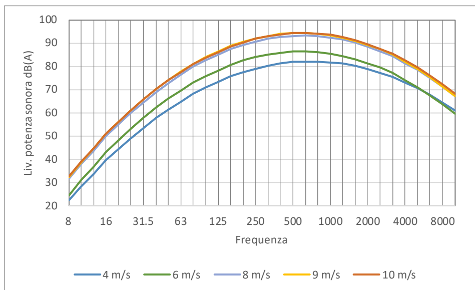
Figura 10 - Parco eolico di Montazzoli - Spettro di potenza sonora ponderato ‘A’ degli aerogeneratori modellati per V_{hub} = 4, 6, 8, 9, 10 m/s.
