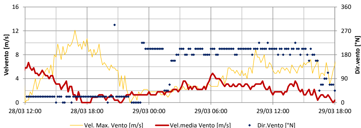
Figura 18 – Parco eolico di Montazzoli: andamento dei principali parametri meteo nell’arco del periodo di fuori servizio del parco stesso per la misura del rumore residuo presso il punto P4.
