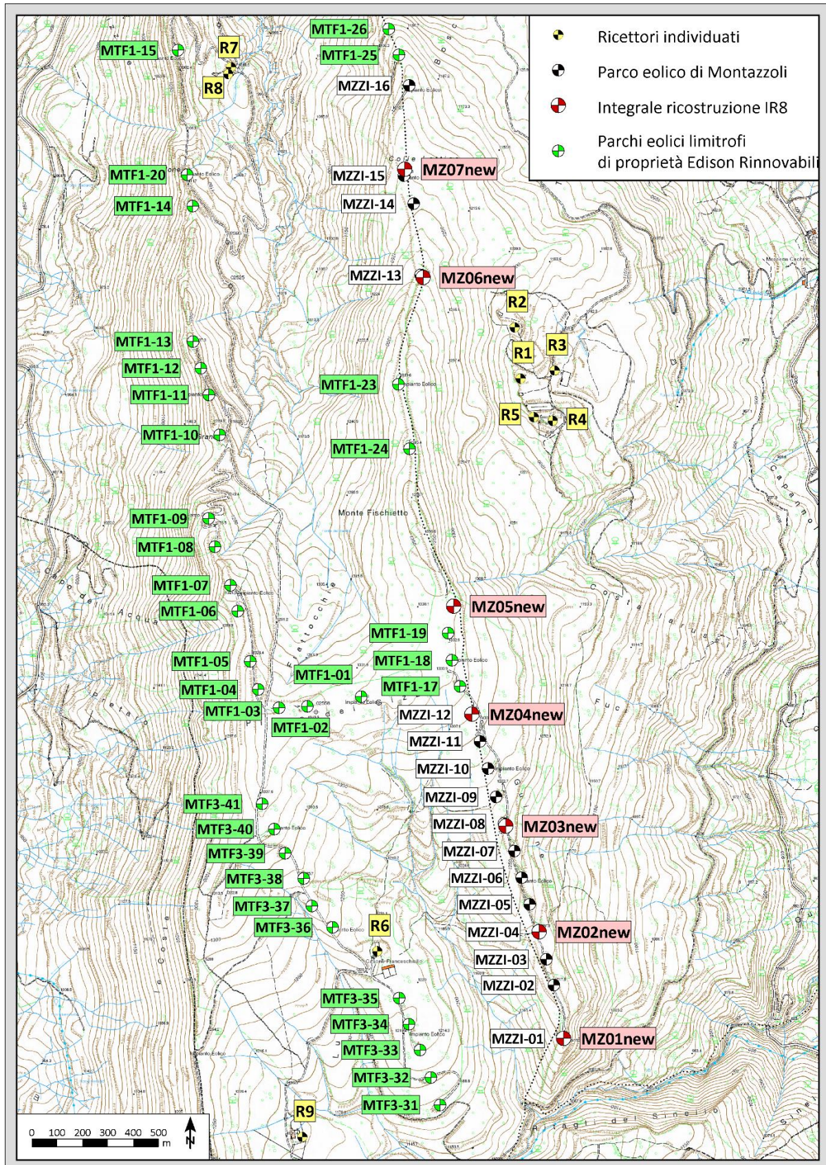
Figura 2 – Parco eolico di Montazzoli - Ubicazione degli aerogeneratori esistenti e in progetto (MZ01new ÷ MZ07new) e dei ricettori individuati nell’ambito del censimento.
