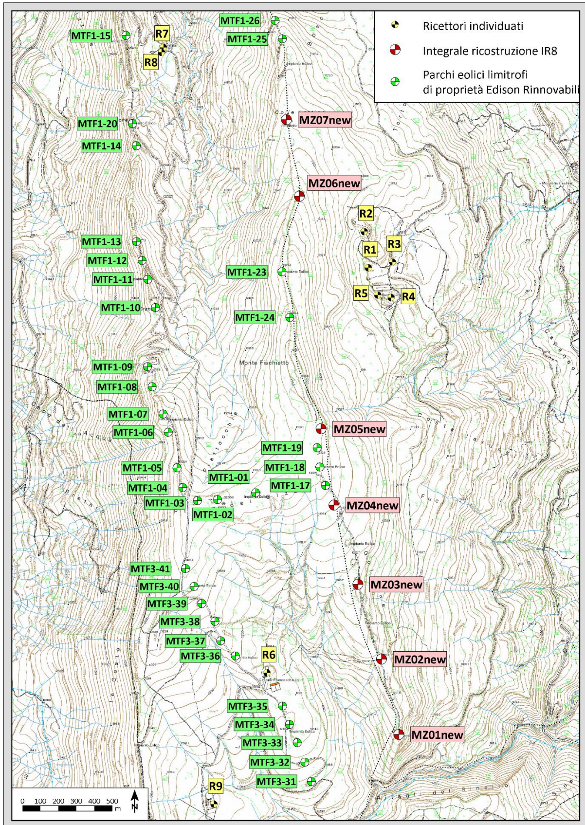
Figura 9 – Parco eolico di Montazzoli - Ubicazione degli aerogeneratori in progetto (MZ01new ÷ MZ07new) e dei punti di calcolo presso ricettori introdotti nella modellazione.
