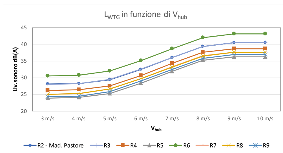
Figura 11- Parco eolico di Montazzoli (IR8) - Livelli di immissione specifica calcolati ai ricettori in funzione di V hub .
