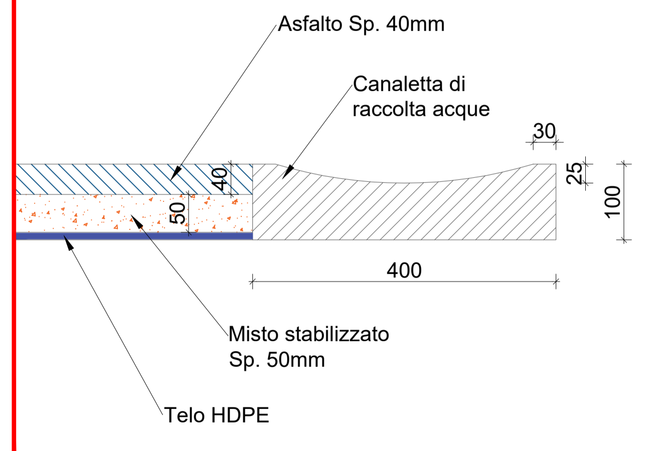
Particolare A - Scala 1:5
