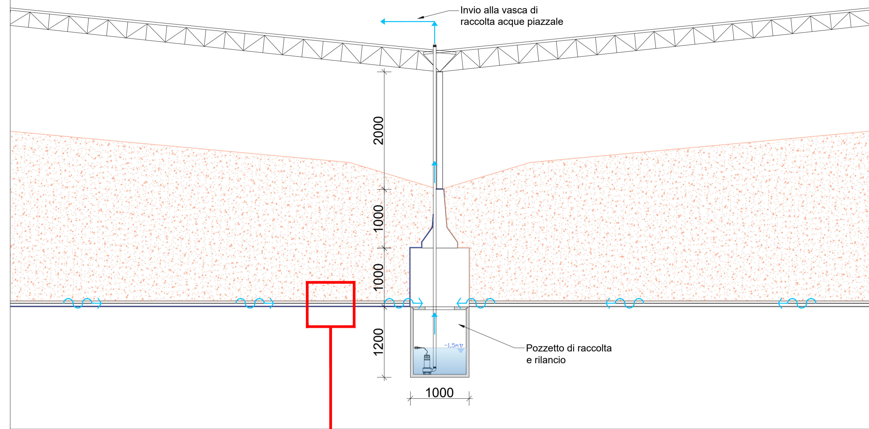
Sezione 3 - Scala 1:50
