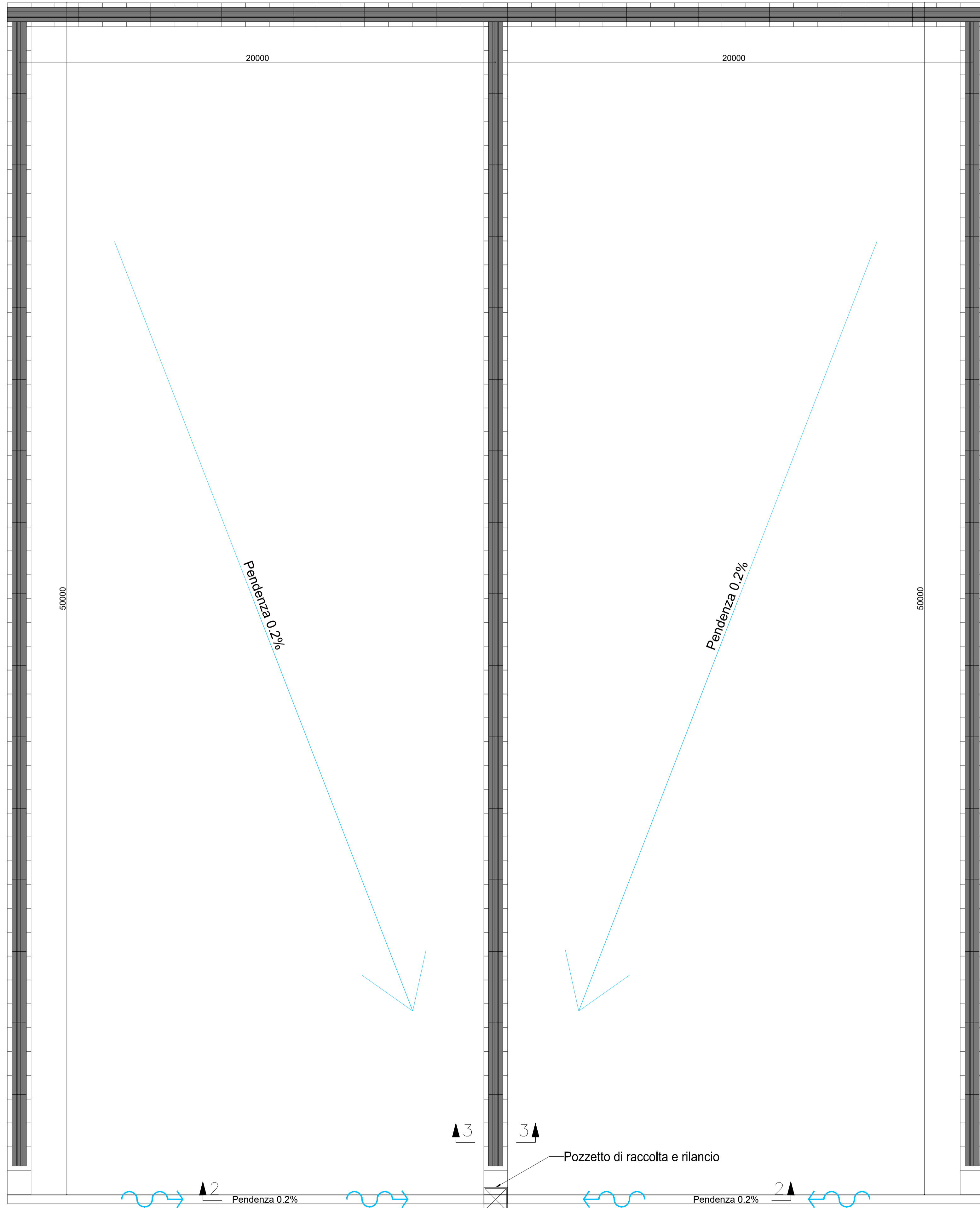
Planimetria - Scala 1:100
