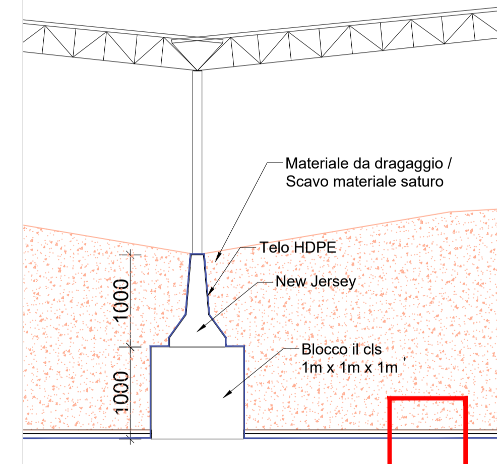
Sezione 3 - Scala 1:50
