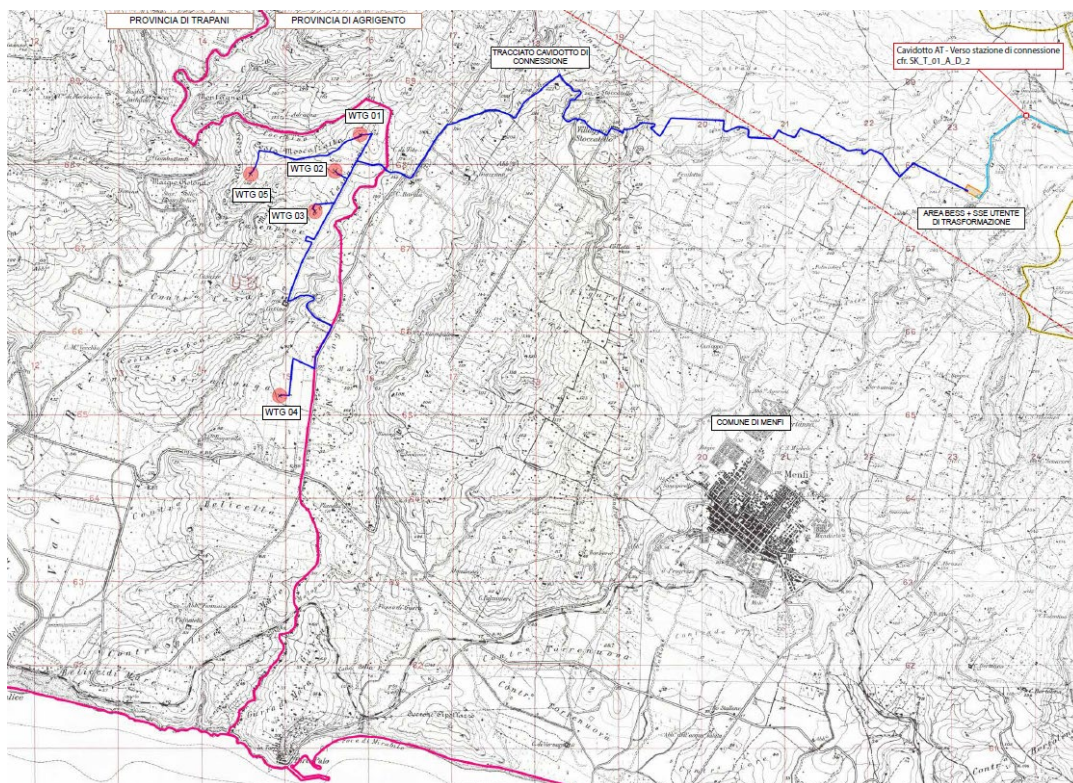
Figura 1 Inquadramento su IGM del parco eolico e della Stazione di trasformazione 30/36 kV
