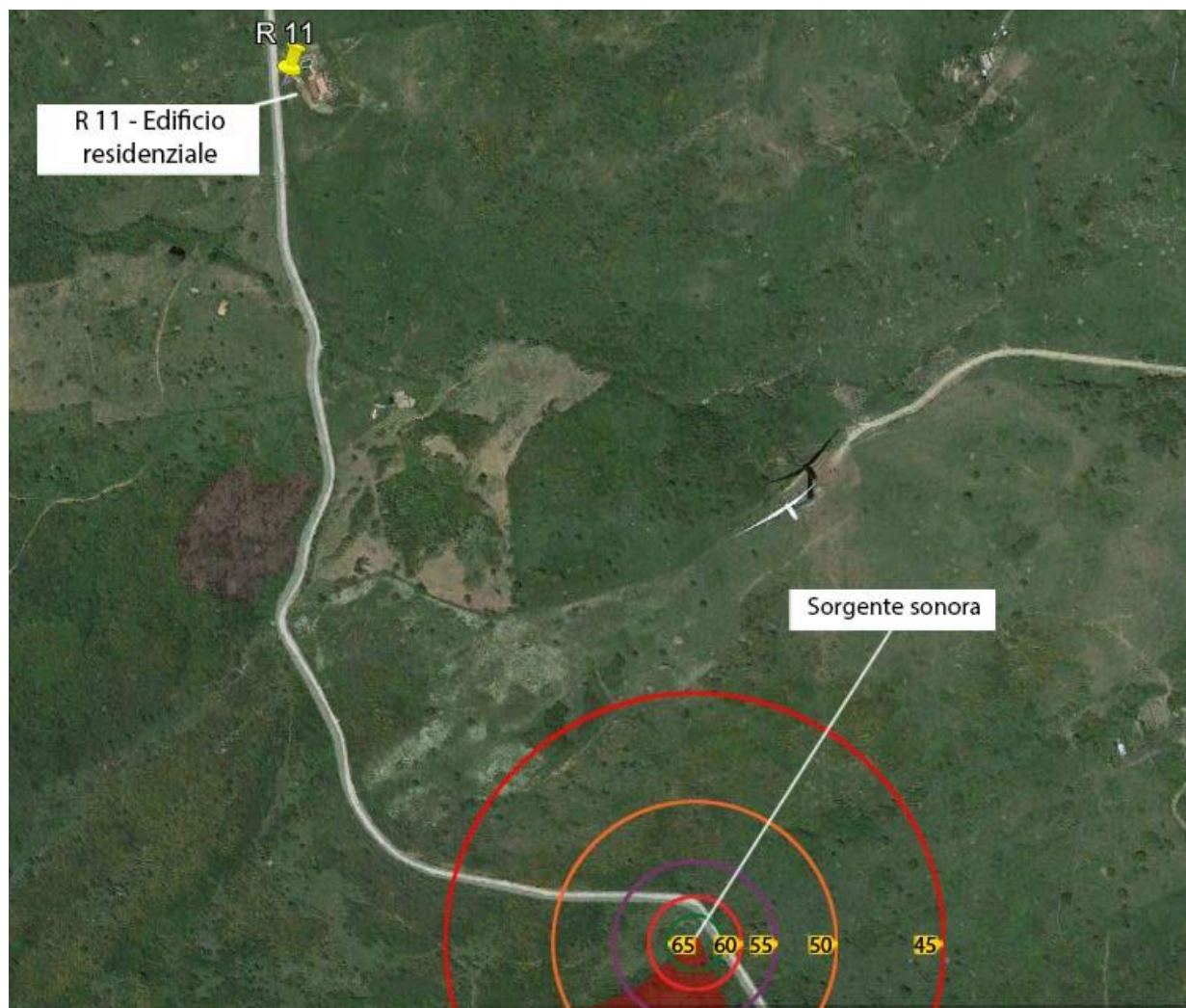
Figura 5: Emissioni sonore in fase di cantiere, mappa dei livelli di pressione sonora [dB(A)]
