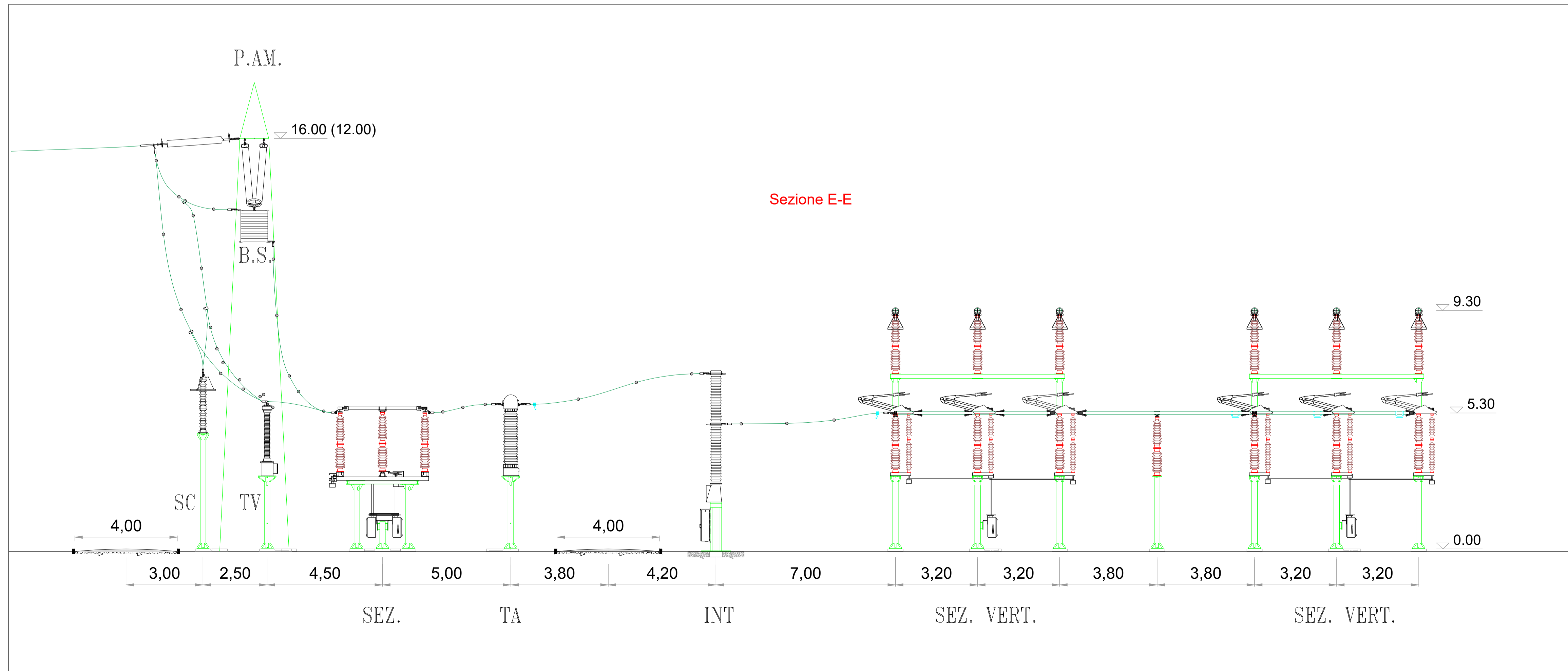
Sezione E-E - Scala 1:100
