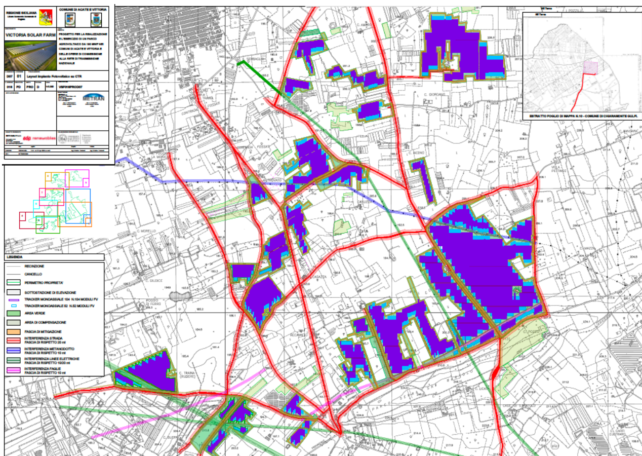
Figura 10 -Layout impianto su CTR
