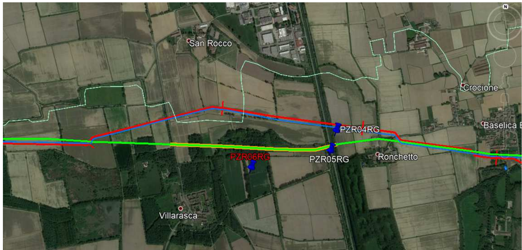
Figura 4.2- Posizione dei piezometri nel tratto di non rimozione della ZSC/ZPS IT2080023 "Garzaia Cascina Villarasca"
