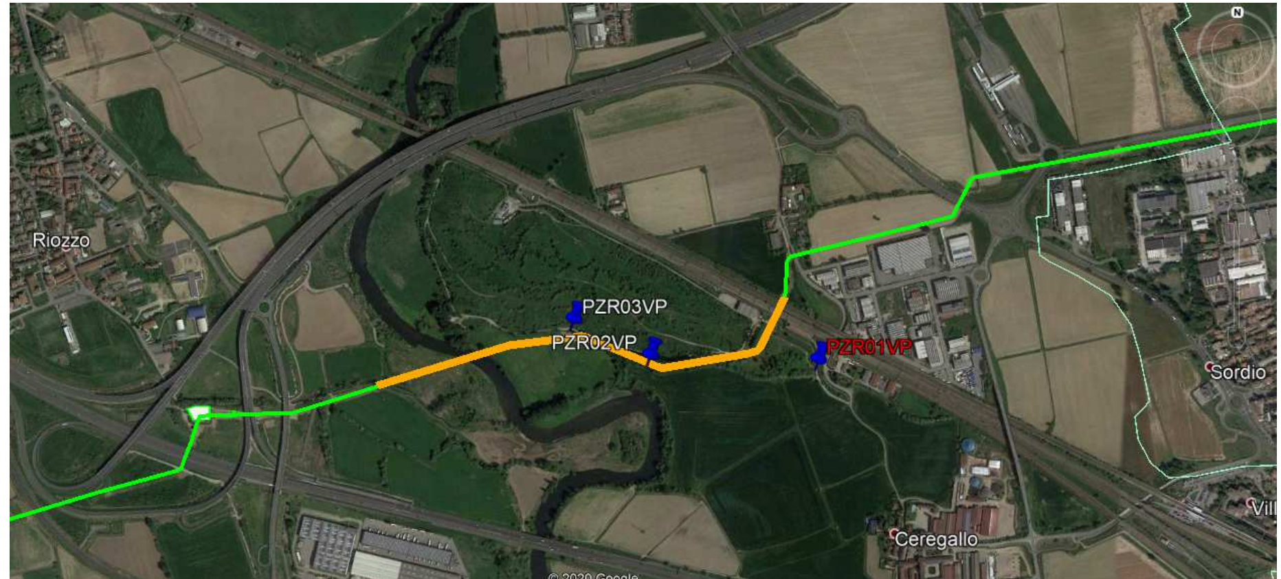
Figura 4.1- Posizione dei piezometri nel tratto di non rimozione della Ex-discarica di Vizzolo - Fiume Lambro
