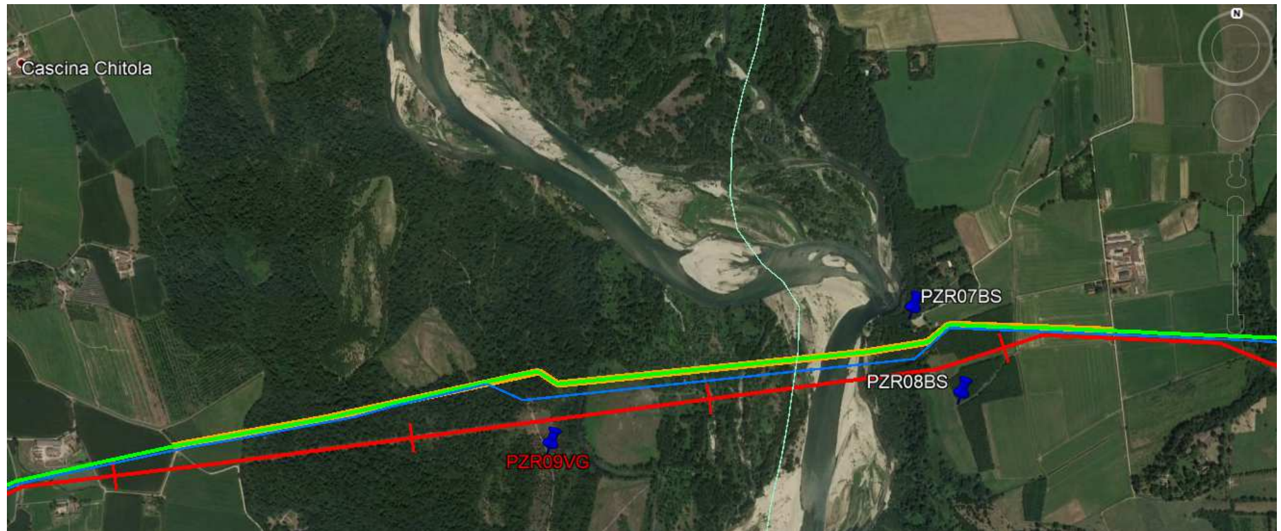
Figura 4.3- Posizione dei piezometri nel tratto di non rimozione del Fiume Ticino e Bosco del Modrone
