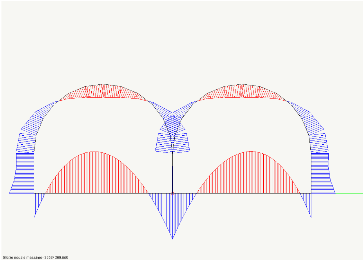
DIAGRAMMA DEL MOMENTIO FLETTENTE CONDIZIONE DI CARICO 1
