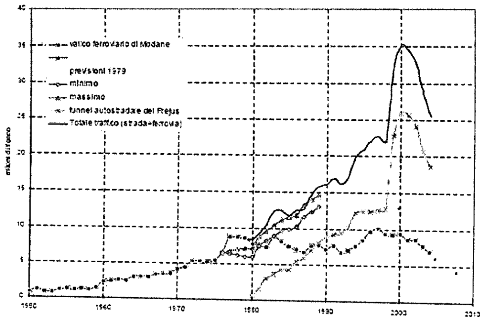
Tunnel ferroviario ed autostradale del Fréjus andamento storico del traffico (1950-2004)
