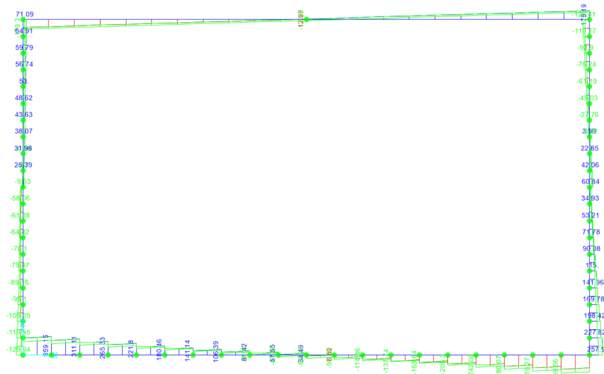
Involuppo SLV sforzo di taglio
