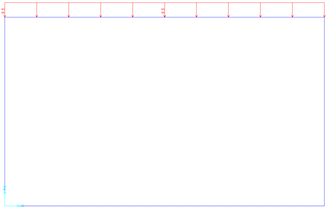
Figura 10.2 - condizione di carico g2 – peso rinterro
