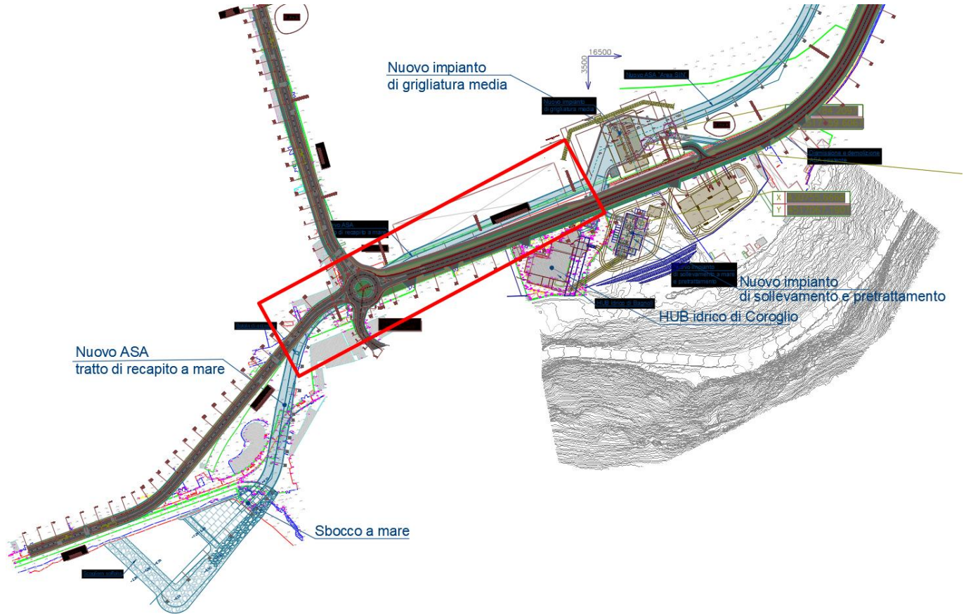
Fig. 1: Planimetria generale e inquadramento dell' opera
