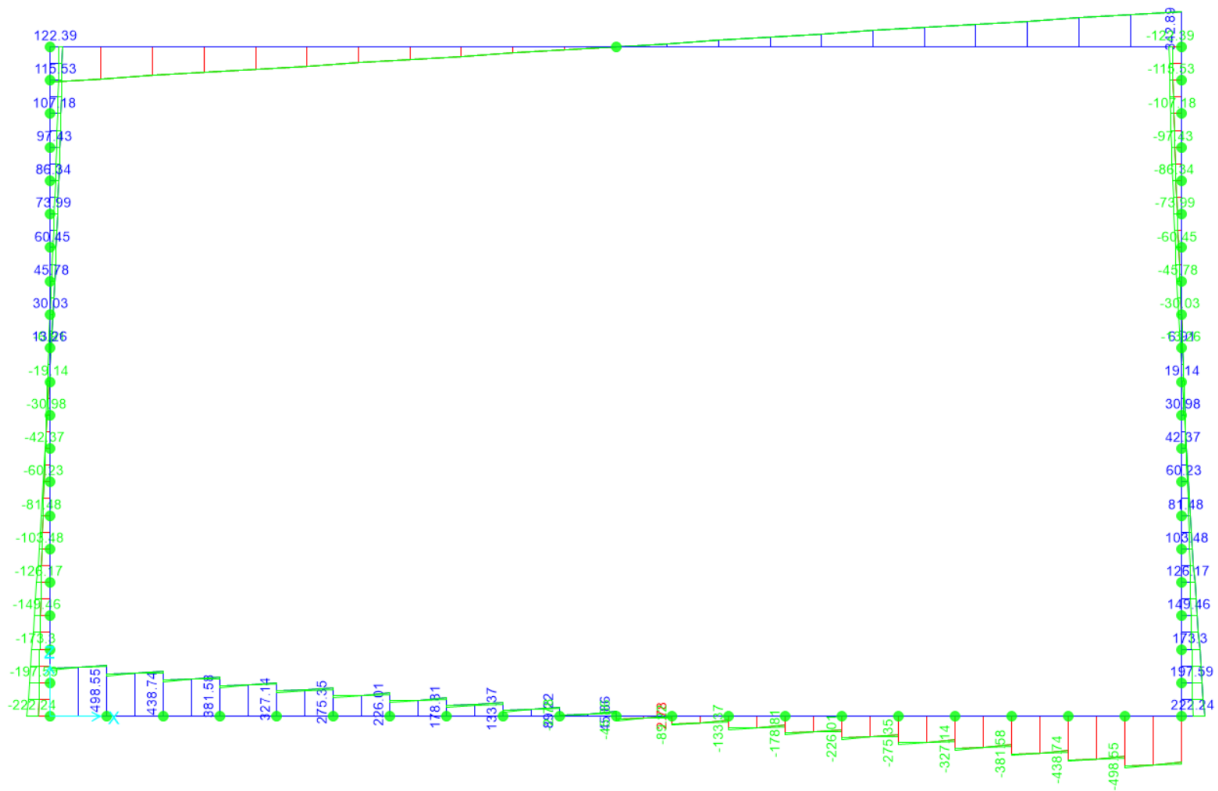
Figura 10.14 – Inviluppo SLU sforzo di taglio
