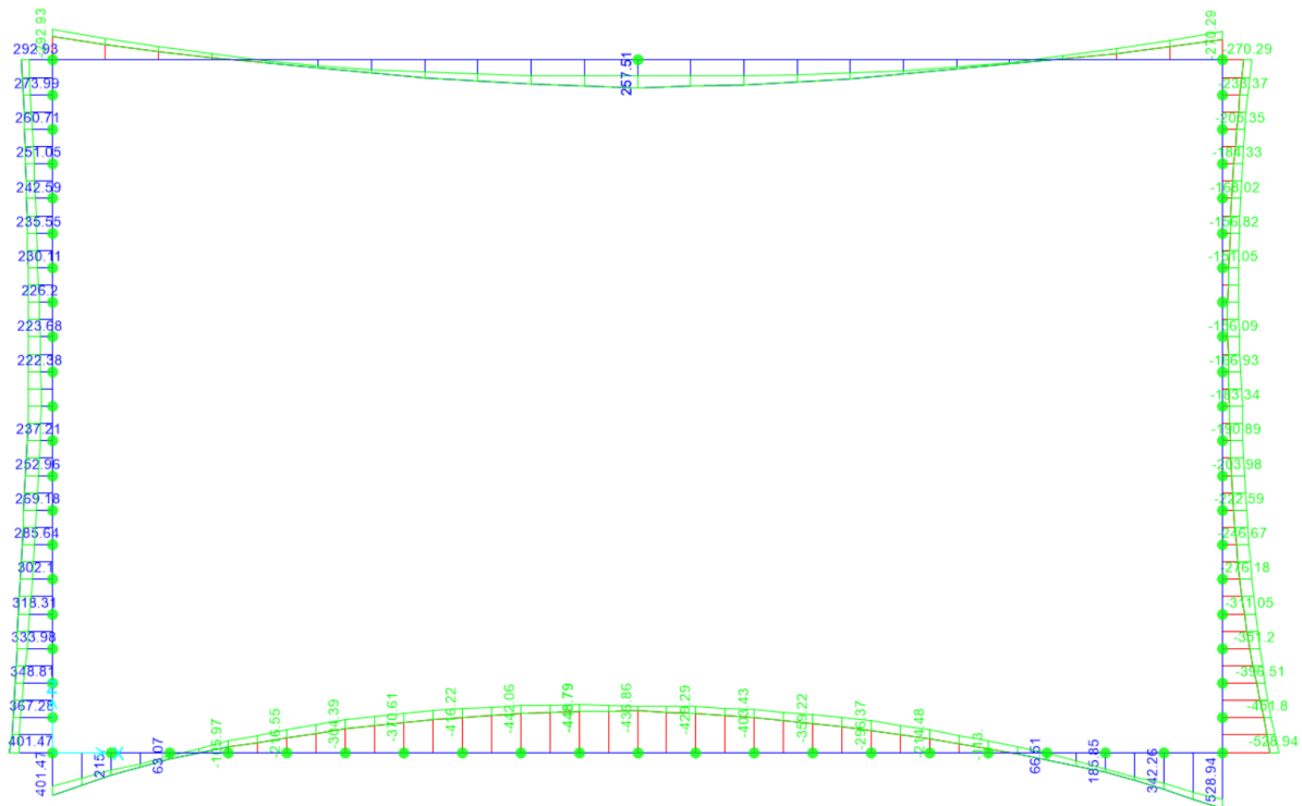
Fig. 11 - Inviluppo SLV momento flettente
