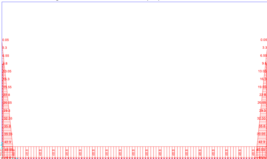
Figura 10.6 - condizione di carico u – spinta statica dell'acqua vasca sinistra
