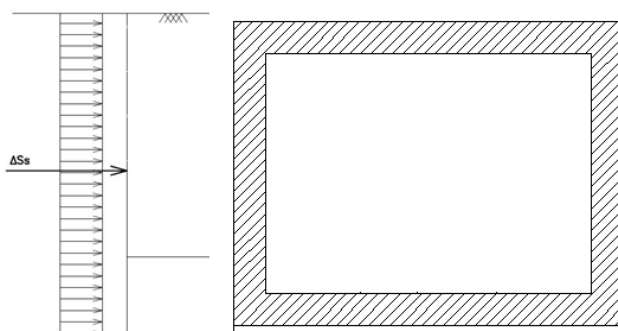
Figura 10.1 – Schema per il calcolo degli effetti della sovrappinta sismica del terreno
