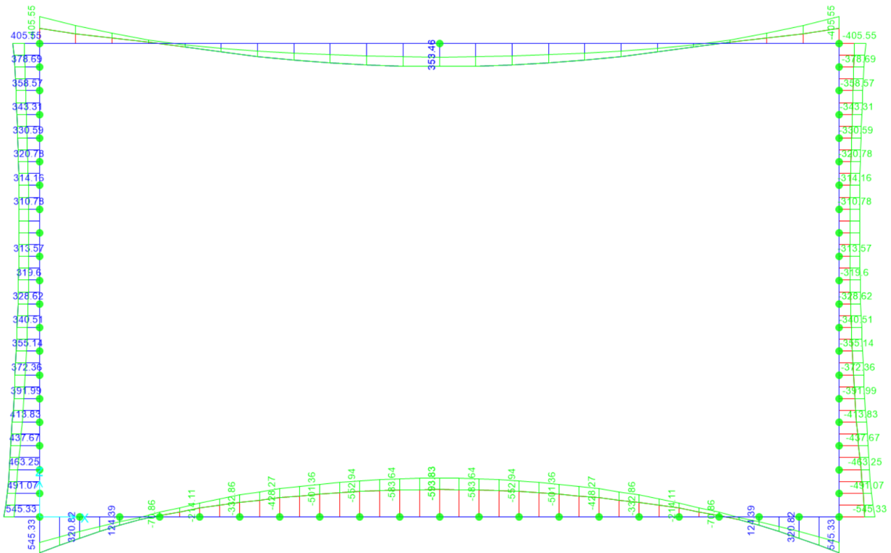
ra 10.12 – Inviluppo SLE momento flettente
