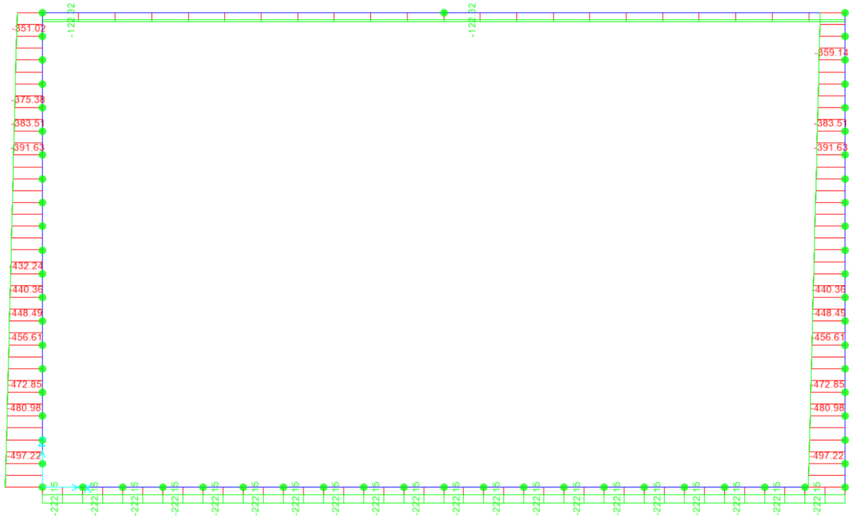
Figura 10.13 – Involuppo SLU sforzo normale
