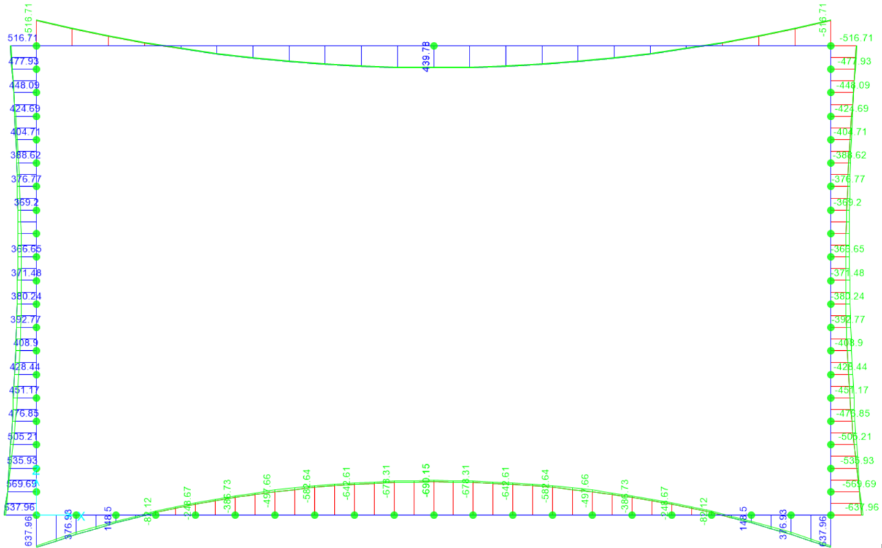
10.15 – Inviluppo SLU momento flettente
