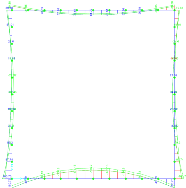
Figura 10.14 – Involupto SLU momento flettente
