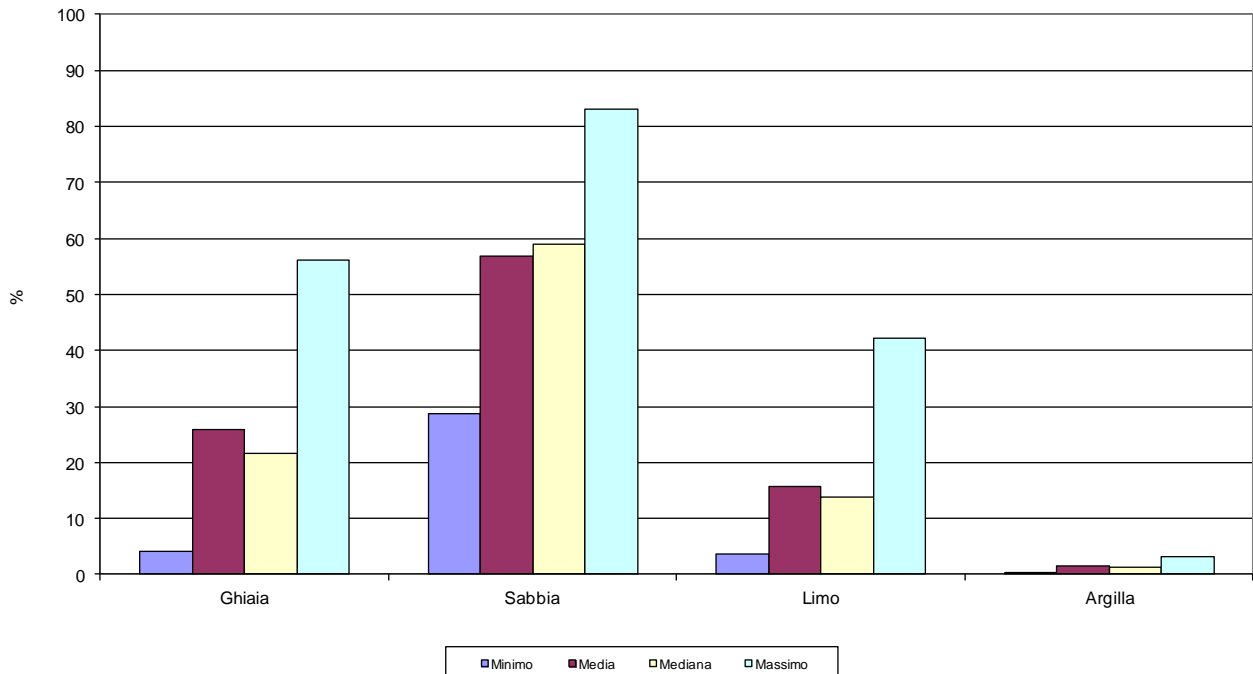
Figura 5.7 - Frazioni granulometriche nelle sabbie ghiaiose
