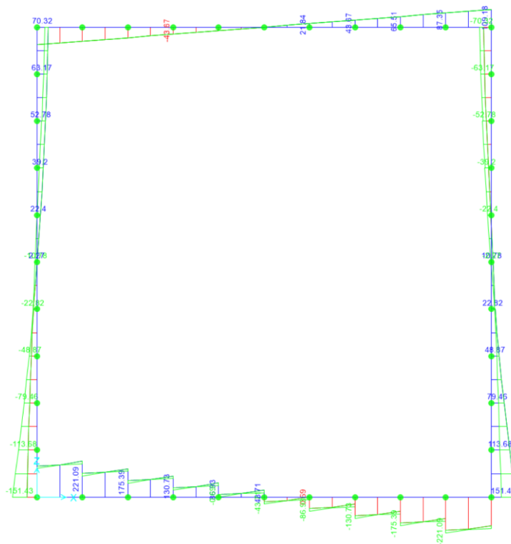
Figura 10.13 – Involuppo SLU sforzo di taglio
