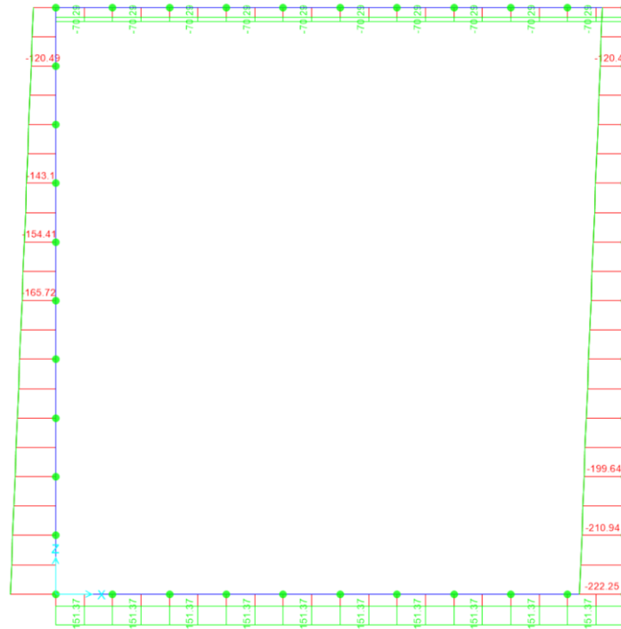
Figura 10.12 – Involuppo SLU sforzo normale
