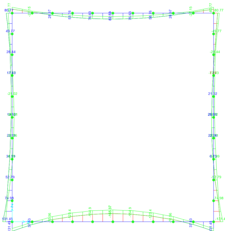
Figura 10.11 – Inviluppo SLE momento flettente
