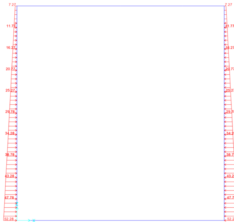
Figura 10.4 - condizione di carico g_1 – spinta del terreno
