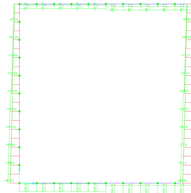
Fig. 9 - Involupto SLV sforzo normale
