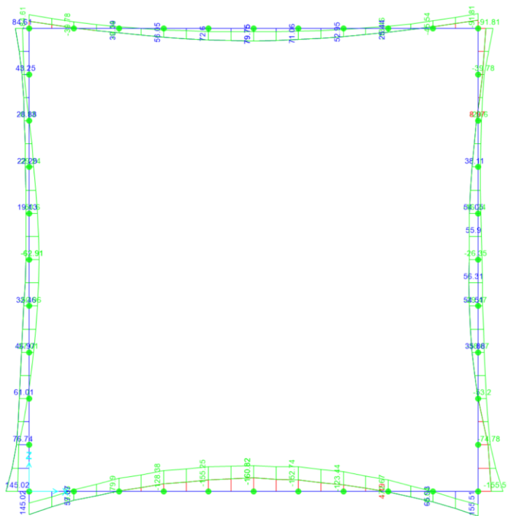
Fig. 11 - Involuppo SLV momento flettente
