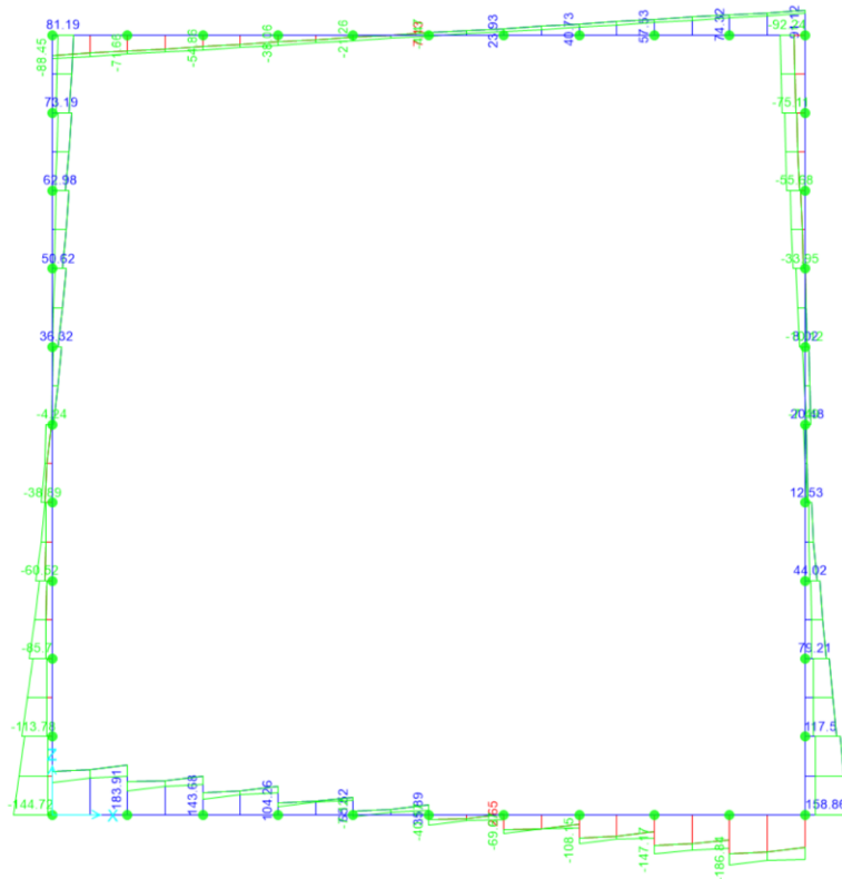
Fig. 10 - Involuppo SLV sforzo di taglio
