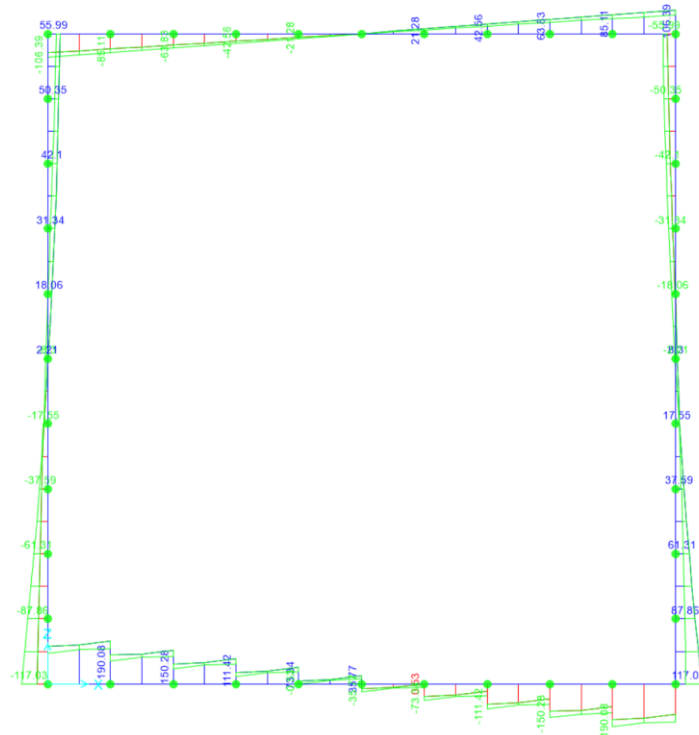
Figura 10.10 – Inviluppo SLE sforzo di taglio
