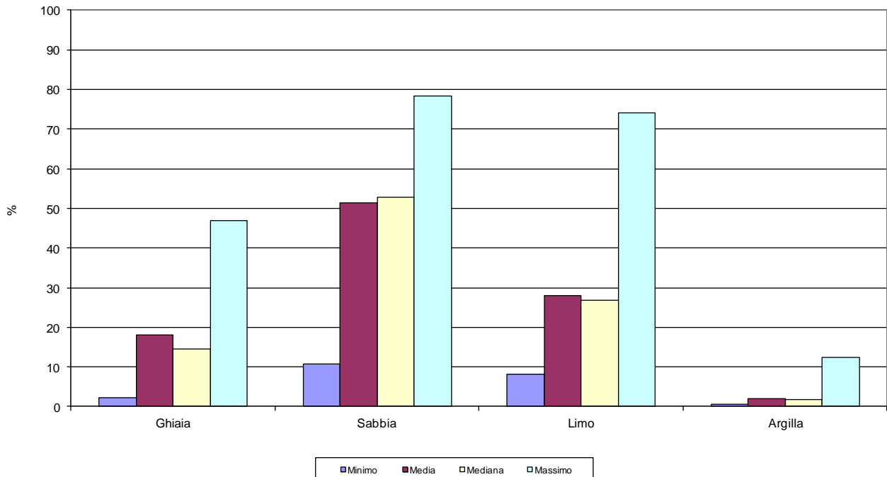
Figura 5.8 - Frazioni granulometriche nelle piroclastici
