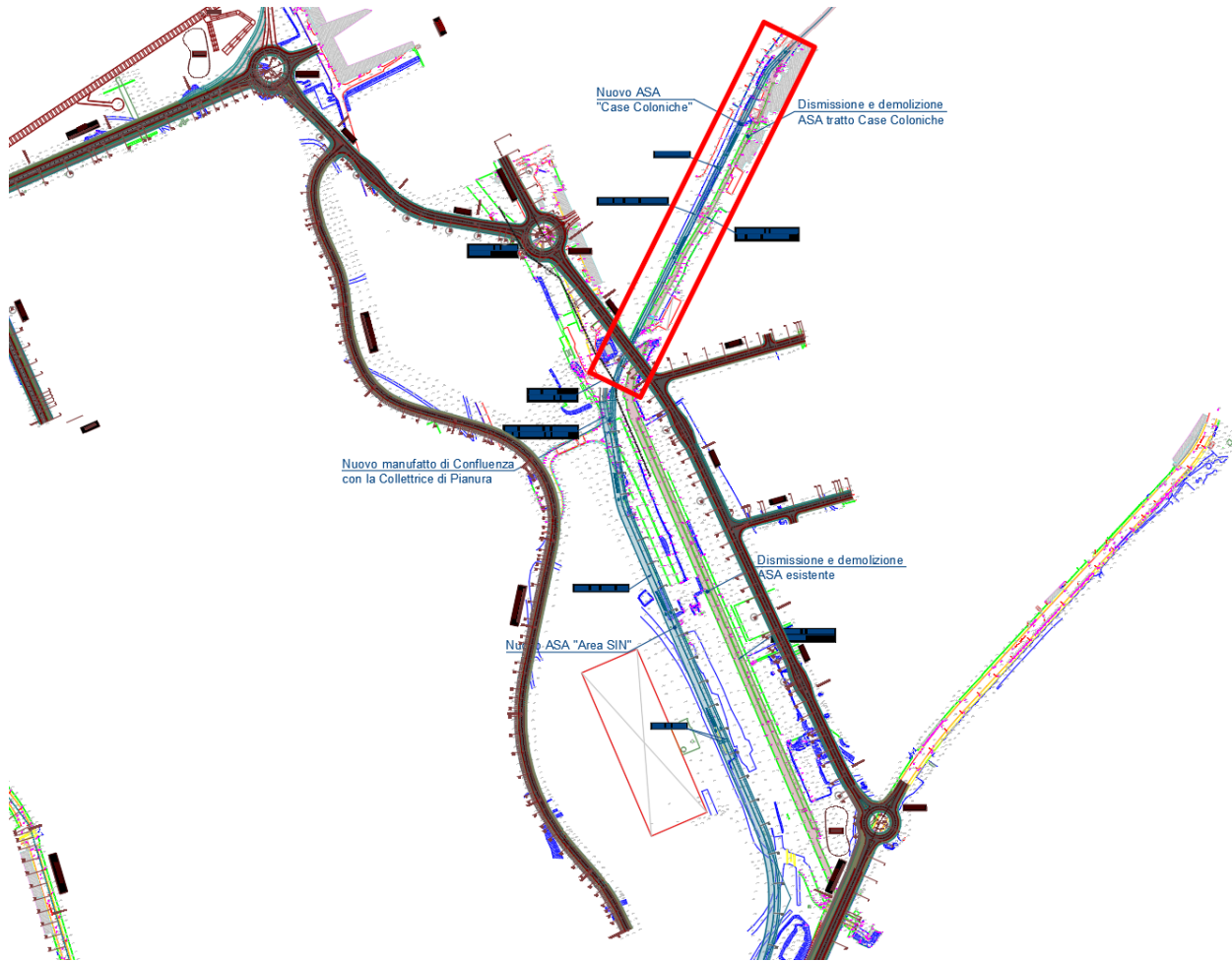
Fig. 1: Planimetria generale e inquadramento dell' opera
