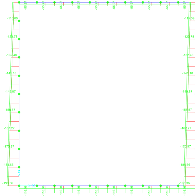
Figura 10.9 – Inviluppo SLE sforzo normale
