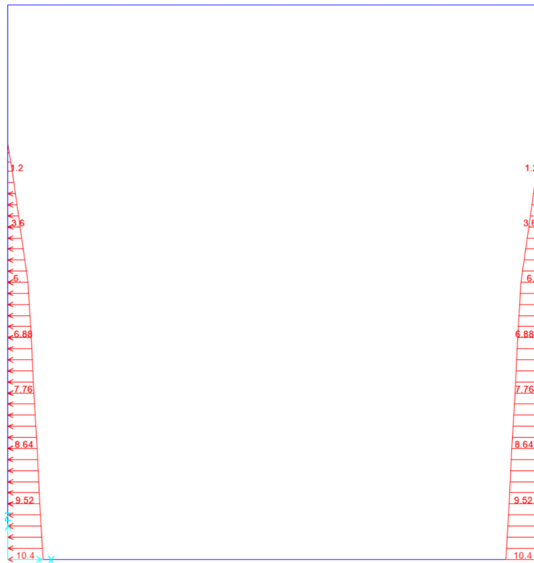
Figura 10.6 - condizione di carico u_{din} – spinta idrodinamica dell'acqua nella vasca
