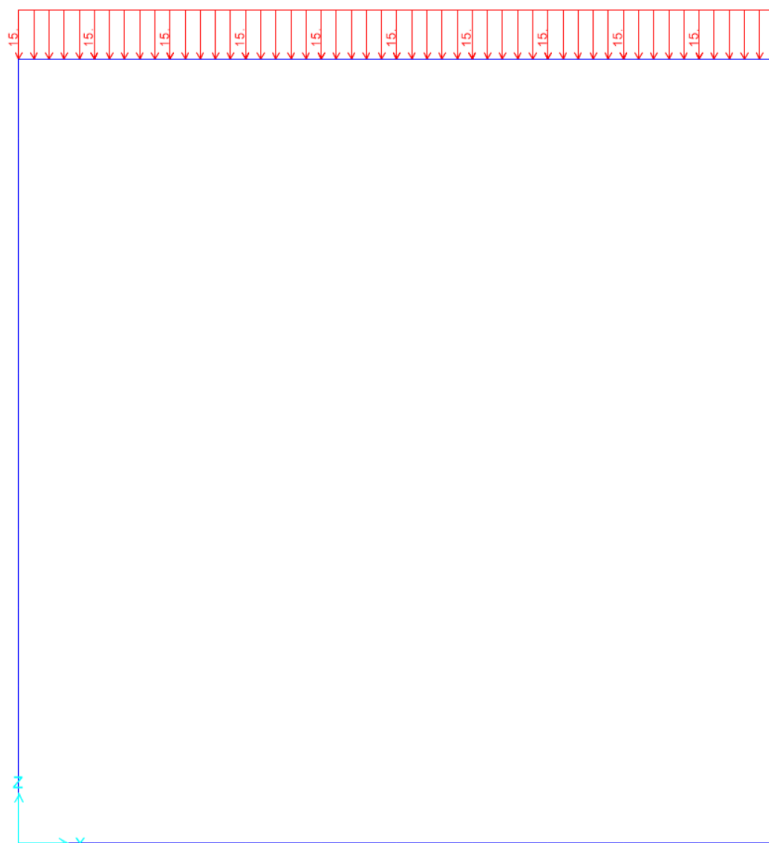
Figura 10.2 - condizione di carico g2 – peso rinterro
