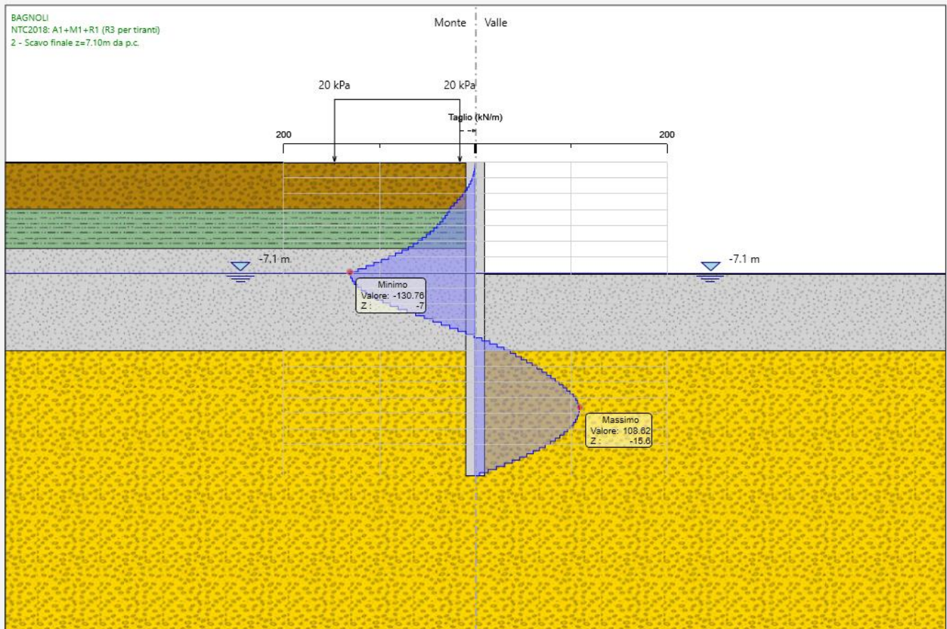
Figura 8: Taglio - SLU.
