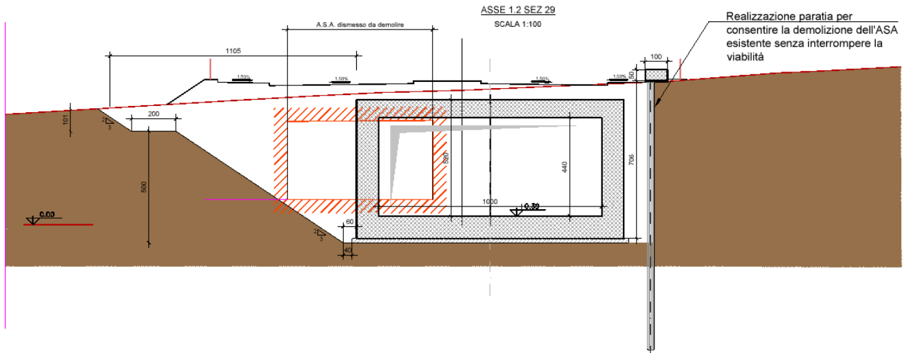
Figura 2: Paratia 1 bis – Prolungamento.
