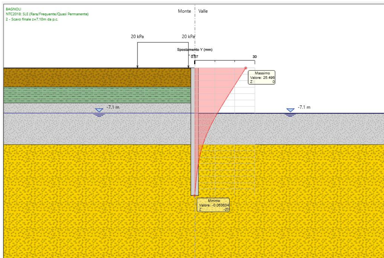
Figura 10: Spostamenti orizzontali allo SLE.
