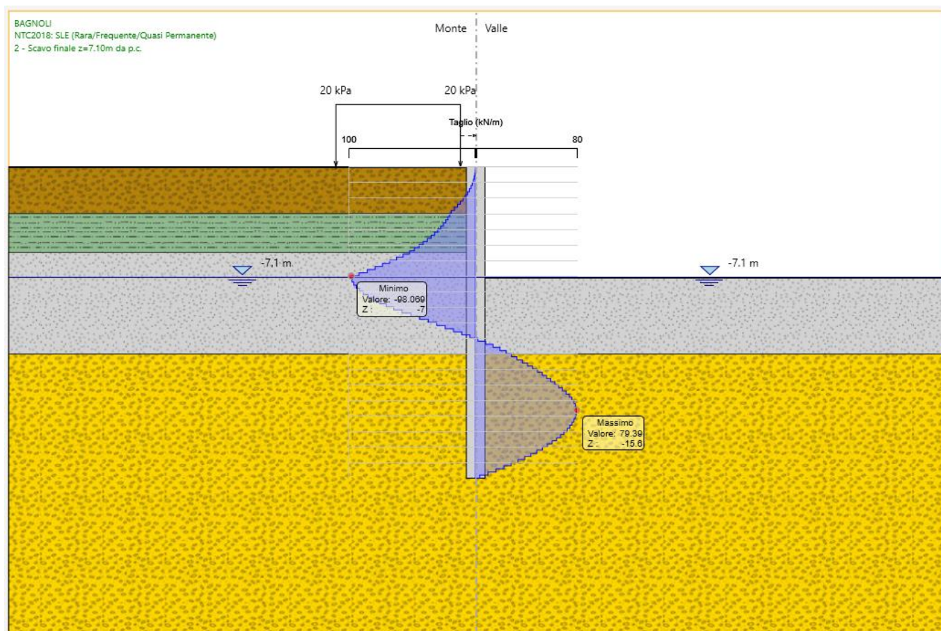
Figura 9: Taglio - SLE.
