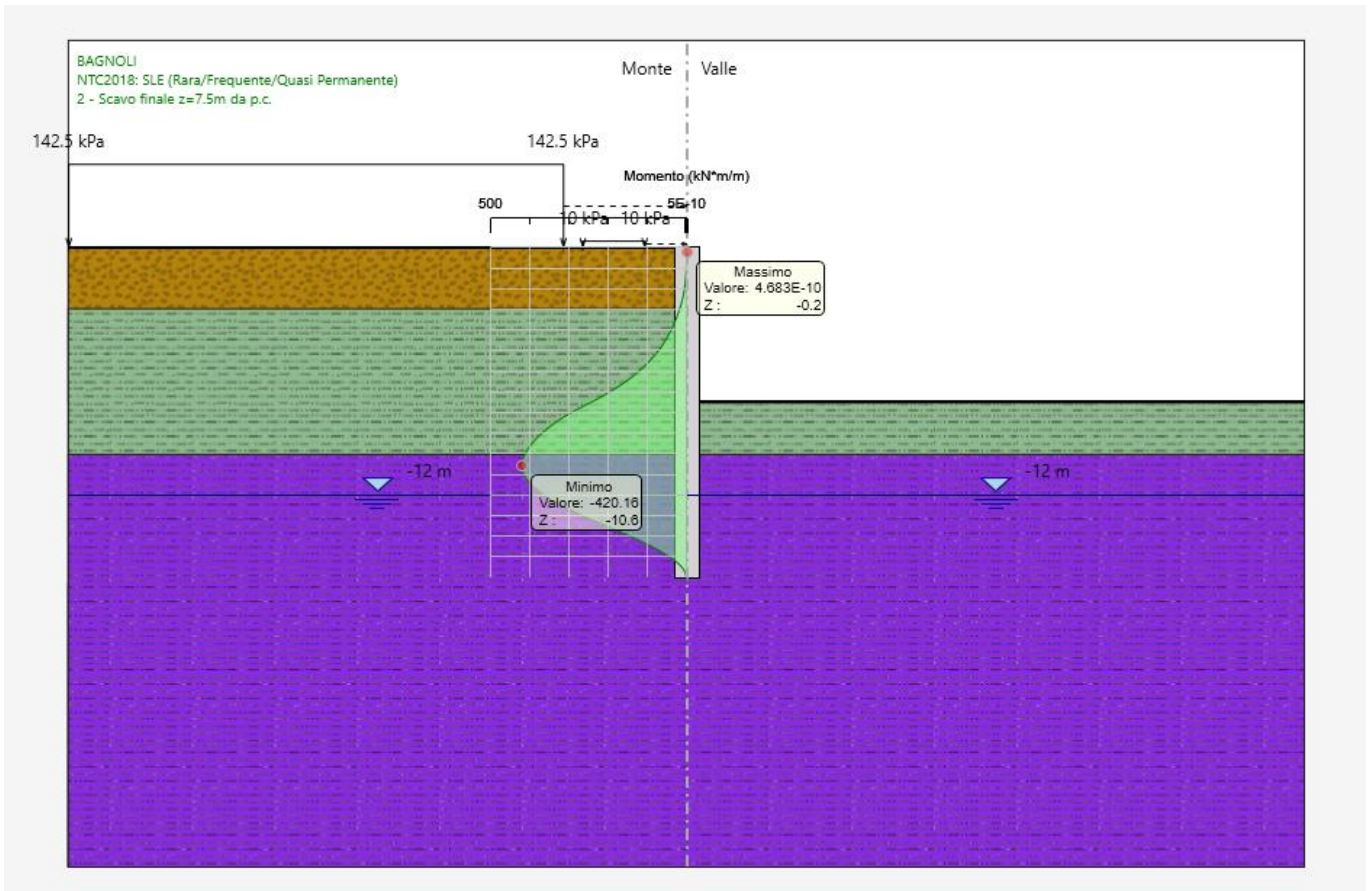
Figura 6: Momento flettente - SLE.
