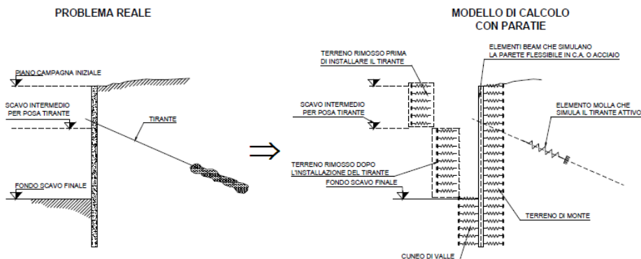
Figura 3: Schematizzazione terreno ed ancoraggi.
