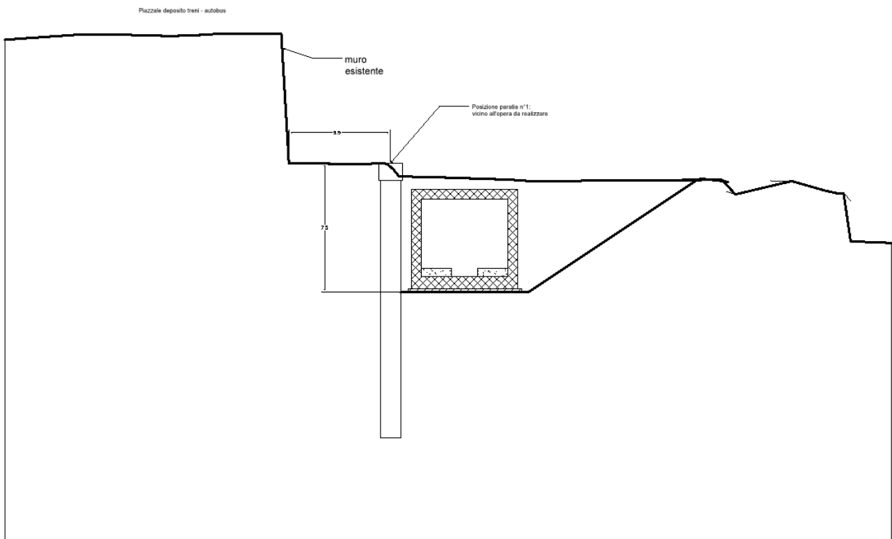
Figura 4: Sezione di calcolo.
