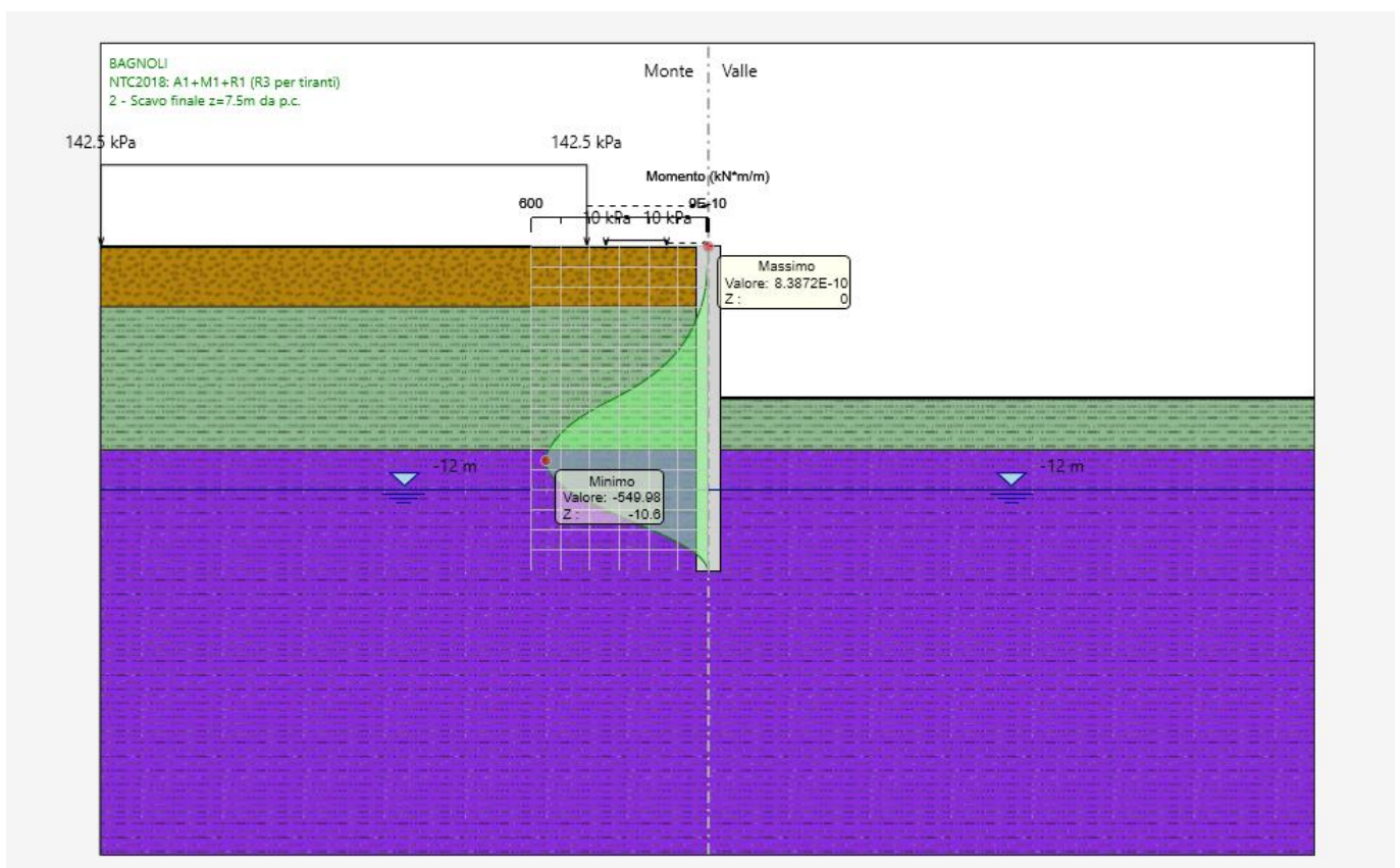
Figura 5: Momento flettente - SLU.
