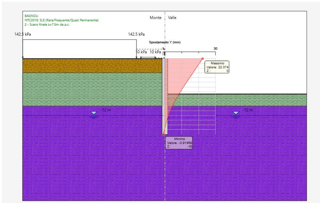
Figura 9: Spostamenti orizzontali allo SLE.
