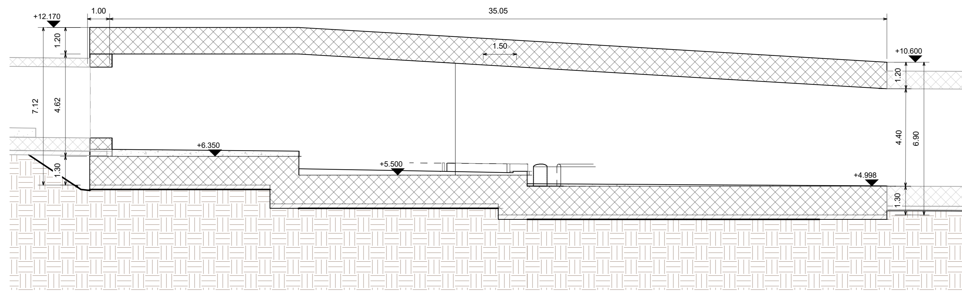
05 Sezione 05 Scala 1 : 100
