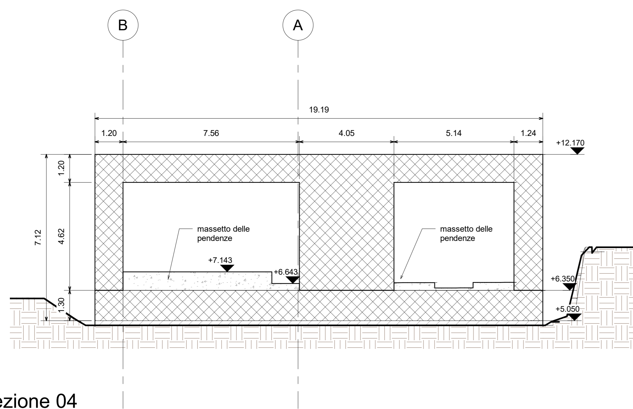
04 Sezione 04 Scala 1 : 100
