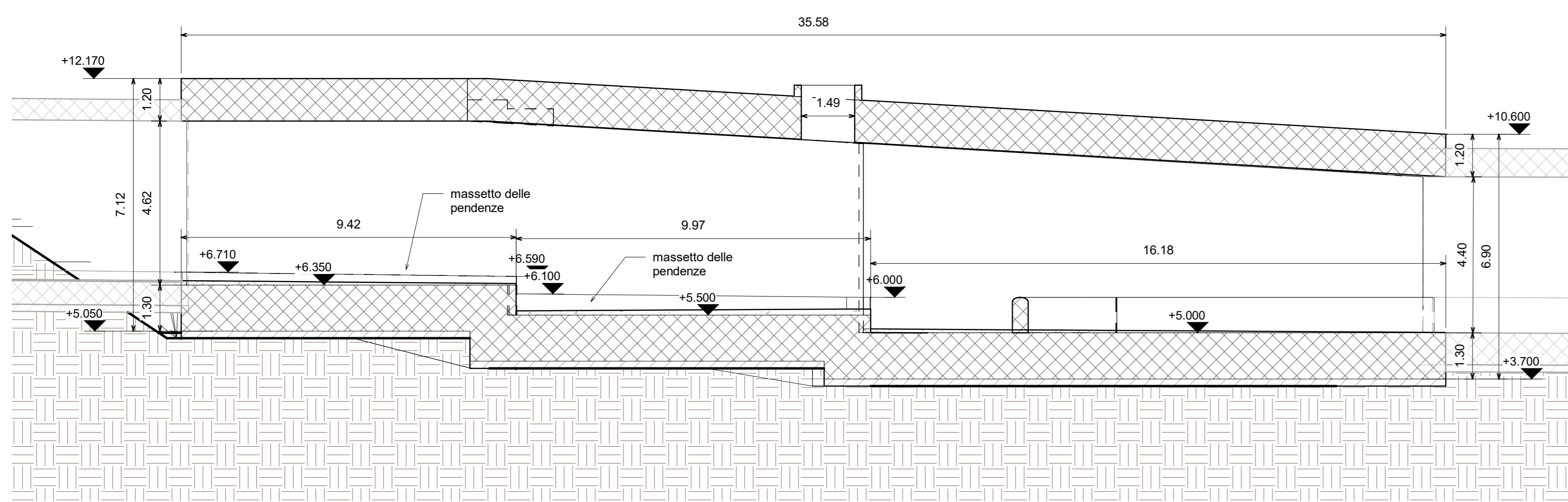
06 Sezione 06 Scala 1 : 100
