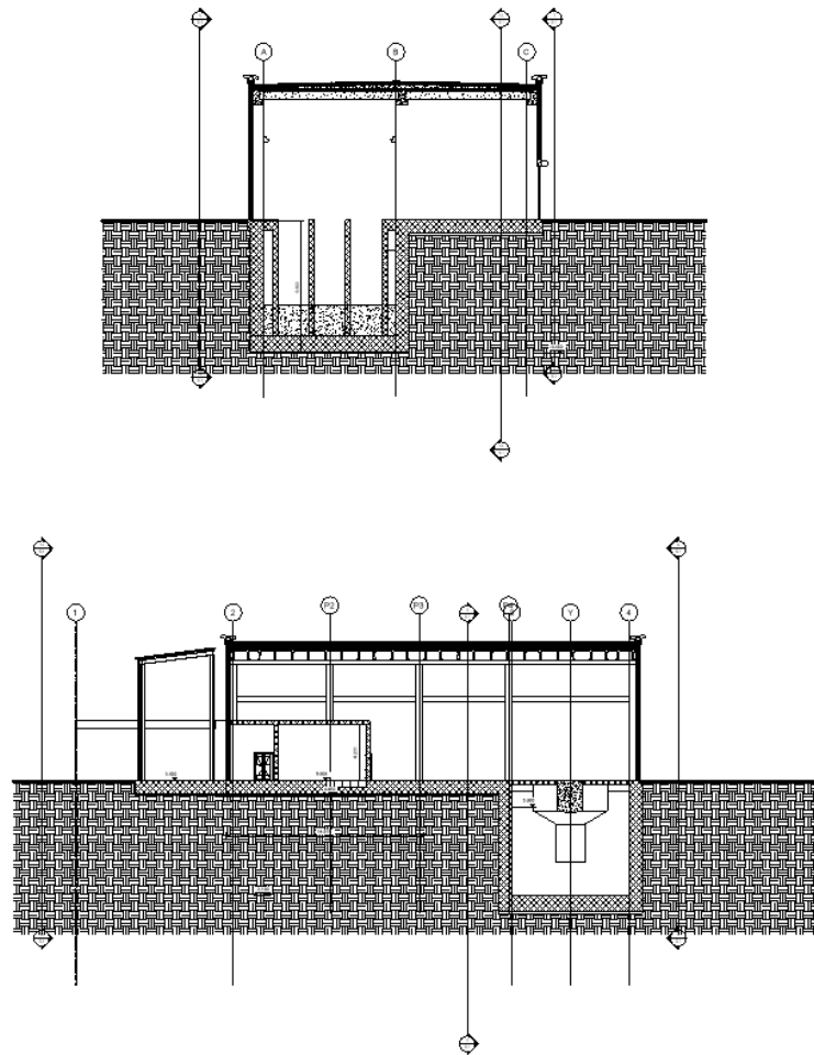
Figura 3: Sezioni tipo.
