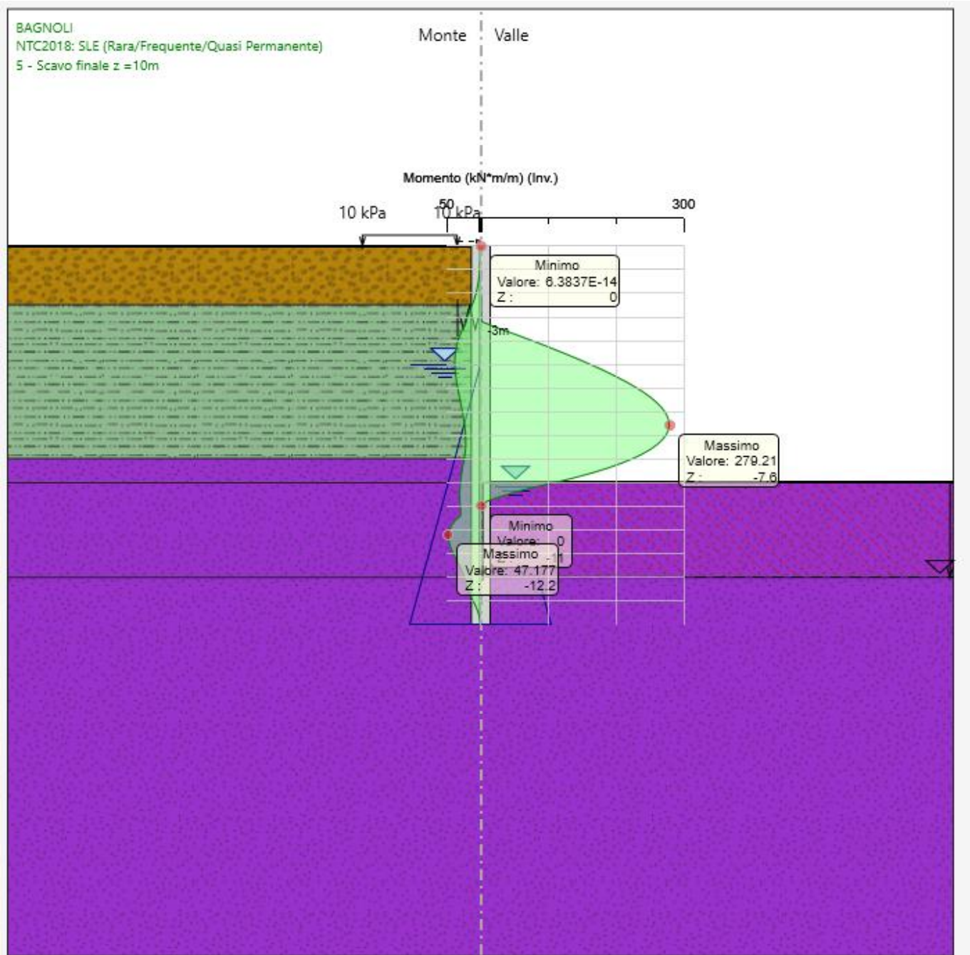
Figura 8: Inviluppo del Momento flettente - SLE.
