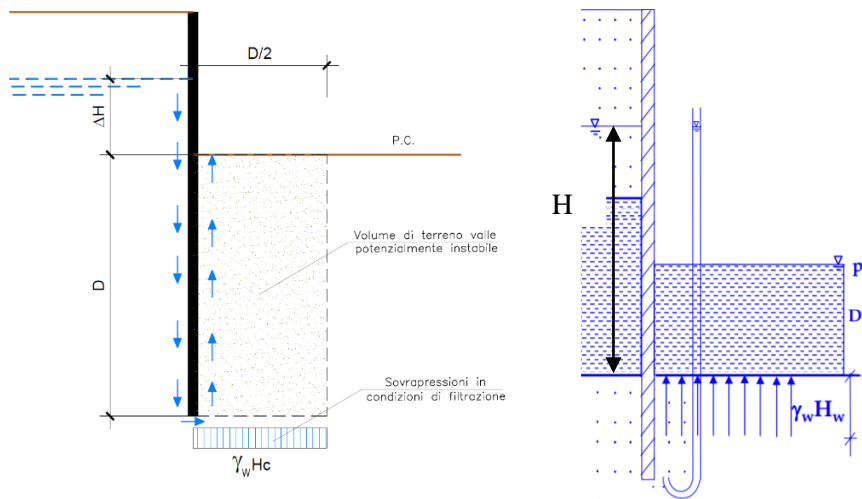
Figura 12: Schema di filtrazione per effetto di scavi sotto falda a valle di opere di sostegno.
