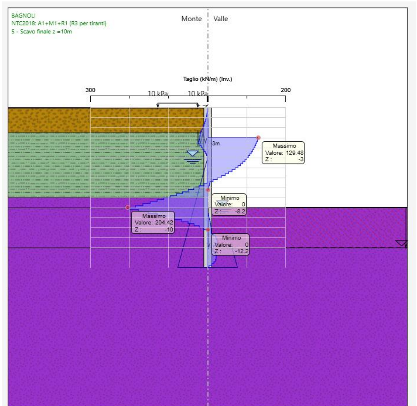
Figura 9: Involuppo del Taglio - SLU.
