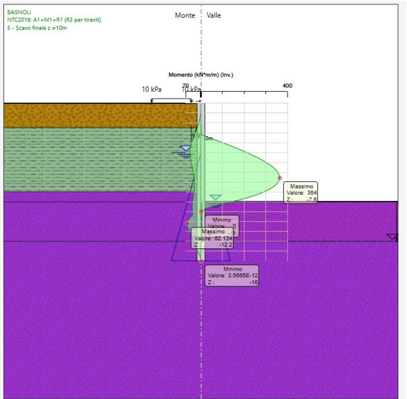
Figura 7: Inviluppo del Momento flettente - SLU.
