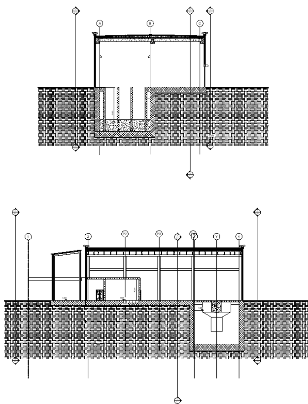
Figura 6: Sezione di calcolo.
