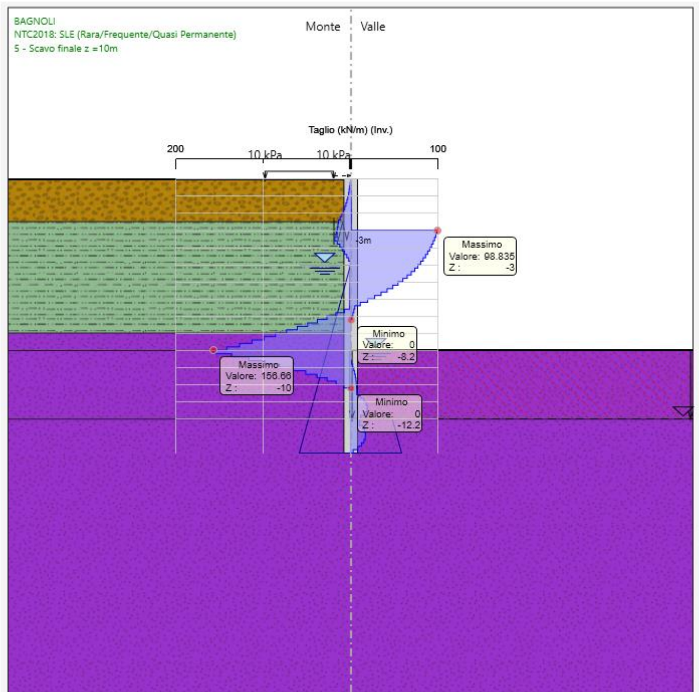
Figura 10: Inviluppo del Taglio - SLE.
