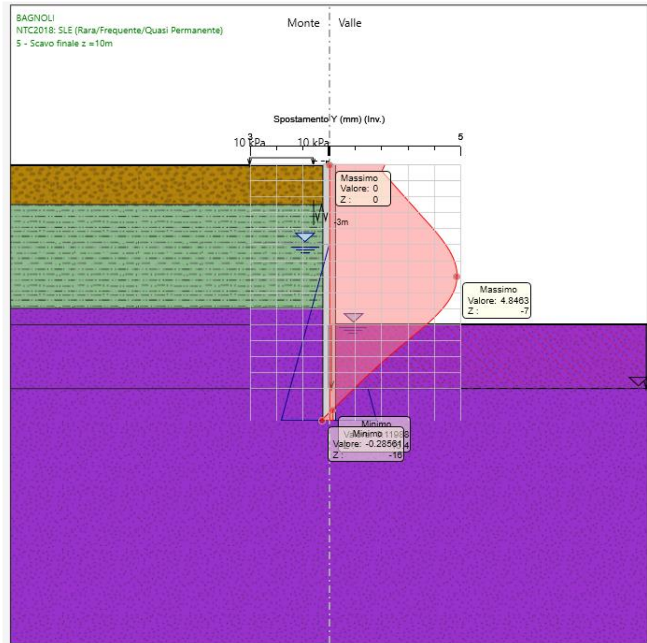
a 11: Involuppo degli spostamenti orizzontali allo SLE.
