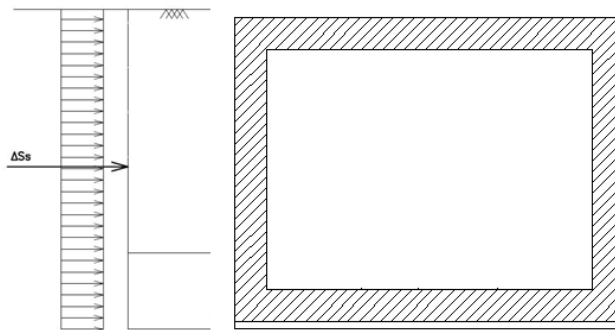
Fig. 8 – Schema per il calcolo degli effetti della sovrappinta sismica del terreno
