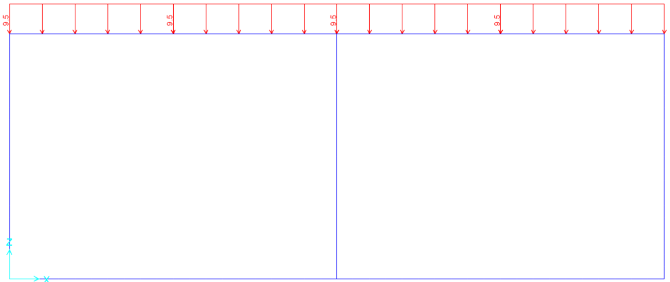
Figura 10.1 - condizione di carico g2 – peso rinterro
