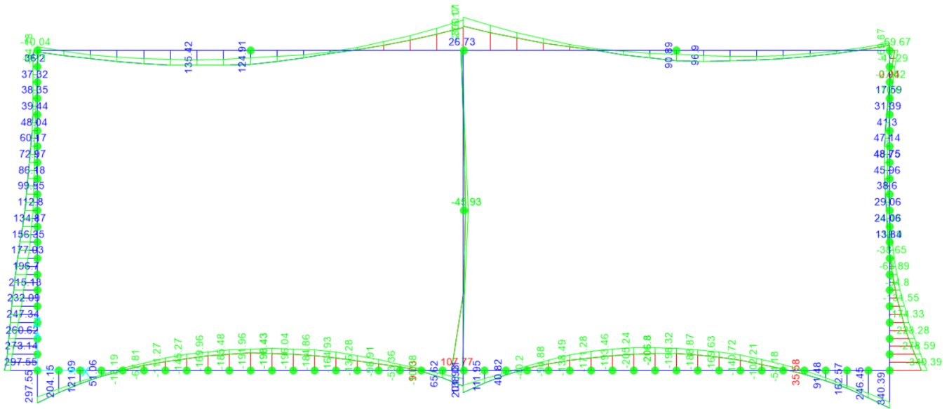
Figura 10.17 - Involuppo SLV momento flettente
