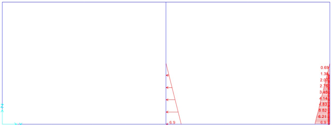
Figura 10.6 - condizione di carico u_{din} – spinta idrodinamica dell'acqua vasca sinistra
