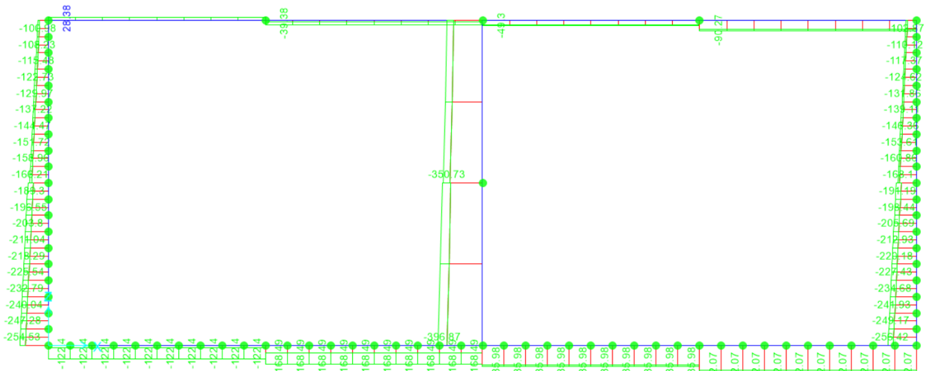
Figura 10.15 - Involuppo SLV sforzo normale
