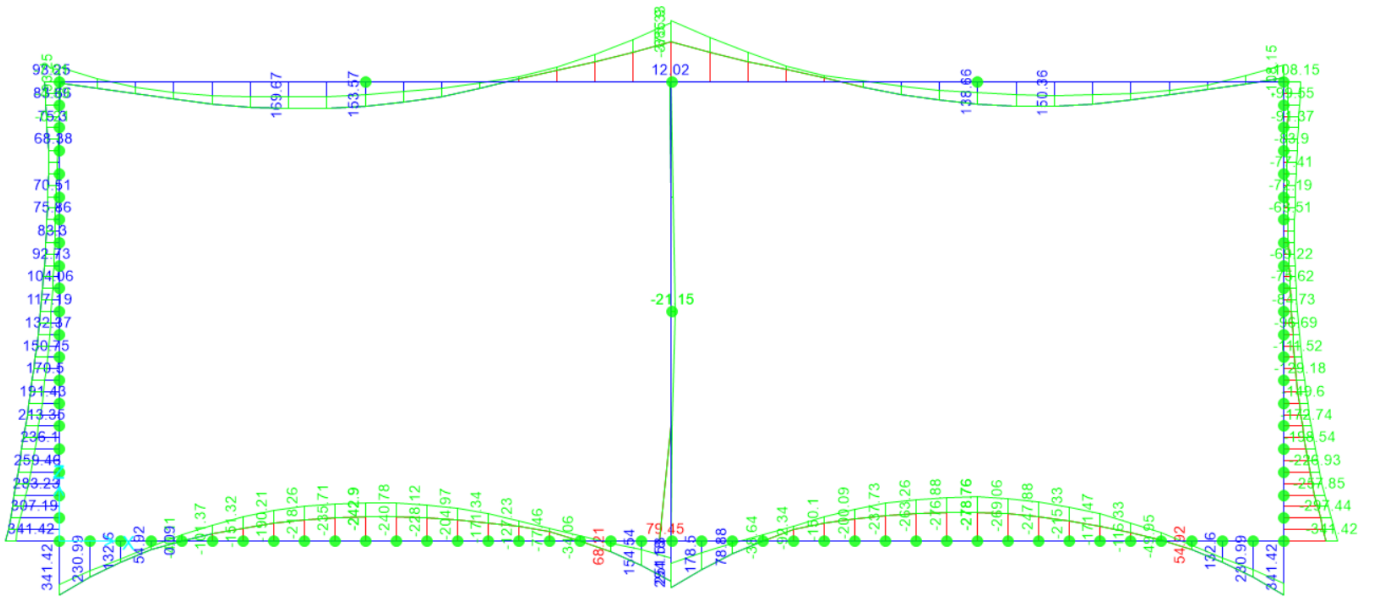
Figura 10.11 – Involuppo SLE momento flettente
