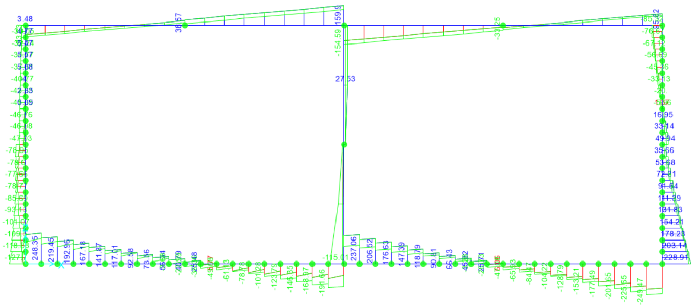
Figura 10.16 - Involuppo SLV sforzo di taglio
