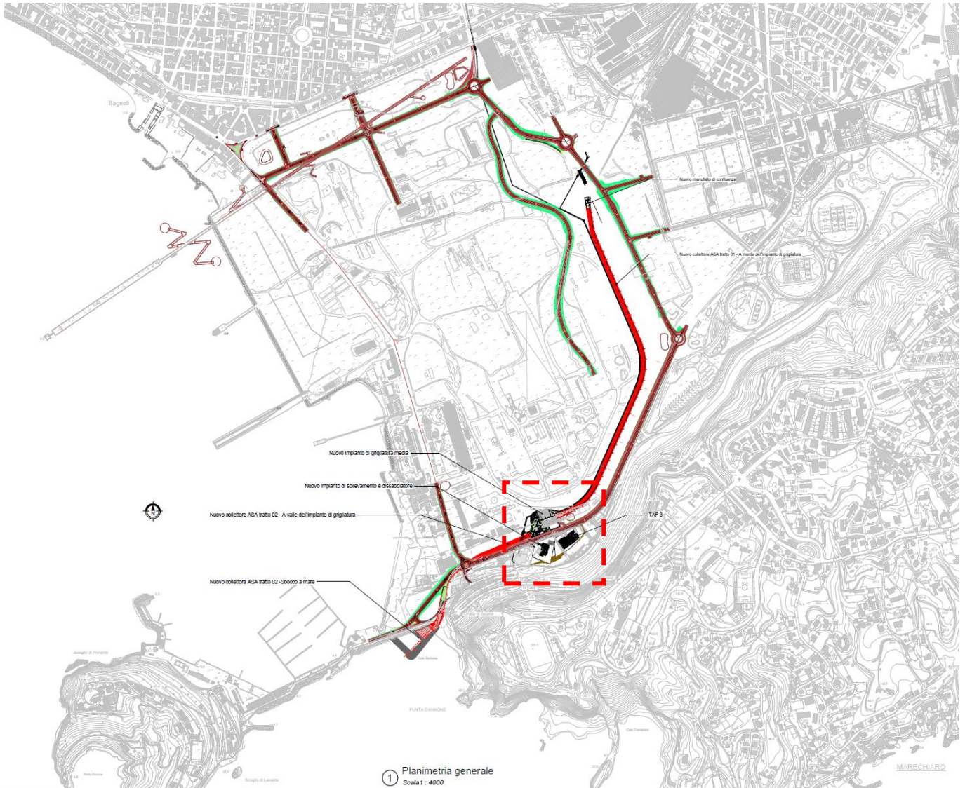
Figura 1.1.- Planimetria generale e inquadramento dell' opera
