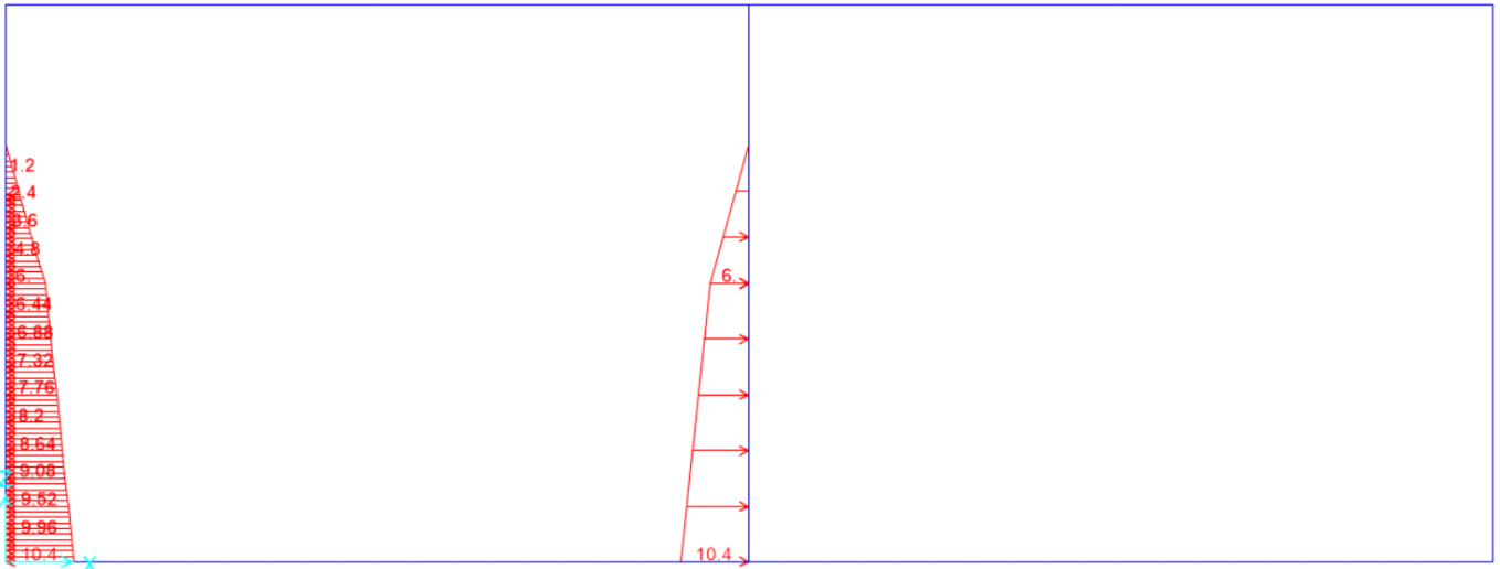
Figura 10.5 - condizione di carico u_{din} – spinta idrodinamica dell'acqua vasca sinistra
