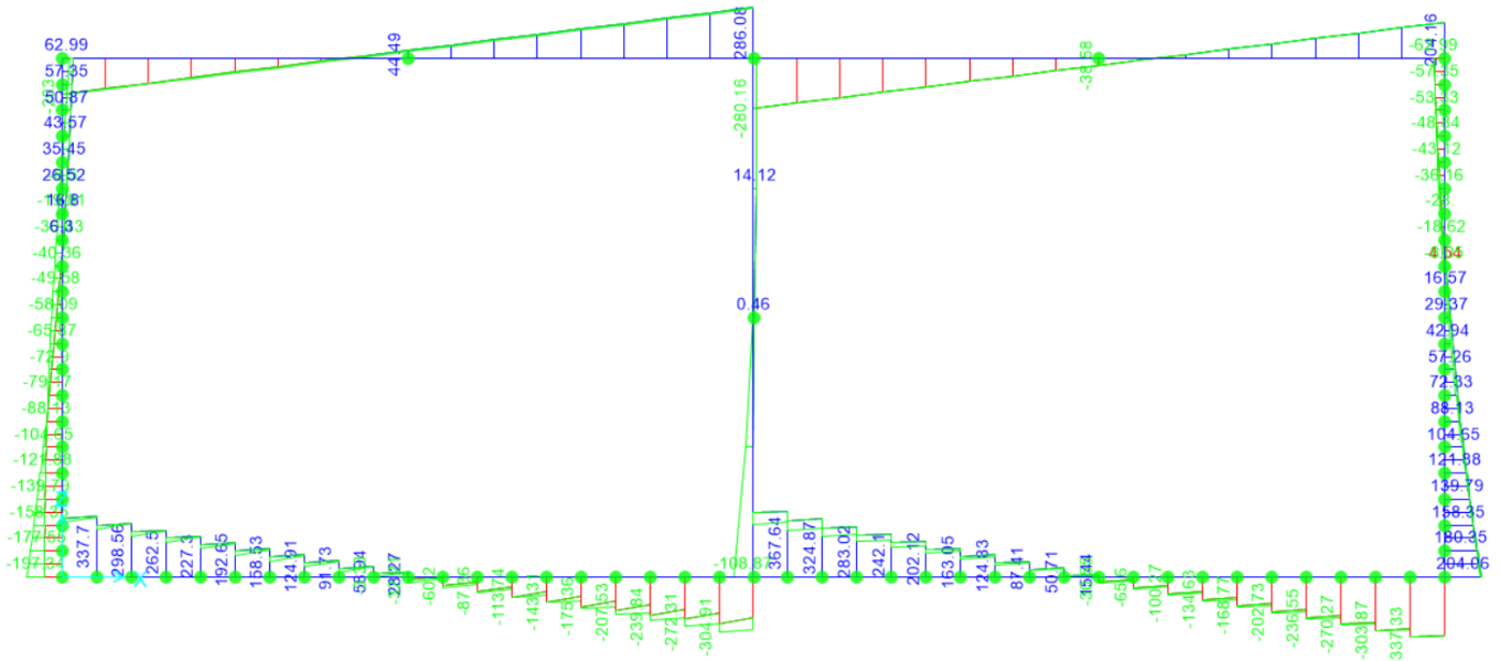
Figura 10.13 – Inviluppo SLU sforzo di taglio
