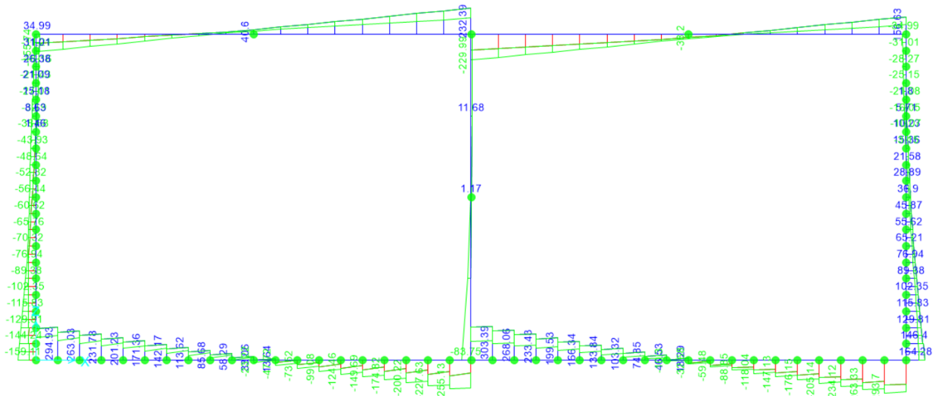
Figura 10.10 – Involuppo SLE sforzo di taglio
