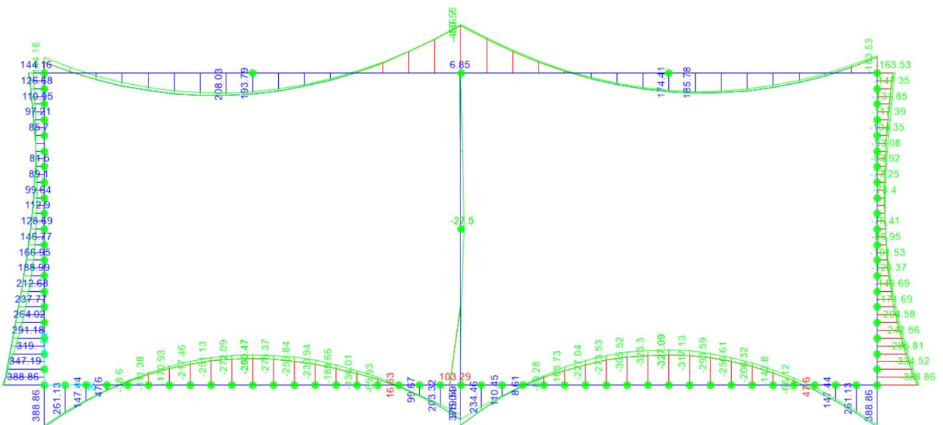
Figura 10.14 – Inviluppo SLU momento flettente
