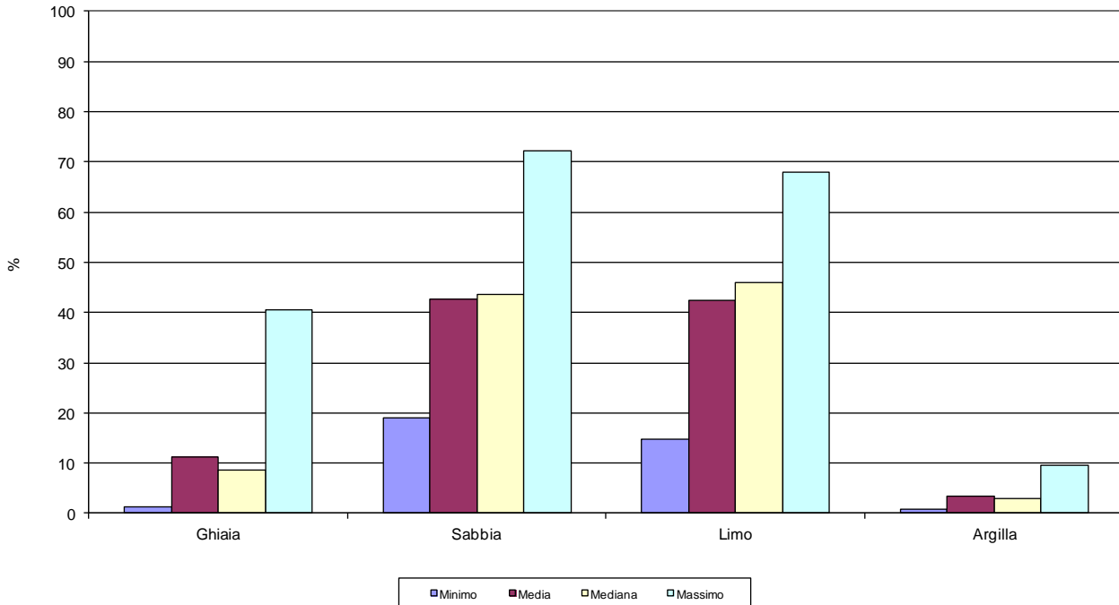
Figura 4.4 - Frazioni granulometriche nelle sabbie limose
