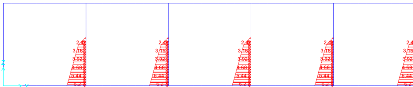
Figura 9.8 - condizione di carico S – spinta idrodinamica
