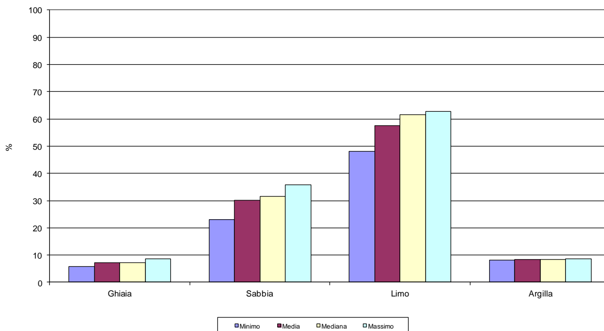
Figura 4.6 - Frazioni granulometriche nei limi torbosi
