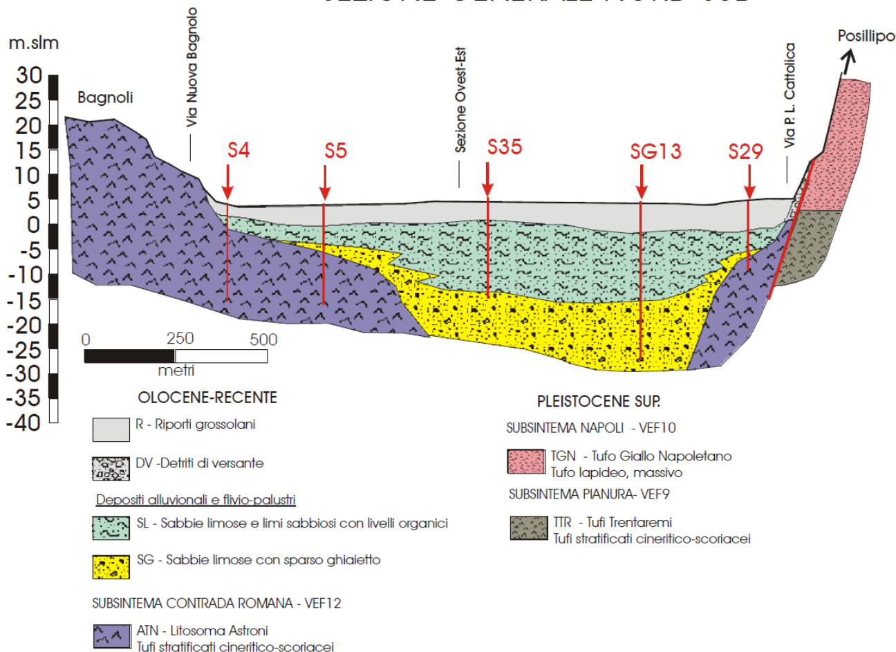
Figura 4.10 - Sezione geologica generale Nord-Sud
