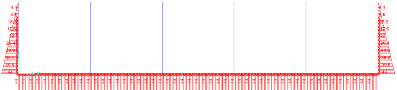
Figura 9.5 - condizione di carico P – spinta idrostatica esterna
