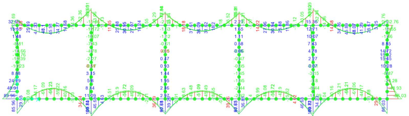
Figura 9.15 – Inviluppo SLU momento flettente
