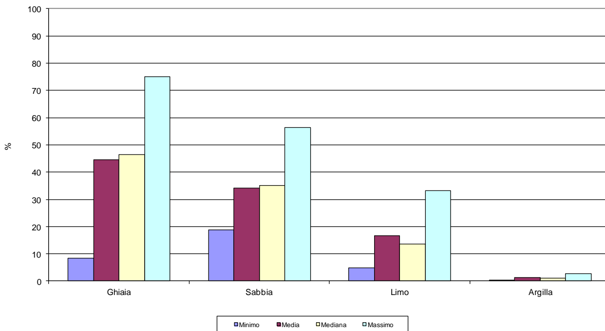
Figura 4.2 - Frazioni granulometriche nei riporti
