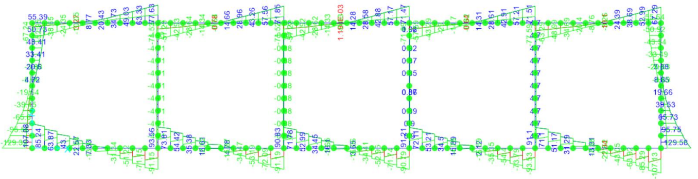
Figura 9.11 – Involuppo SLE sforzo di taglio
