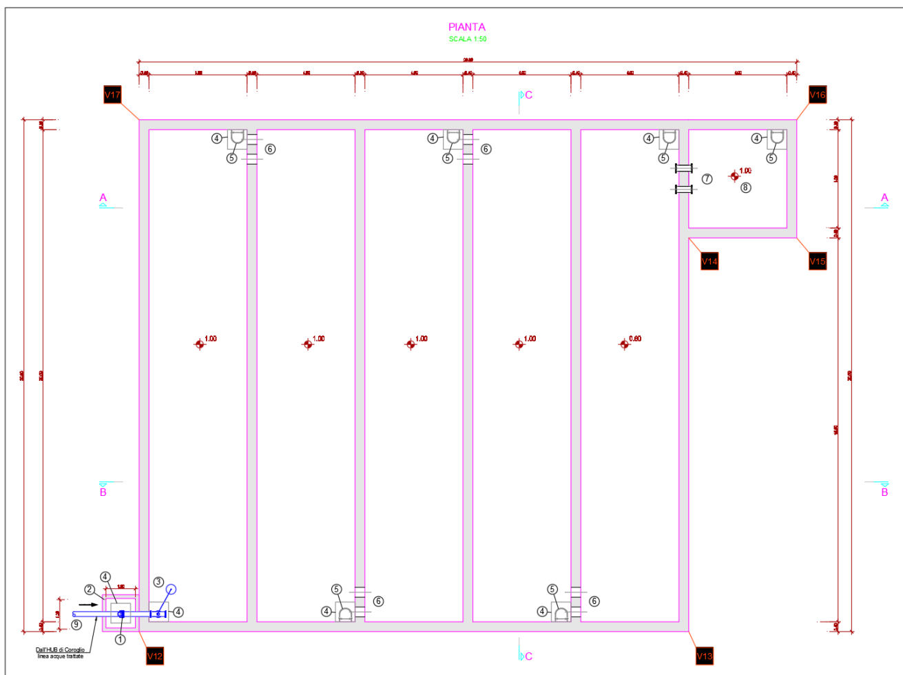
Figura 1.1 – Pianta vasca di accumulo
