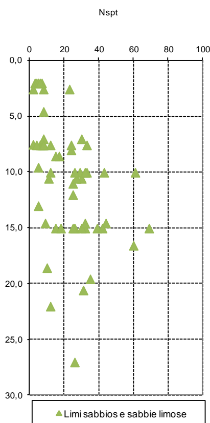
Figura 4.3 – valori penetrometrici SPT nei limi sabbiosi
