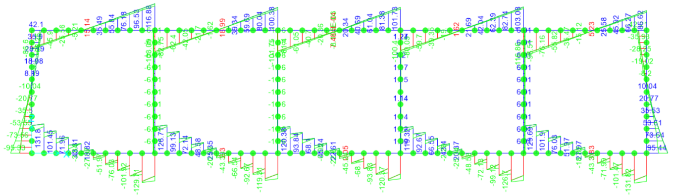
Figura 9.14 – Inviluppo SLU sforzo di taglio
