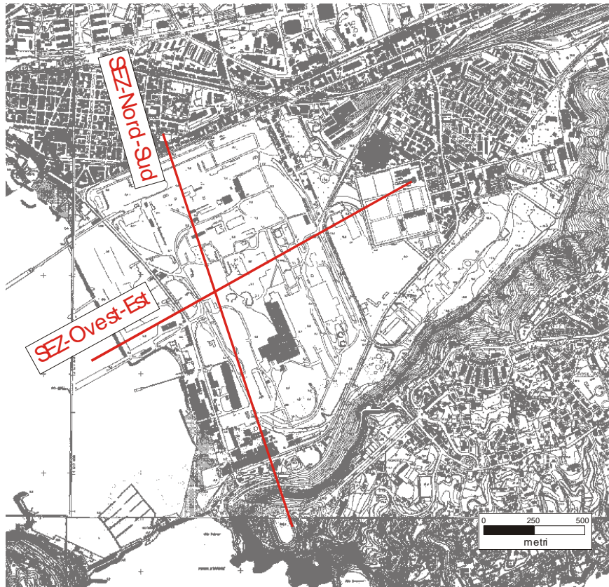
Figura 4.9 - Traccia delle sezioni geologiche generali
