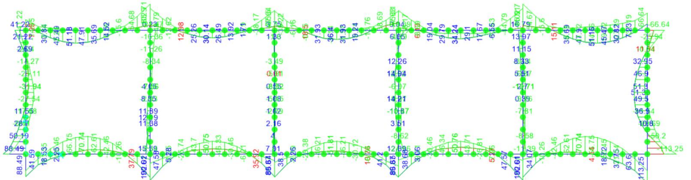
Figura 9.18 - Involuppo SLV momento flettente
