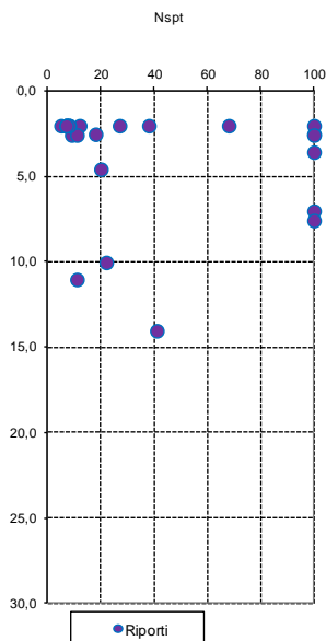
Figura 4.1 – valori penetrometrici SPT nei terreni di riporto
