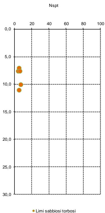
Figura 4.5– valori penetrometrici SPT nei limi torbosi (S 27, S28).
