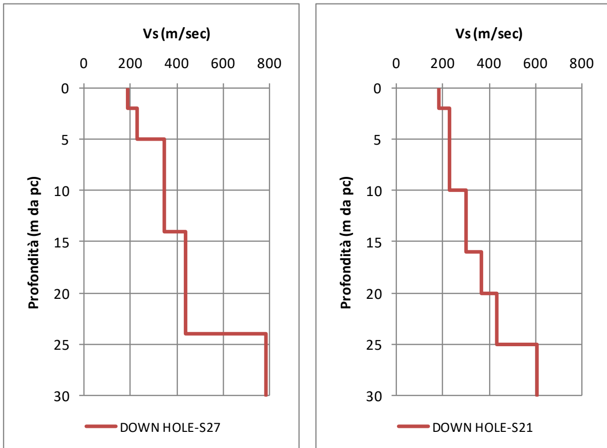
Figura 5.2 - Andamento delle Vs della Down-Hole S27 (Categoria di Sottosuolo B) e della Down-Hole S21 (Categoria di Sottosuolo C).
