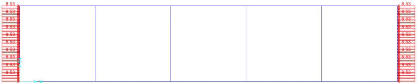
Figura 9.4 - condizione di carico q – spinta da sovraccarico
