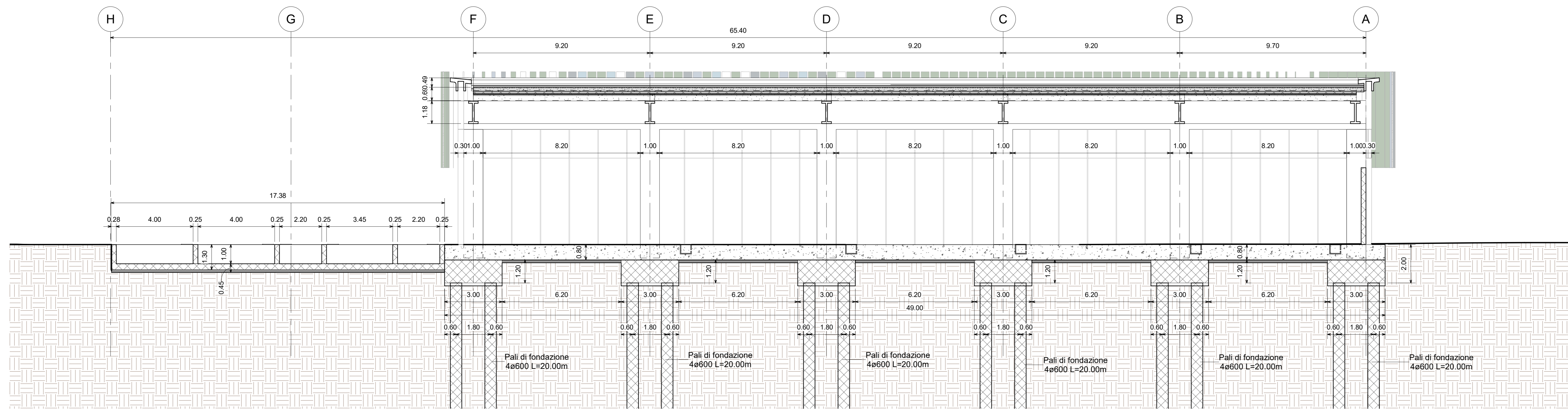
8 Sezione 8 Scala 1 : 100
