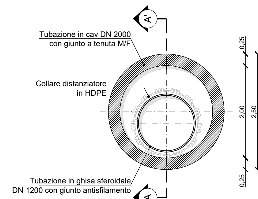
SEZIONE TRASVERSALE B-B' rapp. 1: 50
