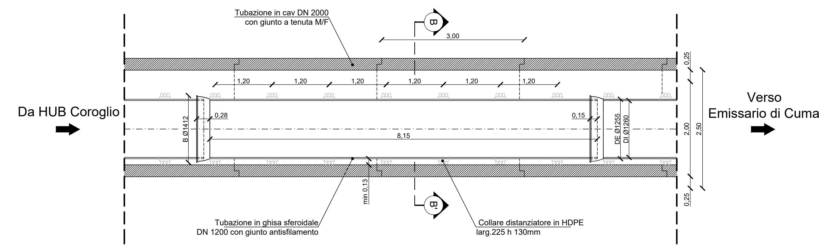
SEZIONE LONGITUDINALE rapp. 1: 50
