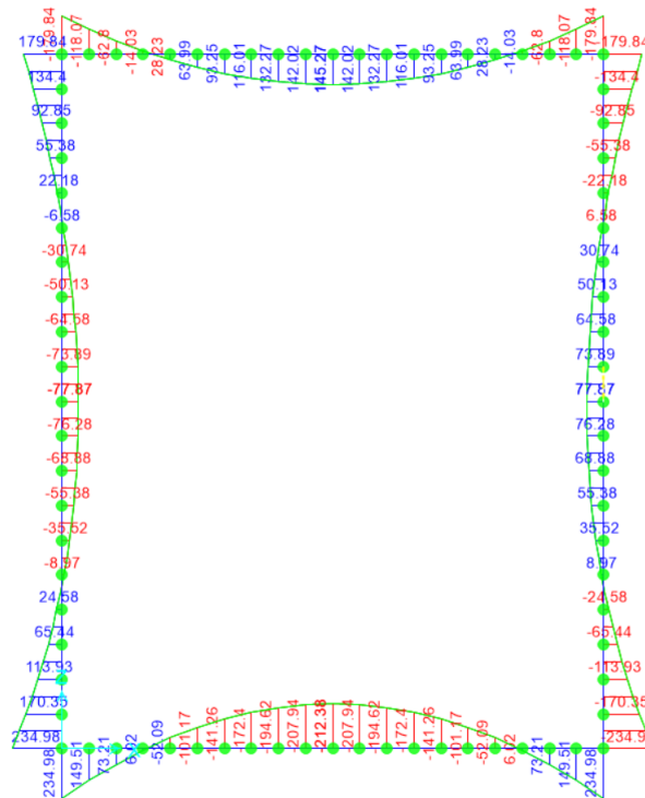
Figura 10.8 – Inviluppo SLE momento flettente
