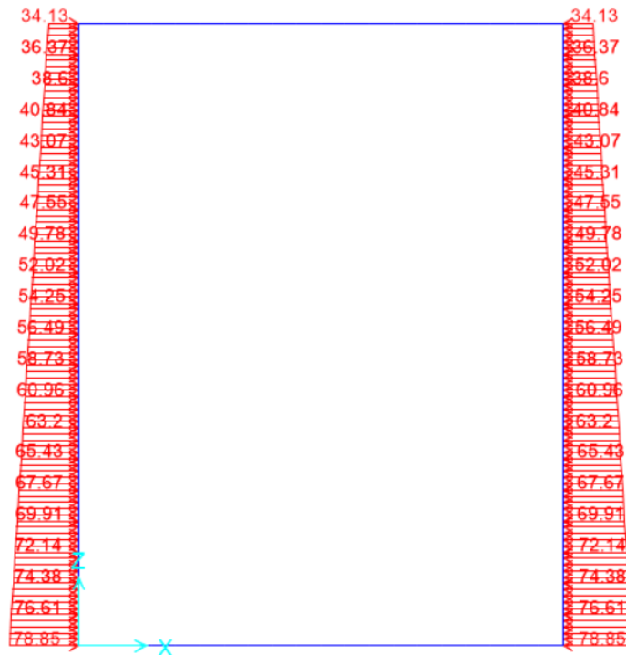
Figura 10.3 - condizione di carico g1 – spinta del terreno
