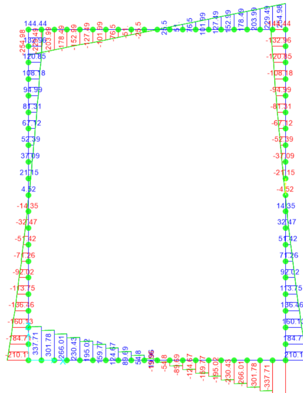
Figura 10.6 – Inviluppo SLE sforzo normale
