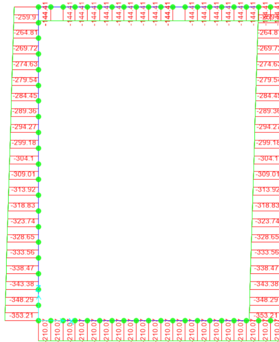
Figura 10.6 – Inviluppo SLE sforzo normale
