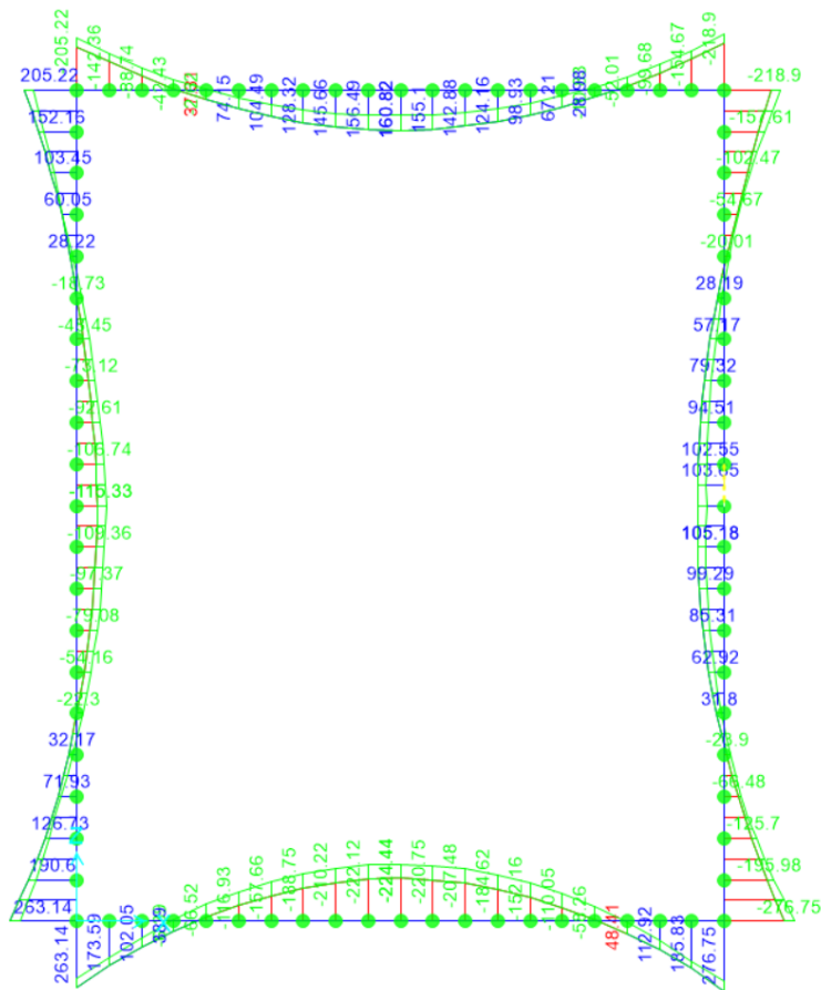
Fig. 11 - Inviluppo SLV momento flettente
