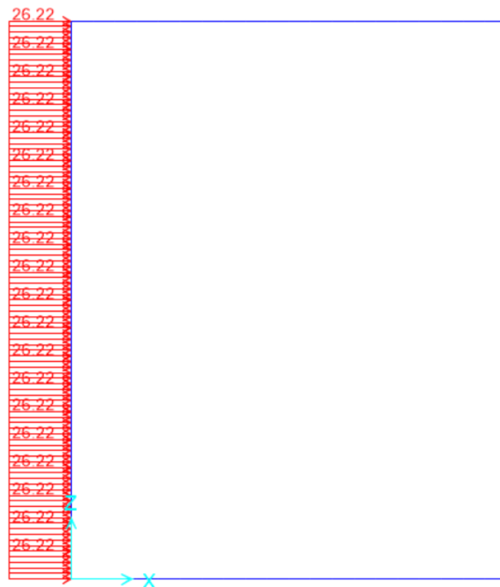
Figura 10.3 - condizione di carico g1 – spinta del terreno
