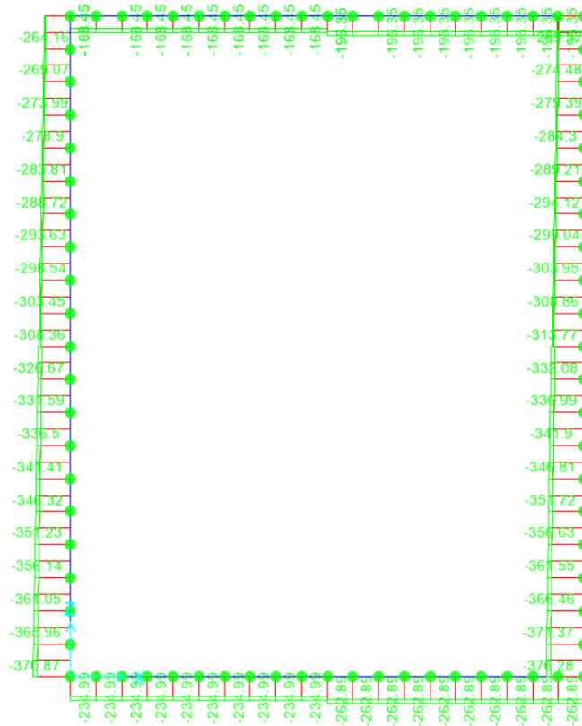
Fig. 9 - Involuppo SLV sforzo normale
