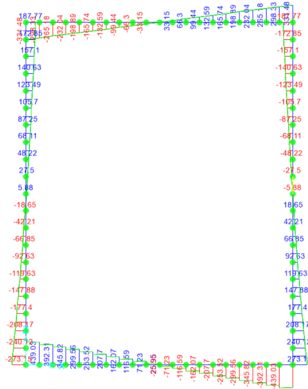
Figura 10.9 – Inviluppo SLU sforzo normale
