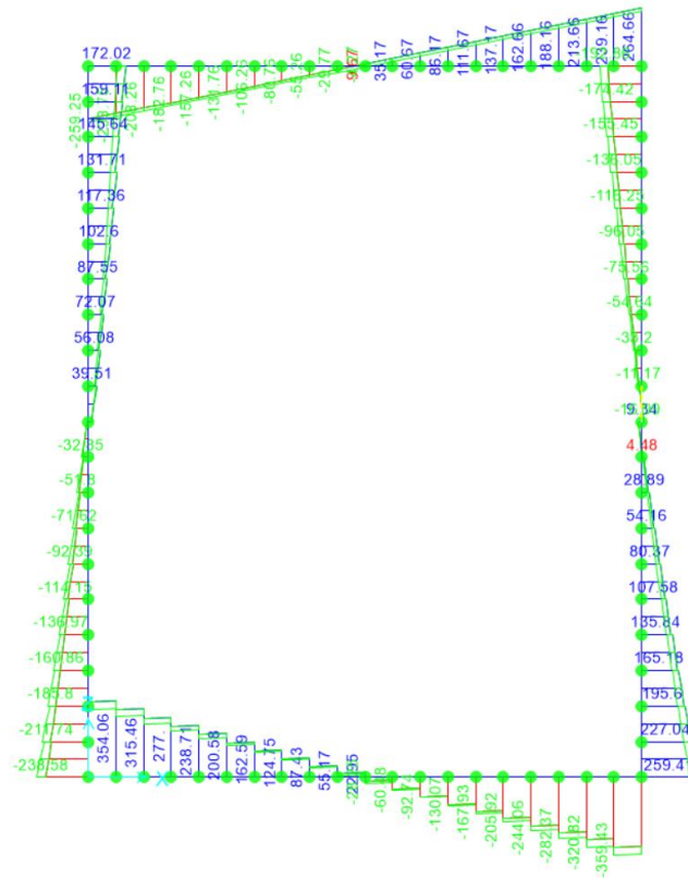
Fig. 10 - Involuppo SLV sforzo di taglio
