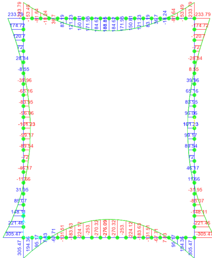
Figura 10.11 – Inviluppo SLU momento flettente
