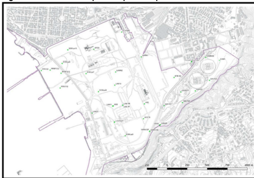
Figura: Planimetria con punti di prelievo piezometri
