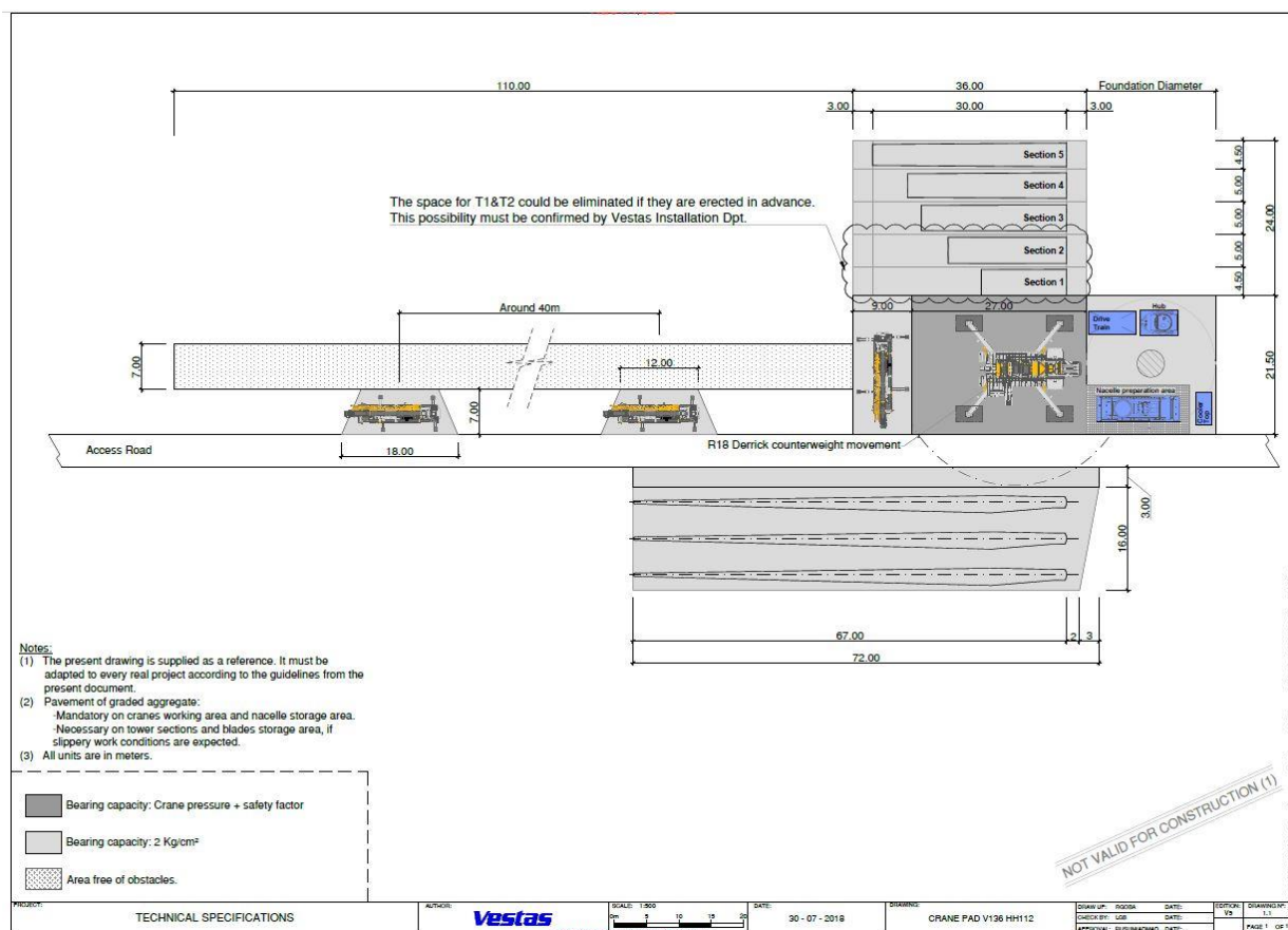
Figura 1_Schema piazzola di montaggio
