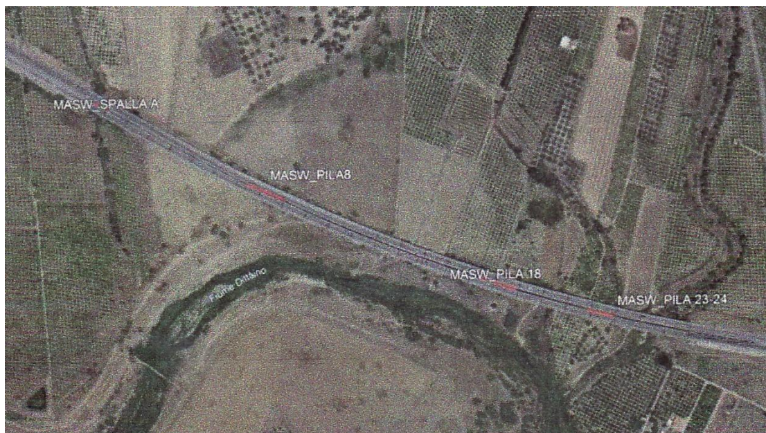
Figura 7.8 - Ubicazione delle prove MASW
