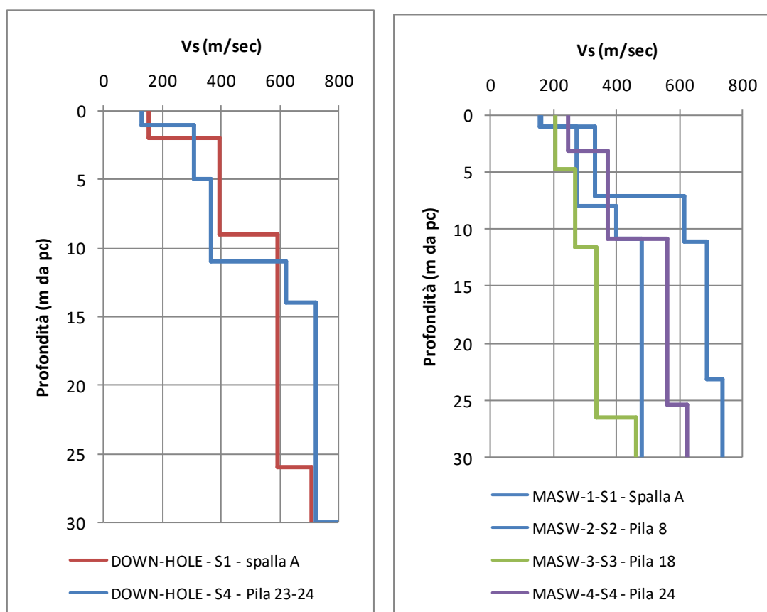
Figura 7.13 - Andamento dei valori di V_s (prove DOWN-HOLE e MASW)
