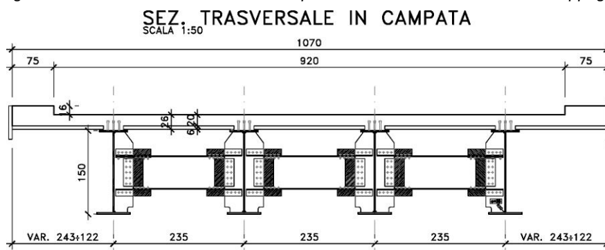
Figura 8.3. Sezione trasversale nuovo impalcato a 4 travi – Sezione corrente
