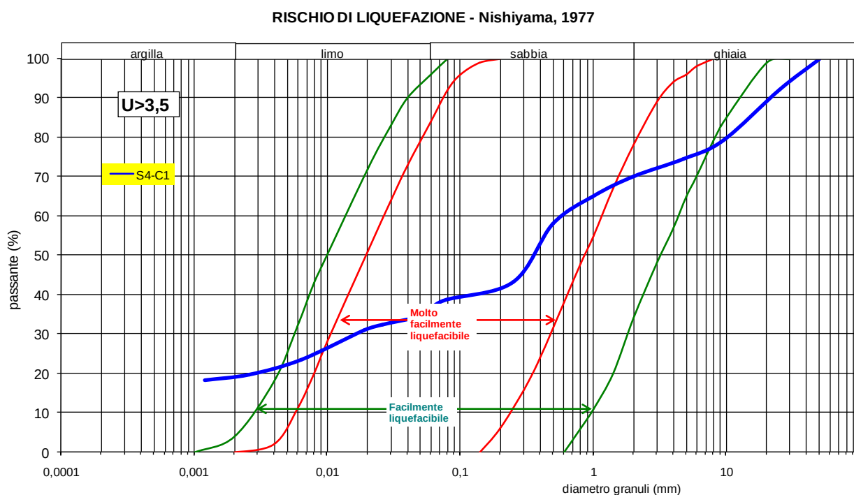
Figura 7.14 - Fuso di potenziale liquefacibilità
