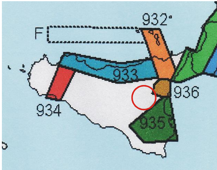
Figura 7.10 – Zonazione sismogenetica ZS9 (INGV, 2004)
