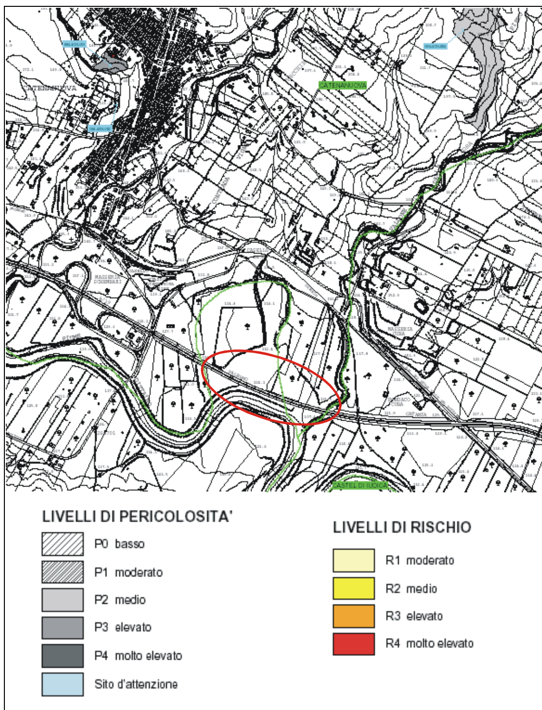
Figura 7.3 - Carta di Pericolosità e Rischio geomorfologico (PAI – TAV. 63010-71)
