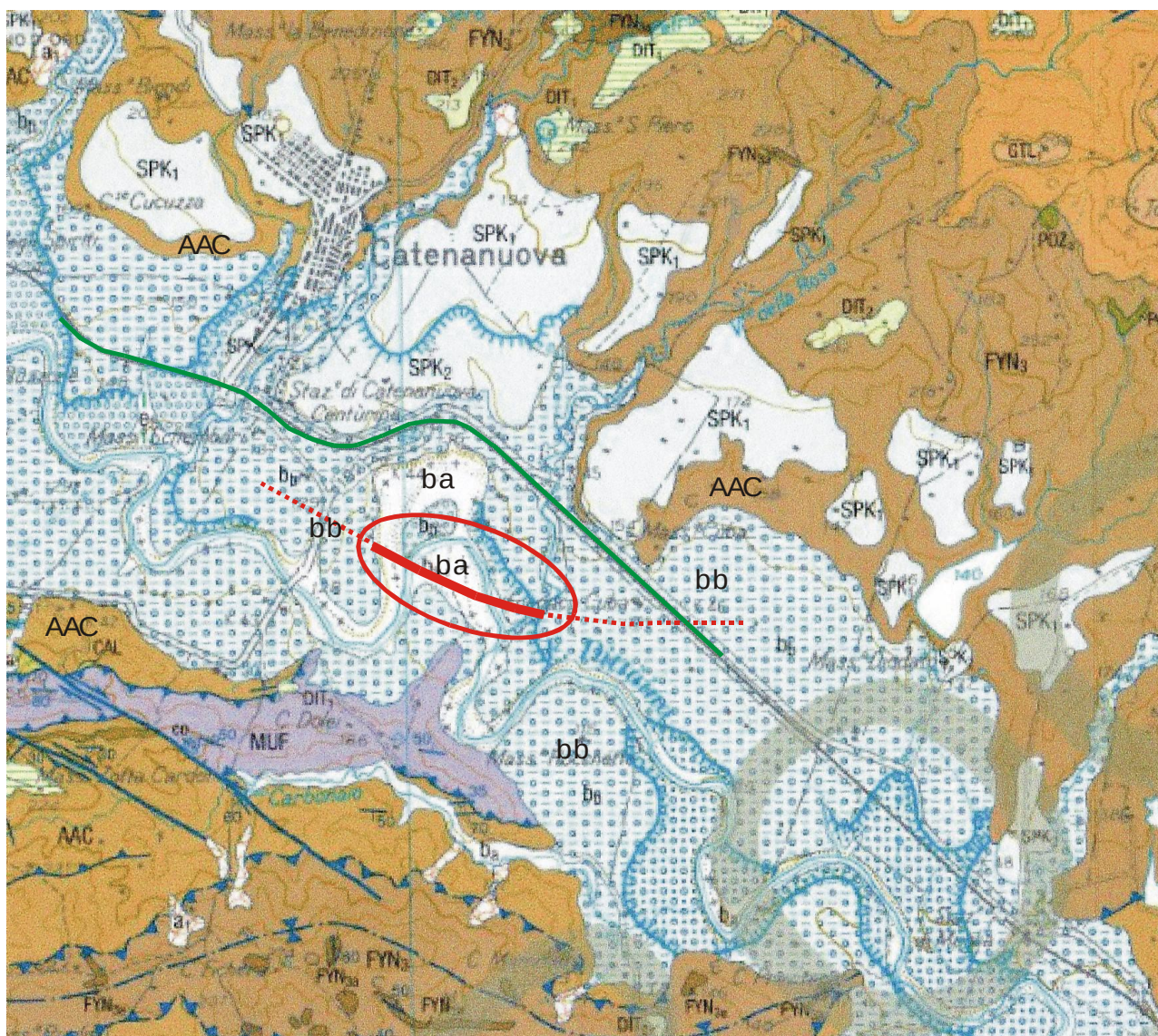
Figura 7.4 - Ubicazione dell'area nel contesto geologico locale
