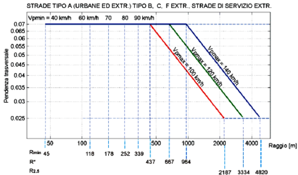
Figura 2. D.M. 05.11.2001 - Abaco per il calcolo delle pendenze trasversali.
