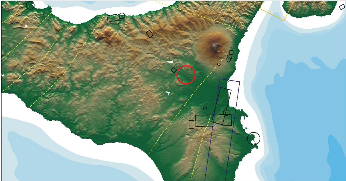
Figura 7.11 - Zone e strutture sismogenetiche (DISS-2, INGV, 2001)
