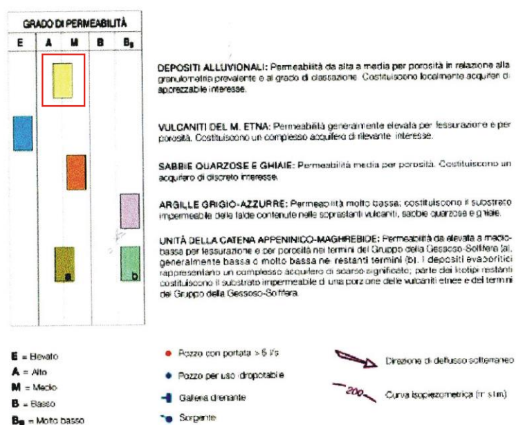
Figura 7.5 – Localizzazione dell'area in studio nel contesto idrogeologico generale.
