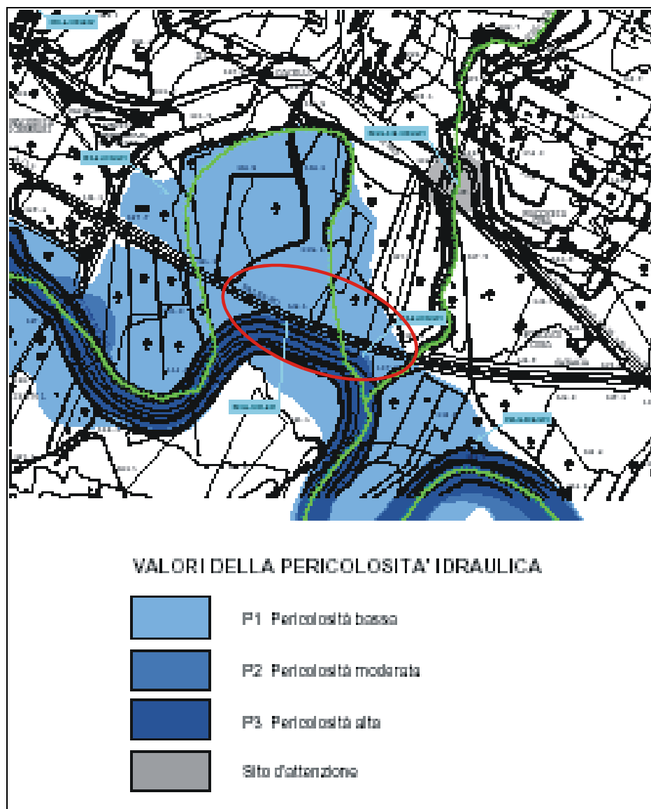
Figura 7.6 - Carta di Pericolosità Idraulica per fenomeni di esondazione (PAI – TAV. 63010-71)
