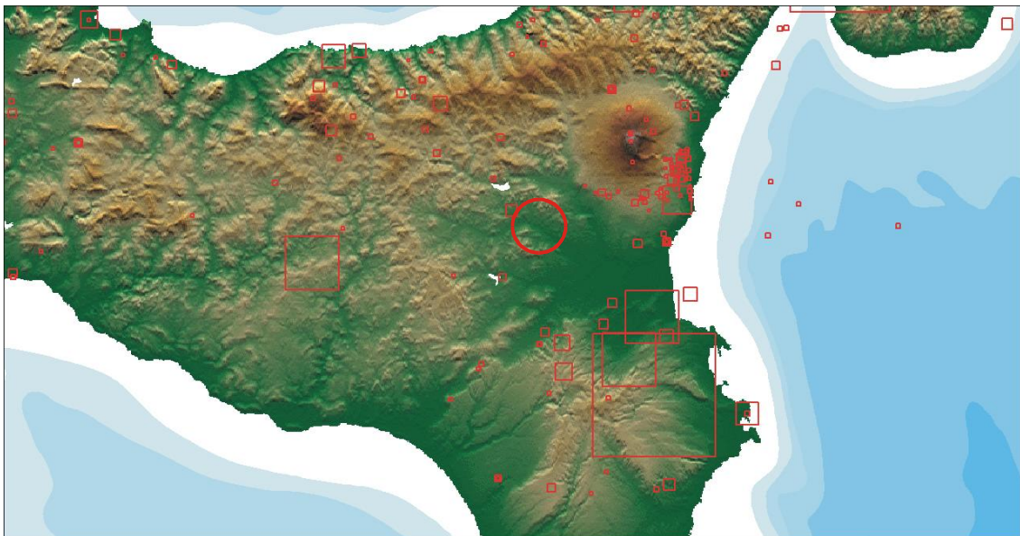
Figura 7.12 - Localizzazione dei sismi storici (Catalogo CPTI, DISS-2, INGV, 2001)
