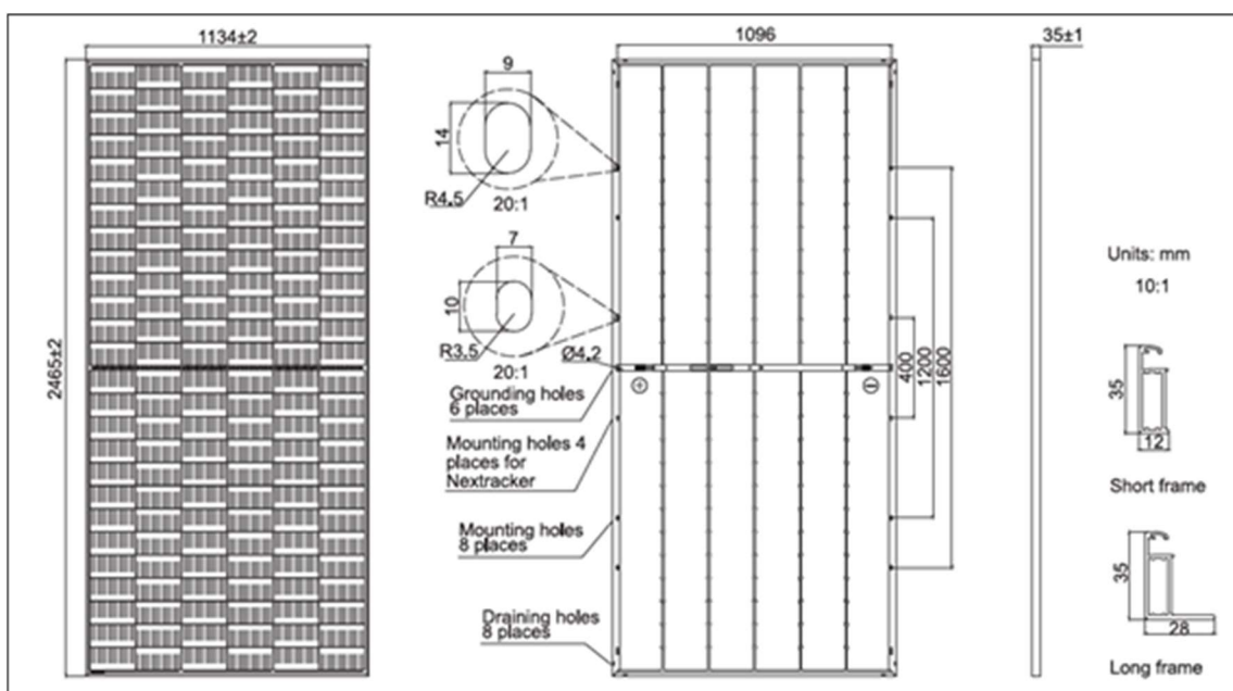
Figura 3.1-1 - Caratteristiche pannelli fotovoltaici
