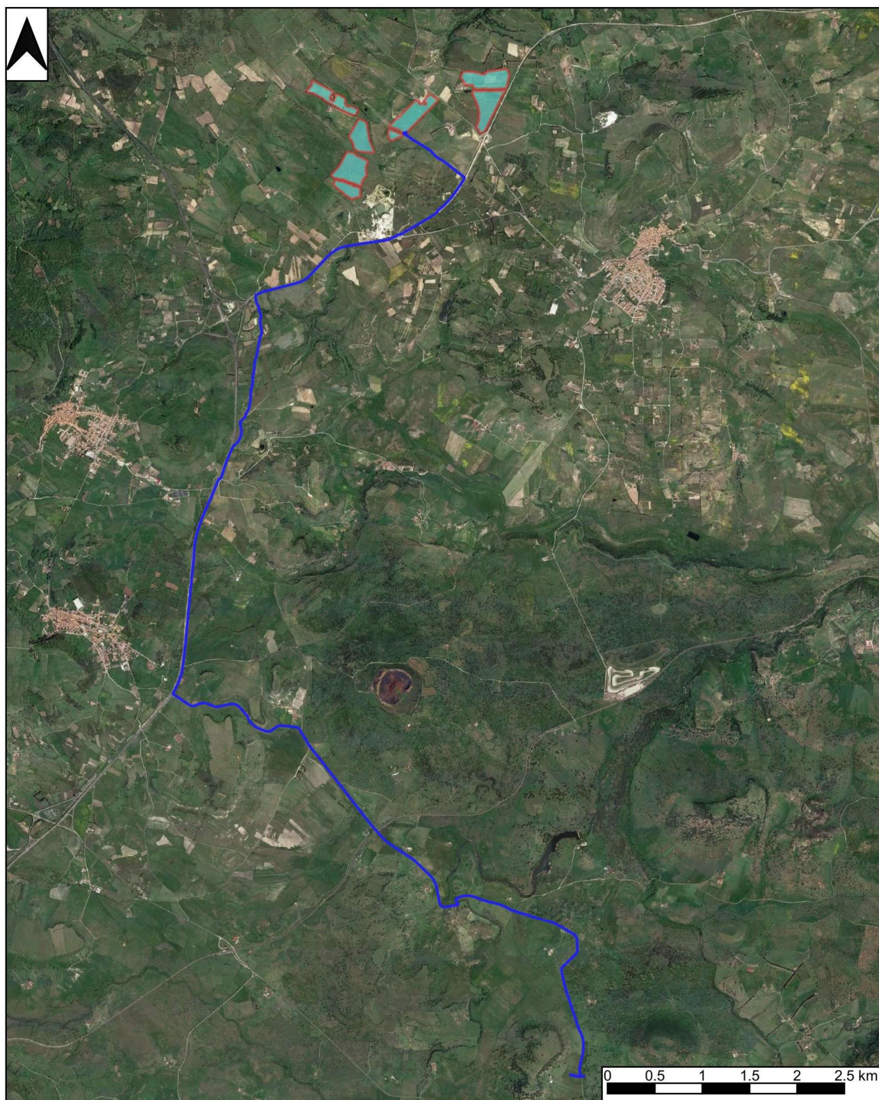
Figura 3.6-7 – Localizzazione cavidotto
