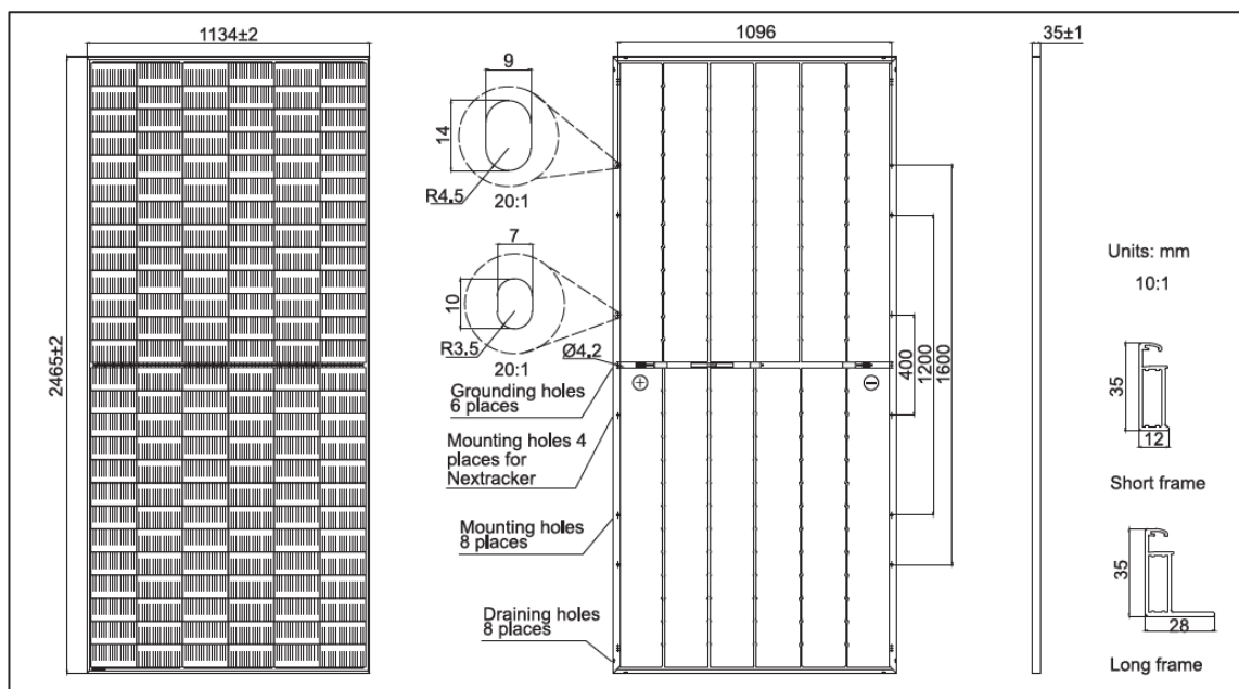
FIGURA 7: PANNELLO FV PARI A 625 WP CON DIMENSIONI 2465 x 1134 x 35 MM
