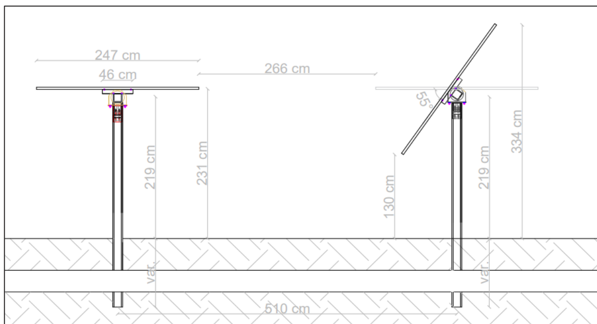
FIGURA 4: TRACKER TIPO AD ASSE VARIABILE
