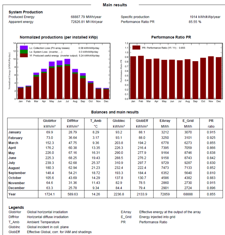
FIGURA 5: PRODUCIBILITA' ELETTRICA DELL'IMPIANTO AGRIVOLTAICO VALUTATA TRAMITE PVSYS
