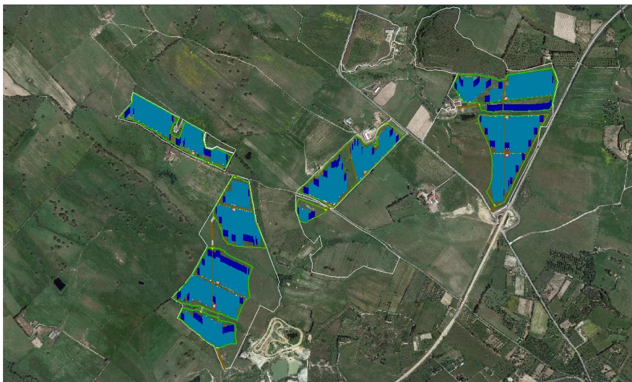
FIGURA 1: LAYOUT D' IMPIANTO
