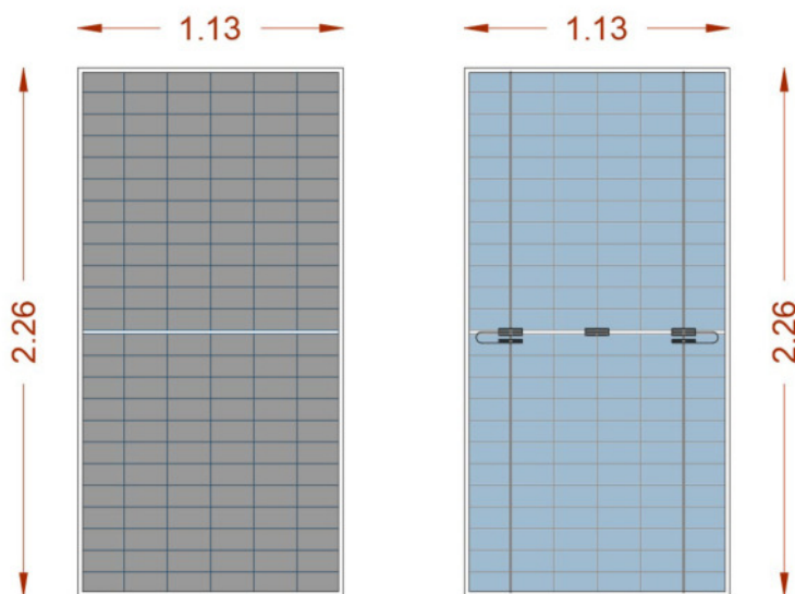
Figura 5: Dettaglio modulo FV.
