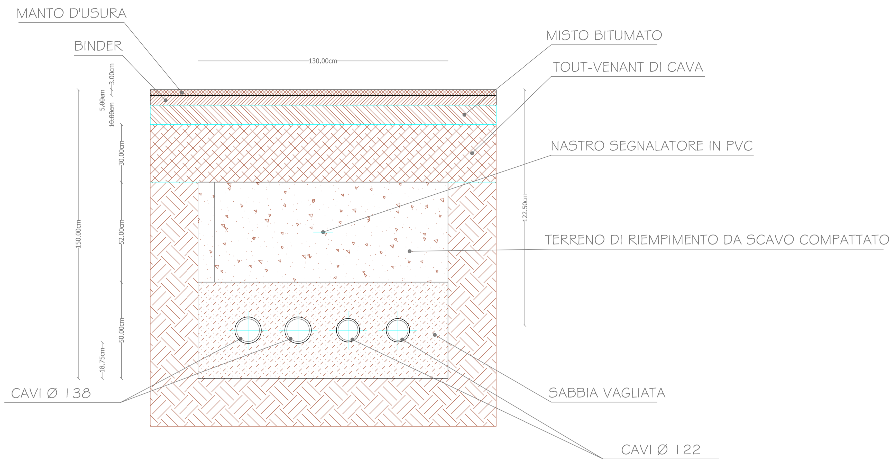
SEZIONE TIPO CAVIDOTTI MEDIA TENSIONE POSA DIRETTAMENTE INTERRATA Scala 1:10
