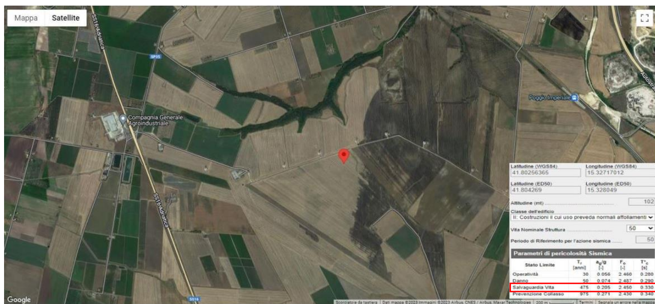
Figura 4: Parametri di pericolosità sismica del sito a_g/g , F_0 , T_c^* per i periodi di ritorno T_R di riferimento
