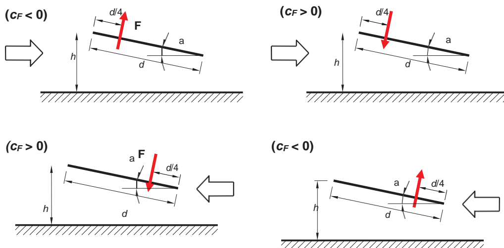
Figura 3: (Rif. Figura G.27 NTC) – Tettoie a semplice falda: posizione del punto di applicazione della forza risultante in funzione della direzione di provenienza del vento e della direzione della forza.
