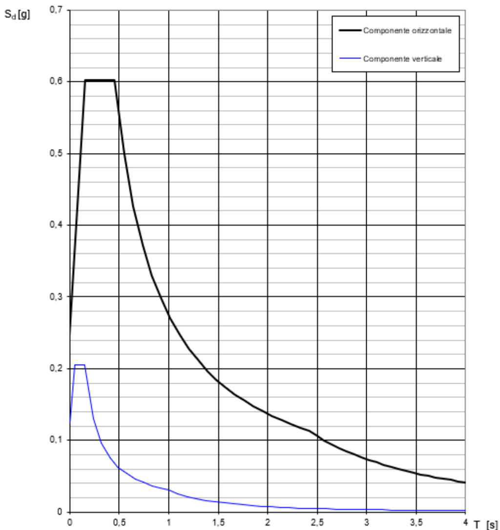
Figura 5: Spettro di risposta di progetto in termini di pseudo-accelerazione (componenti orizzontale e verticale) allo stato limite di salvaguardia della vita (SLV)
