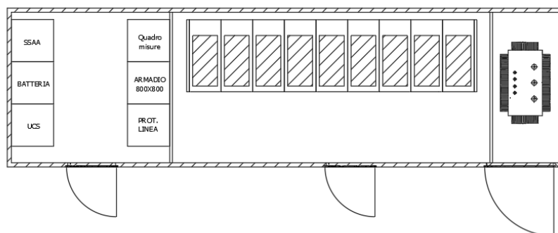
Figura05:Cabina utente di smistamento 36kV
