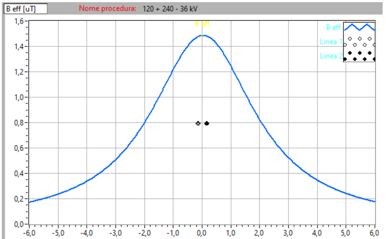
Figura 5: Profilo laterale induzione magnetica (B) a 1 m da terra- V=36 kV– B=1,48 \mu T- 1 cavo 120 e 240 mm 2
