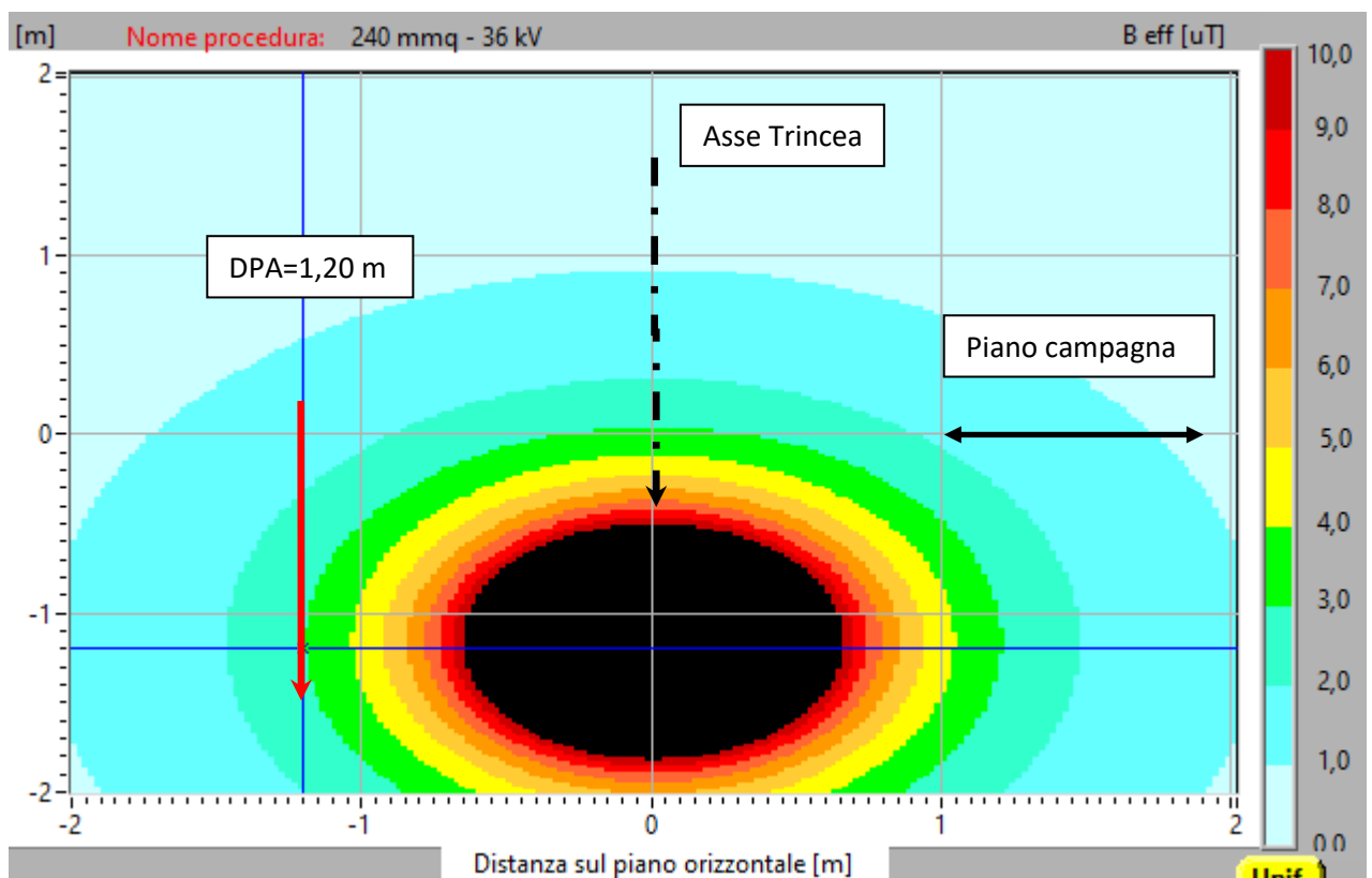
Figura 10: Mappa verticale induzione magnetica (B) sezione tipo con indicazione della DPA - V=36 kV - 1 cavo 240 mm 2
