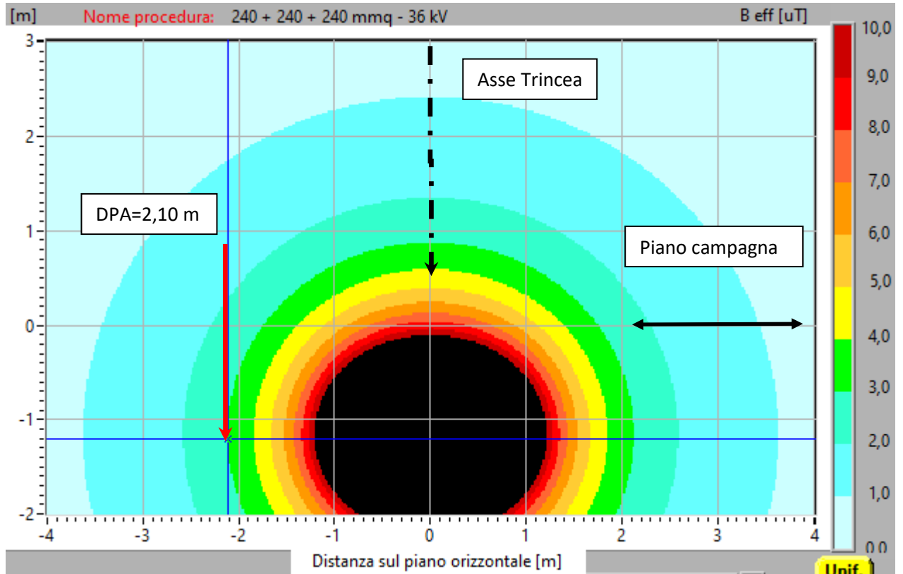
Figura 13: Mappa verticale induzione magnetica (B) sezione tipo con indicazione della DPA - V=36 kV - 3 cavi 240 mm 2
