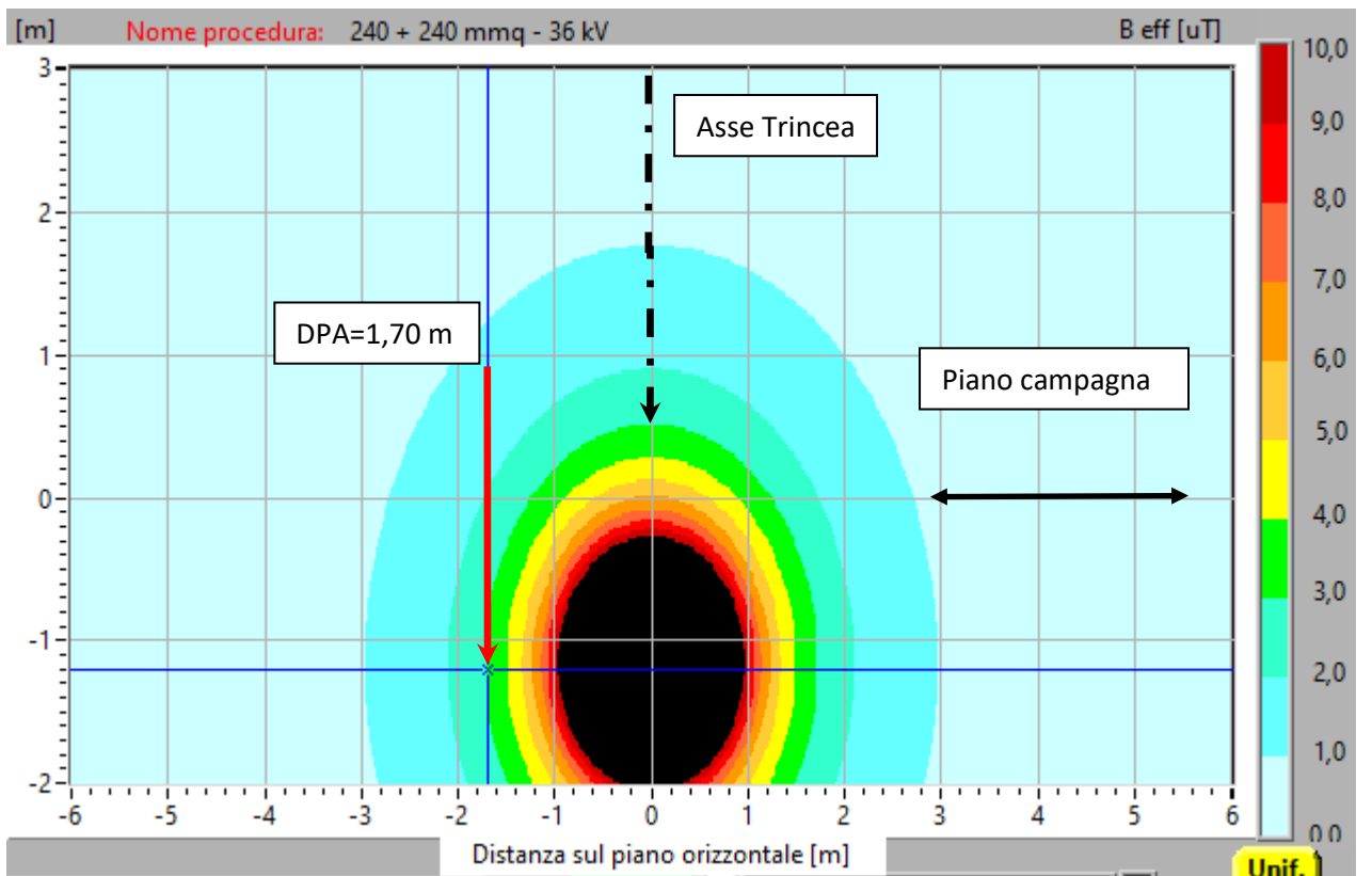
Figura 12: Mappa verticale induzione magnetica (B) sezione tipo con indicazione della DPA - V=36 kV - 2 cavi 240 mm 2
