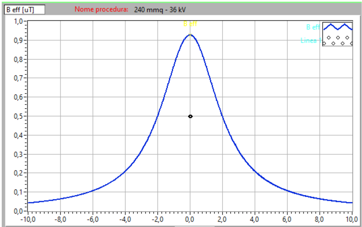
Figura 4: Profilo laterale induzione magnetica (B) a 1 m da terra- V=36 kV – B=0,93 \mu T- 1 cavo 240 mm 2
