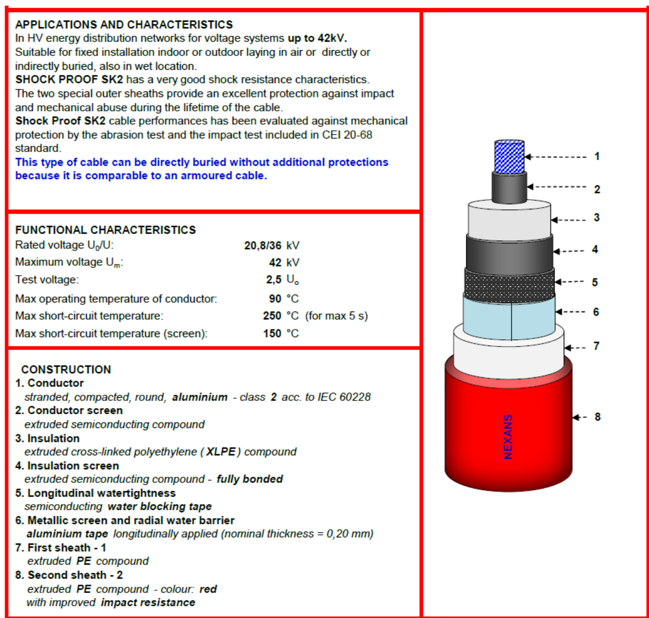
Figura 1: Schema tipo del cavo 36 kV
