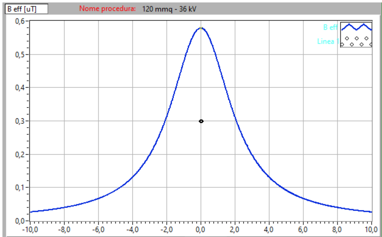
Figura 3.: Profilo laterale induzione magnetica (B) a 1 m da terra- V=36 kV- B=0,57 \mu\text{T} - 1 cavo 120 mm 2
