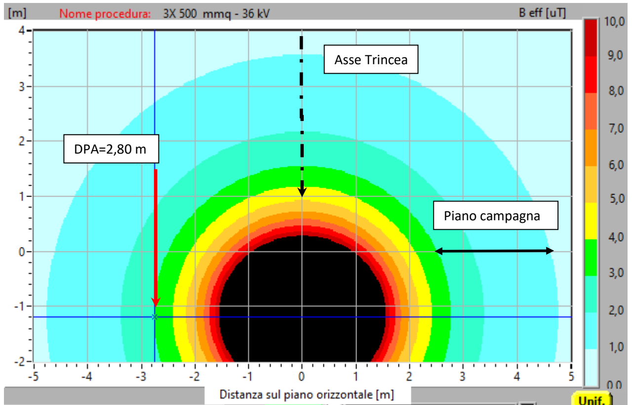
Figura 14: Mappa verticale induzione magnetica (B) sezione tipo con indicazione della DPA - V=36 kV - 3 cavi 500 mm 2
