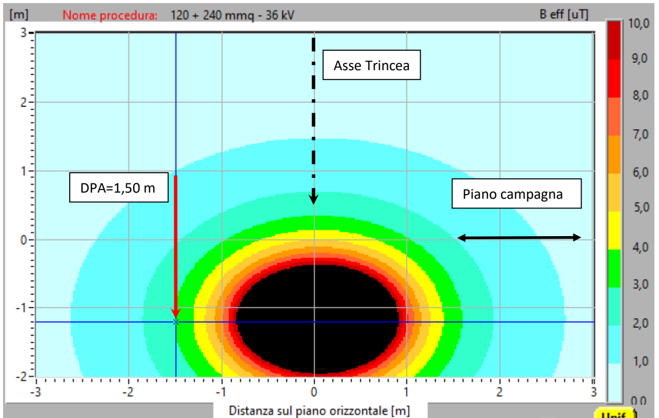
Figura 11: Mappa verticale induzione magnetica (B) sezione tipo con indicazione della DPA-V=36 kV- 1 cavo 120 e 240 mm 2
