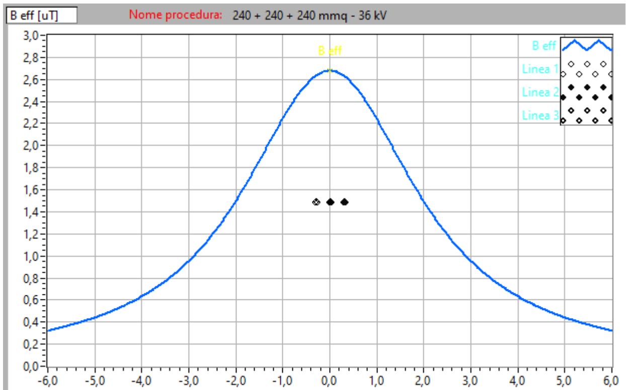
Figura 7: Profilo laterale induzione magnetica (B) a 1 m da terra- V=36 kV- B=2,68 \mu T- 3 cavi 240 mm 2
