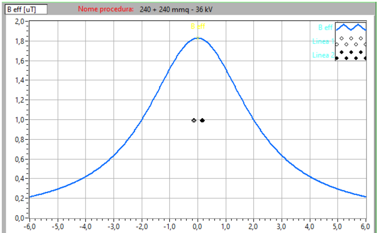
Figura 6: Profilo laterale induzione magnetica (B) a 1 m da terra- V=36 kV- B=1,83 \mu T- 2 cavi 240 mm 2
