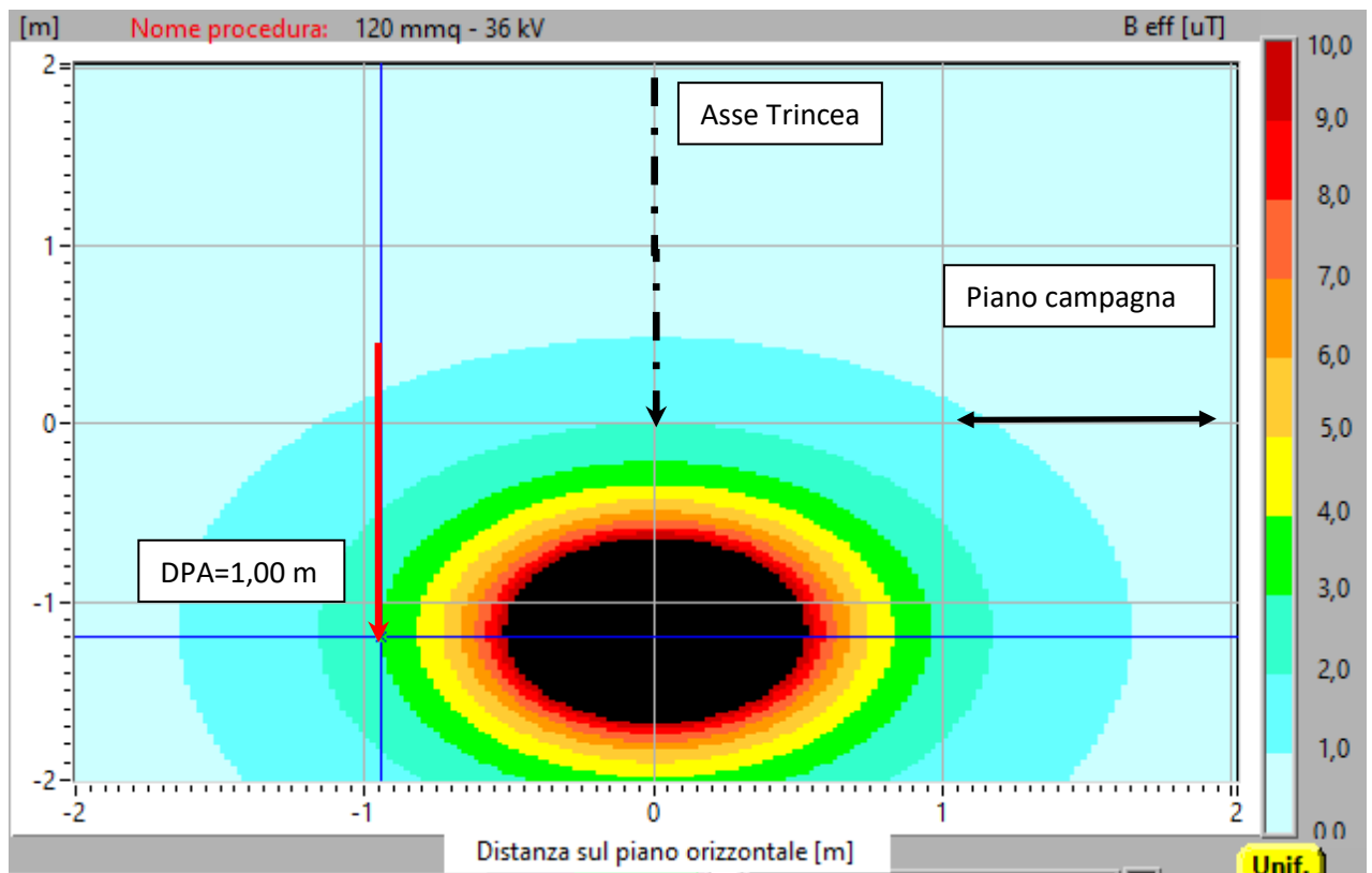
Figura 9: Mappa verticale induzione magnetica (B) sezione tipo con indicazione della DPA - V=36 kV - 1 cavo 120 mm 2
