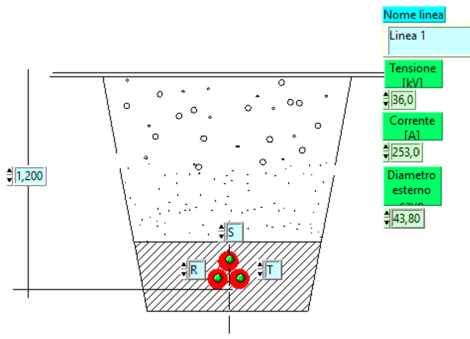
Figura 2: Posa cavo 36 kV
