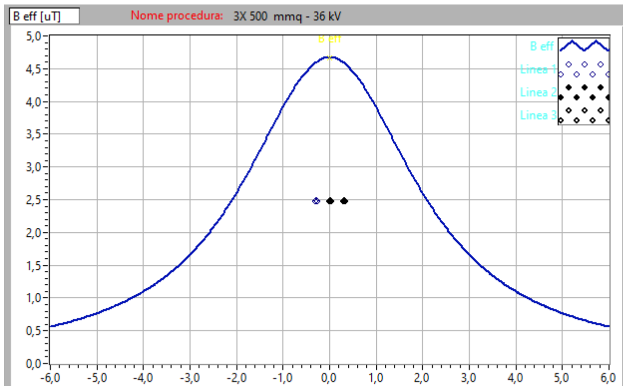
Figura 8: Profilo laterale induzione magnetica (B) a 1 m da terra- V=36 kV- B=4,67 \mu T- 3 cavi 500 mm 2
