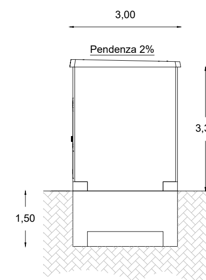
Prospetto destro
