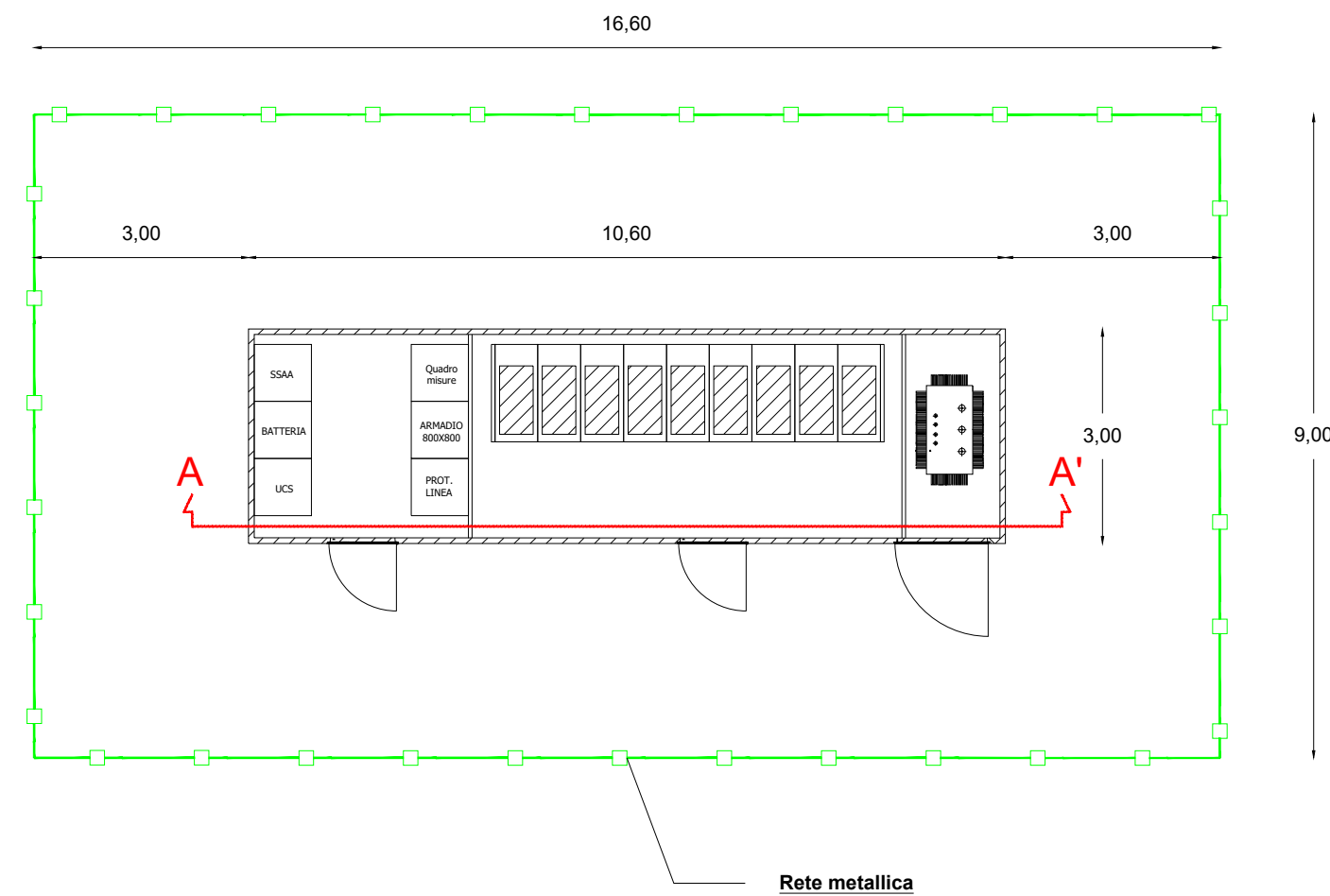
Sezione A-A'
