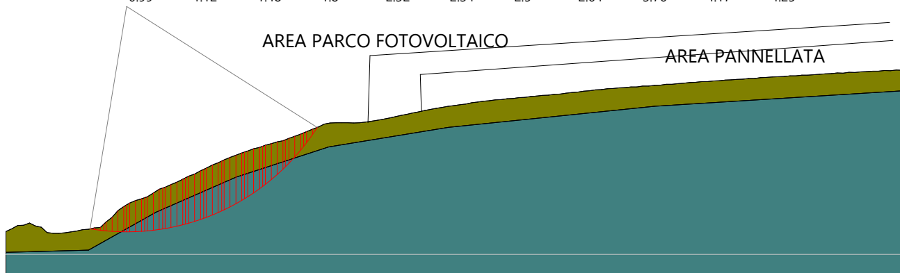
SEZIONE D-D' ANTE/POST OPERAM
