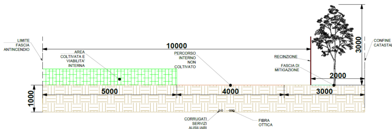
Figura 60 – Schematizzazione della fascia perimetrale degli impianti costituita dalle quinte arboree e dalla fascia tagliafuoco
