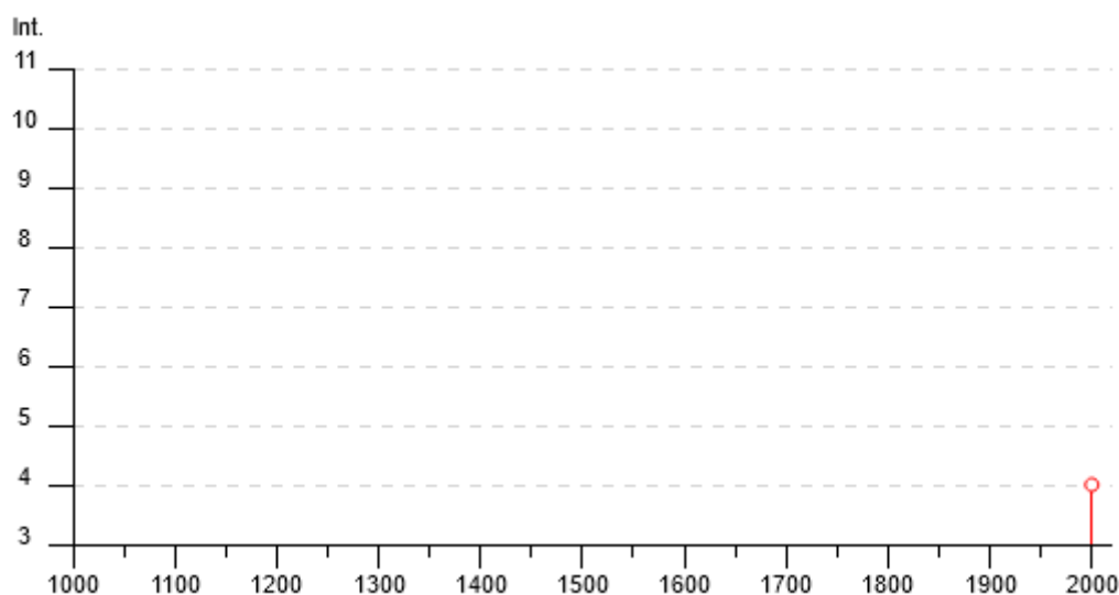
Figura n. 8-2 Grafico illustrante la storia sismica di San Gavino Monreale. Sulle ascisse sono riportati i riferimenti temporali espressi in anni, sulle ordinate le intensità sismiche (I) degli eventi rilevati (da https://emidius.mi.ingv.it/CPTI15-DBMI15_v1.5/query_place/ )
