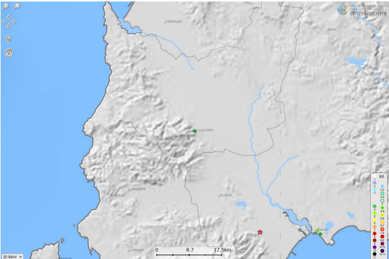
Figura n. 8-1 Stralcio DBMI15 Massime intensità macrosismiche osservate (2015)
