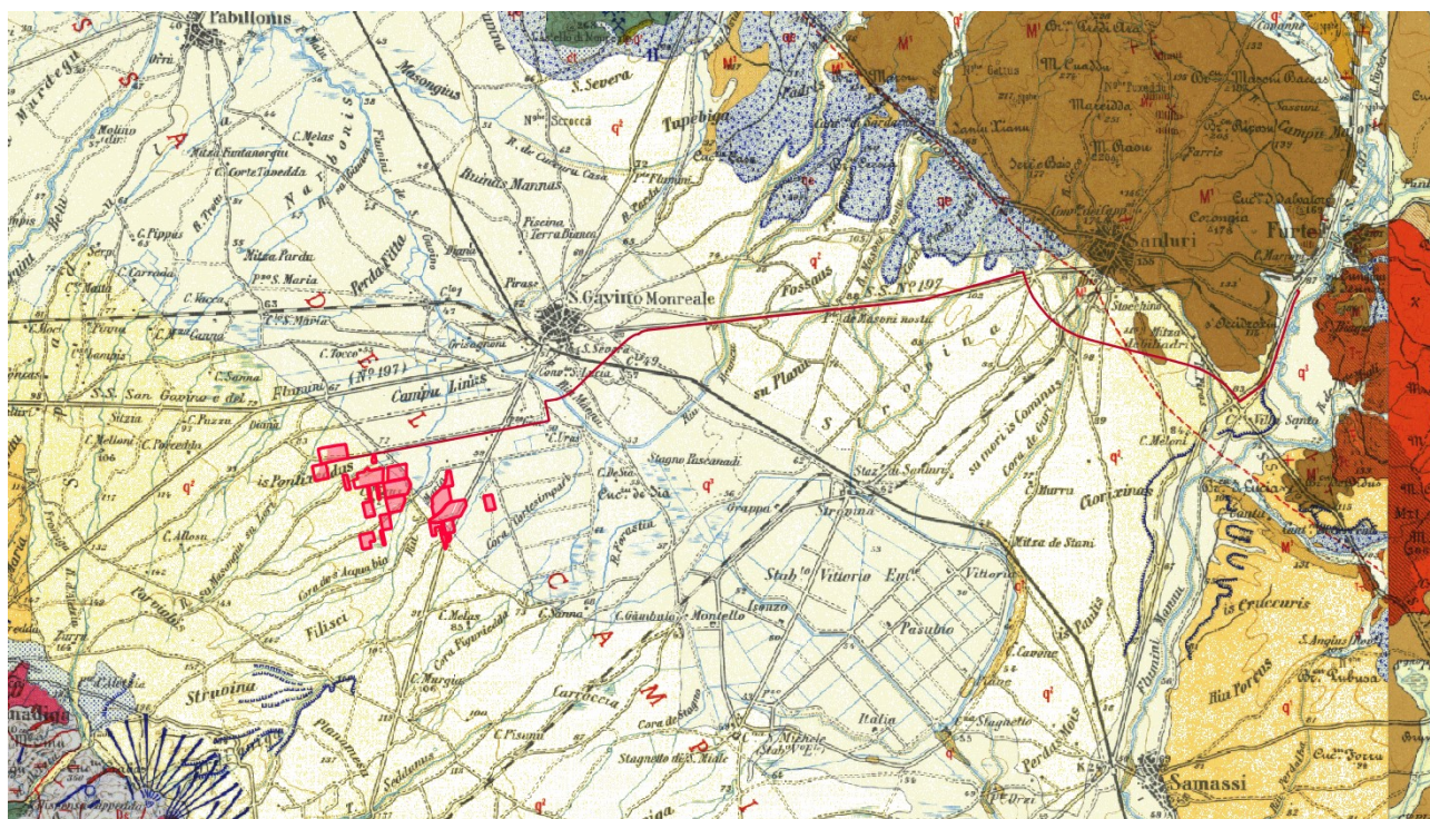
Figura n. 5-2. Stralcio del Foglio 224-225 Guspini della Carta Geologica d'Italia, scala 1:100.000 con evidenza dell'area di progetto
