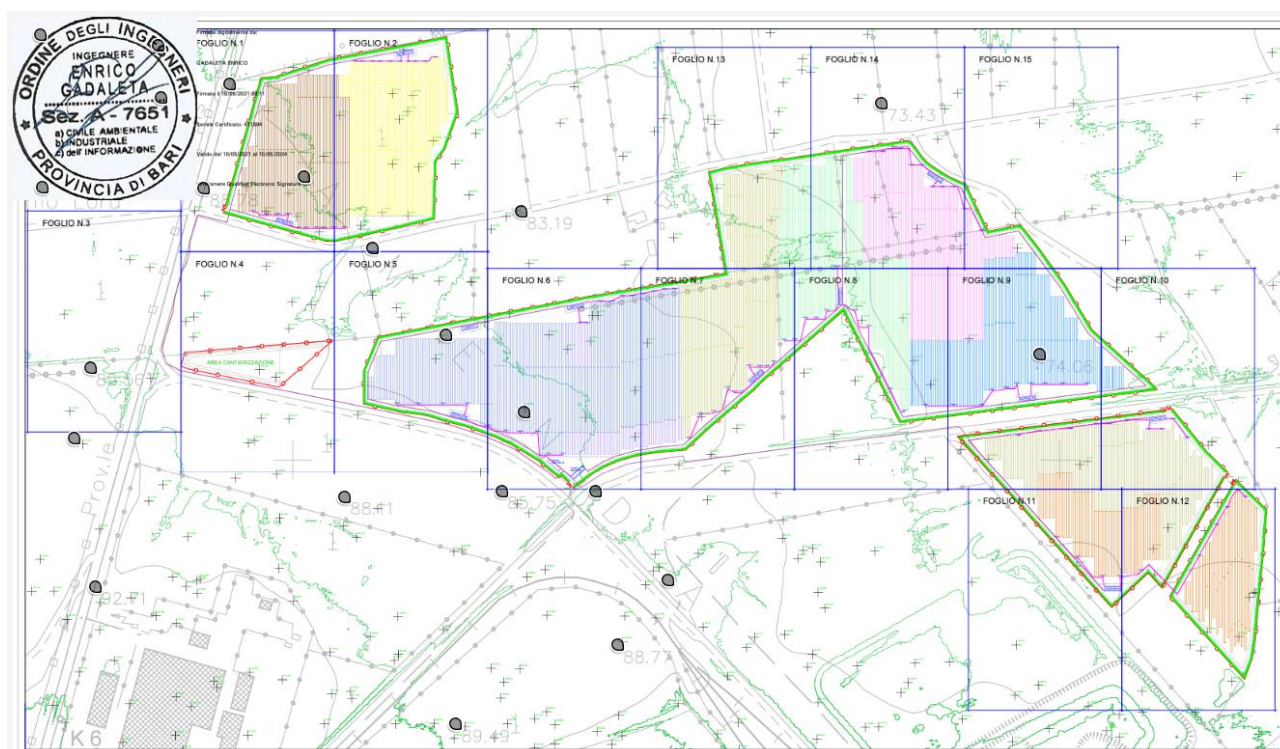
Figura 16 - Layout di progetto
