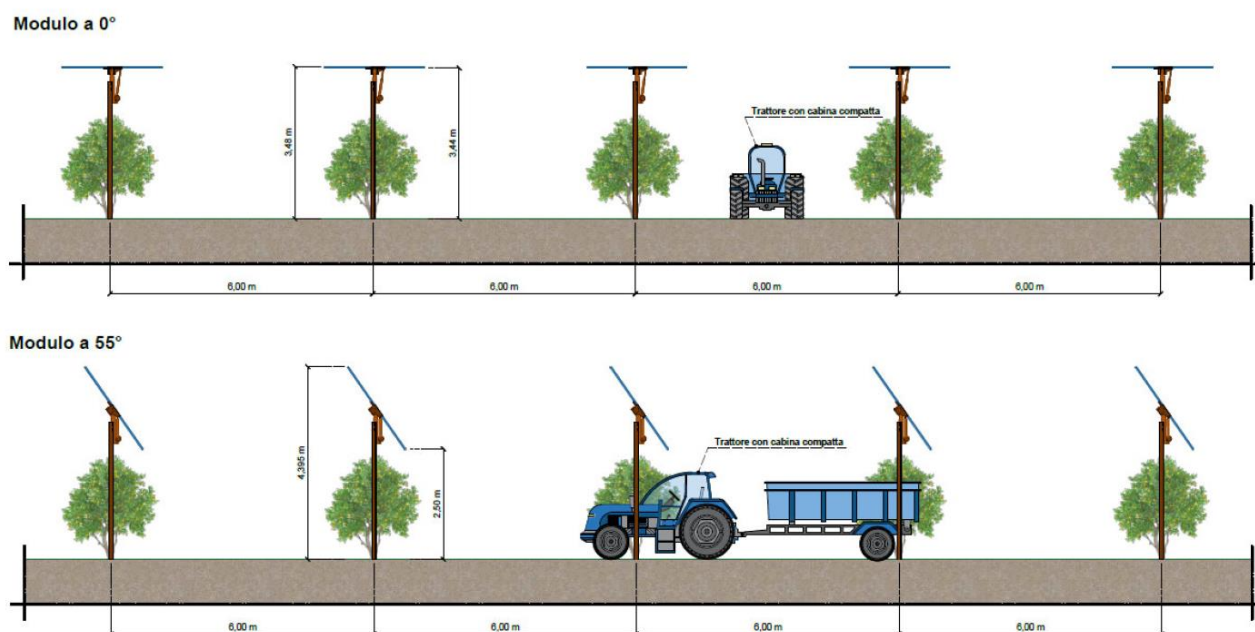
Figura 25 - Schema impianto (pitch, 6 metri)
