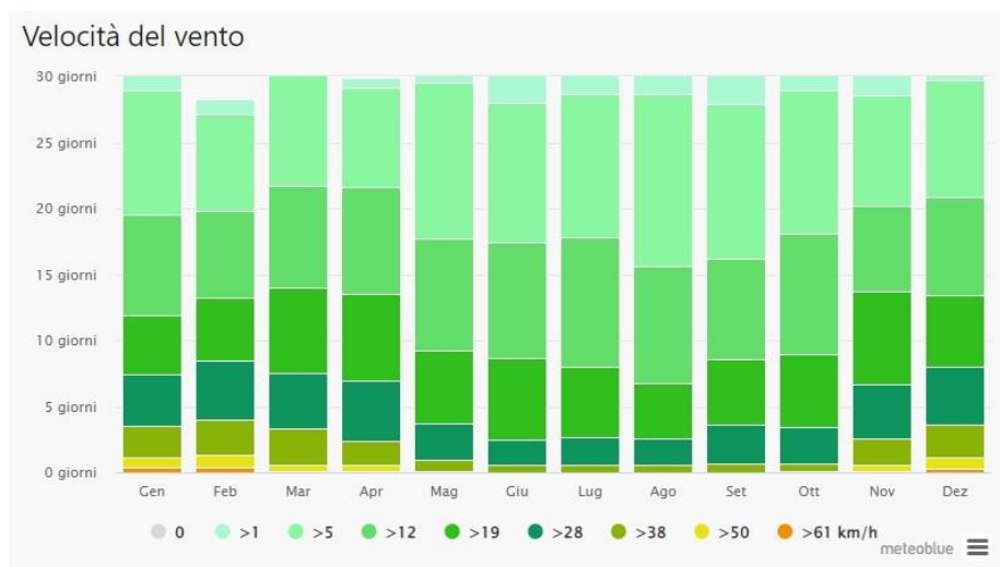
Figura 58 - Grafico Velocità del vento
