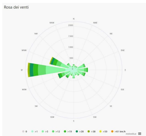
Figura 59 -Grafico della Rosa dei venti
