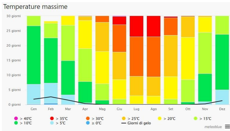
Figura 56 - Grafico Temperature massime
