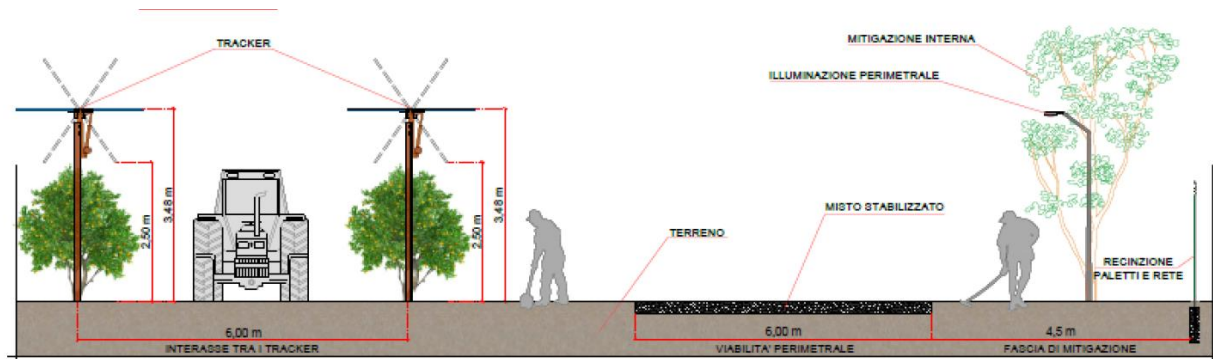
Figura 46: Dettagli Costruttivi Recinzione. Opera di Mitigazione e Viabilità perimetrale Figura 27 - Sezione mitigazione
