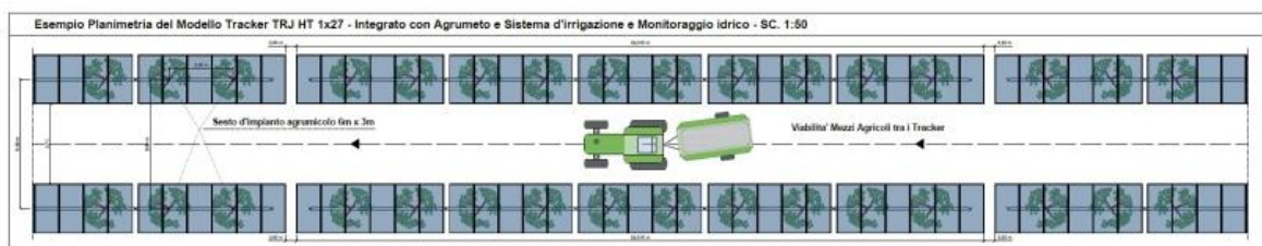
Figura 28 - Assetto agrovoltaico in pianta
