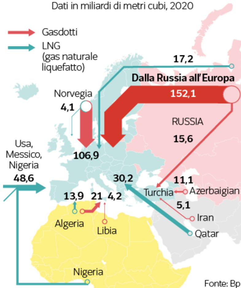
Figura 100 - Flussi di gas metano in miliardi di mc nel 2020
