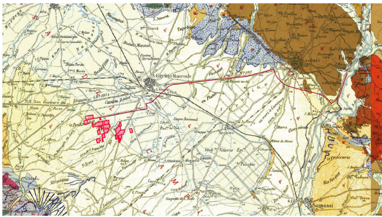
Figura 42 - Stralcio Foglio 224-225 della Carta Geologica
