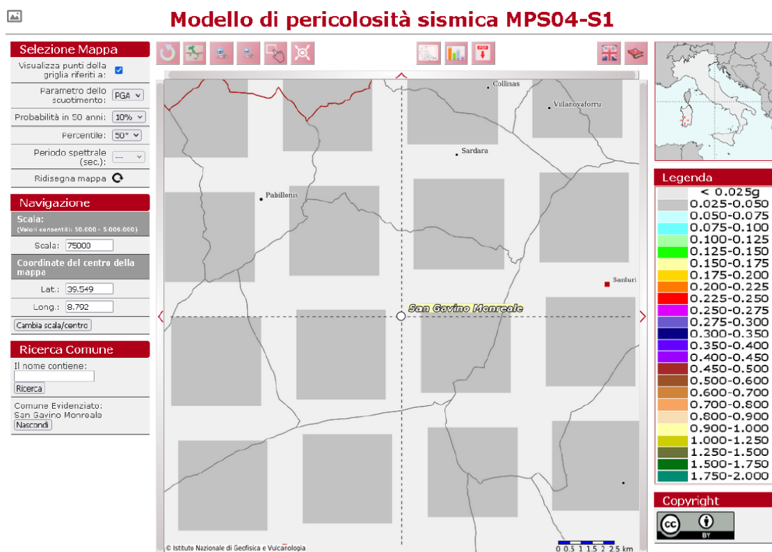
Figura 48 - Modello di pericolosità sismica
