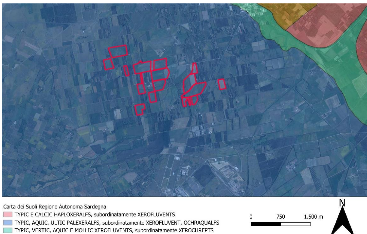
Figura 63 - Estratto della Carta dei Suoli della Sardegna
