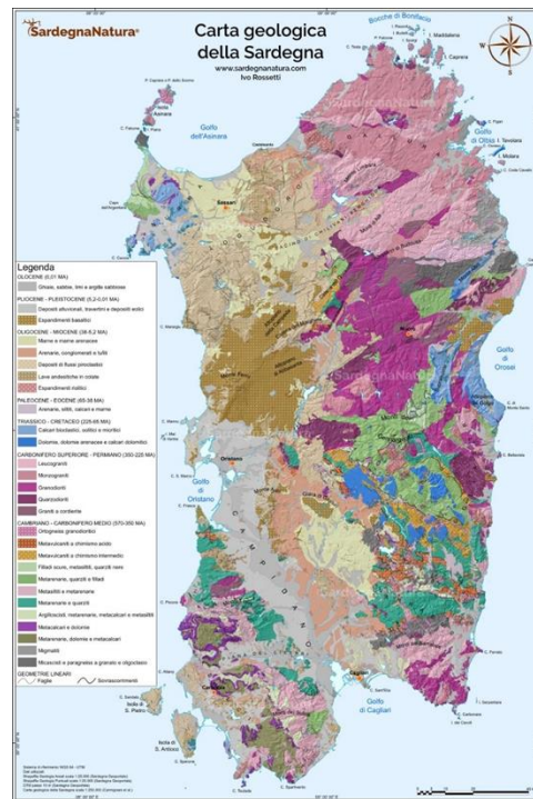
Figura 41 - Carta geologica della Sardegna
