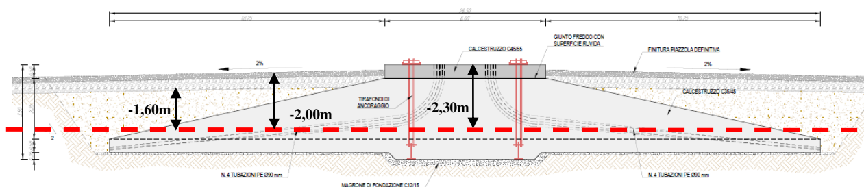
Figura 2 – Schema della dismissione del plinto della fondazione, fino a - 2,0 m dal piano campagna finale di progetto.
