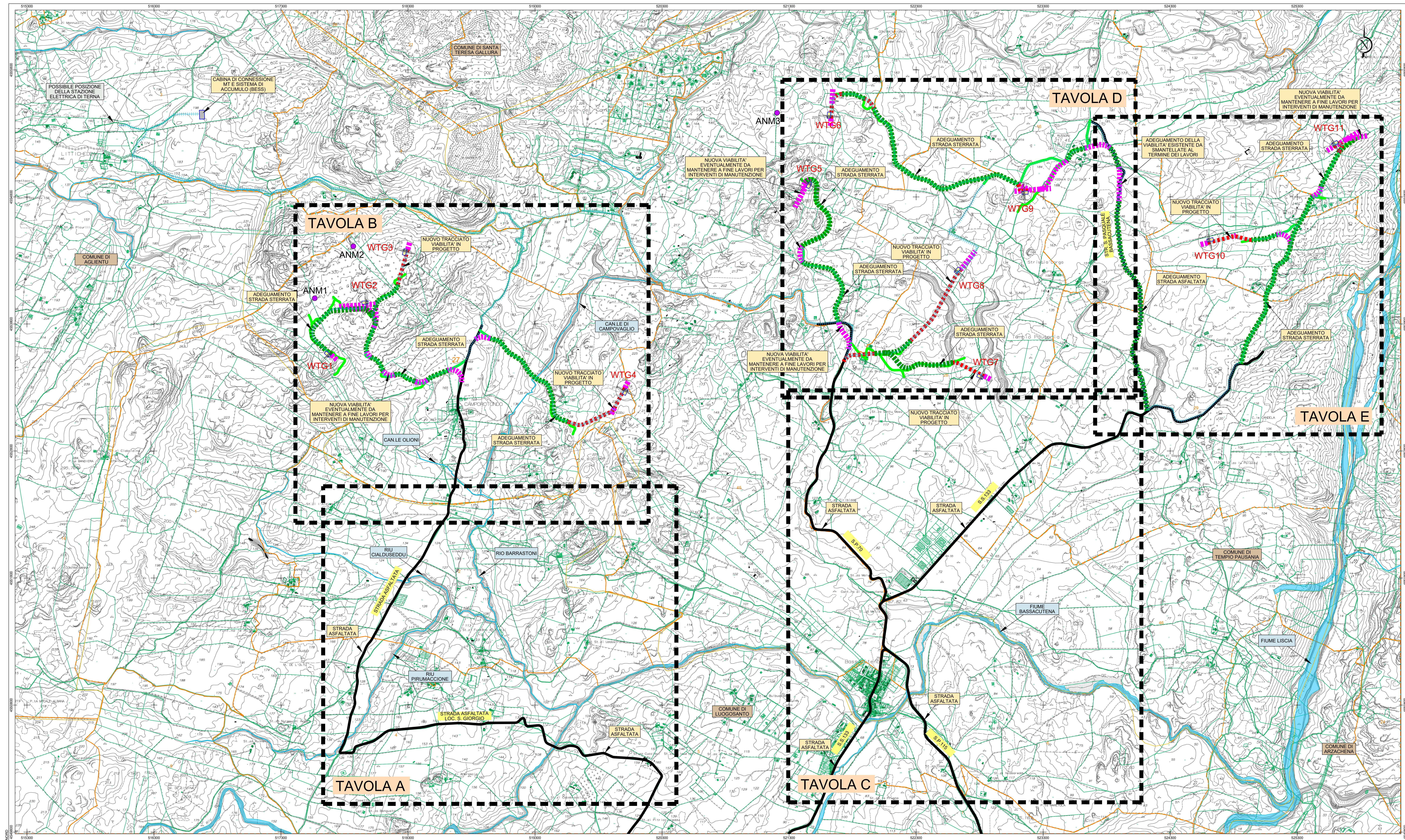
PLANIMETRIA GENERALE DI PROGETTO Base carta: Carta Tecnica Regionale 1:10.000 e Catastale Scala 1 : 10.000
