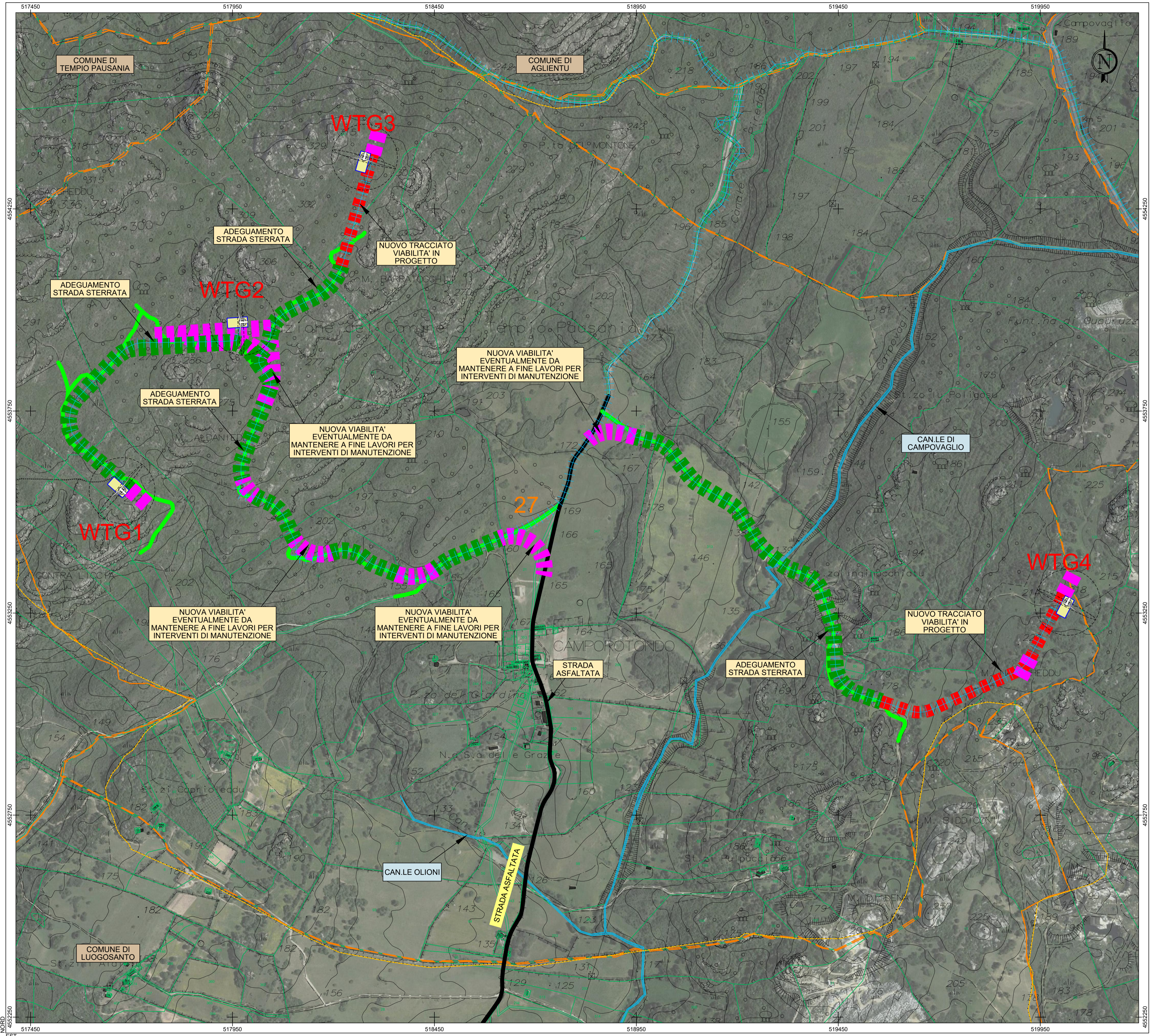
PLANIMETRIA DI PROGETTO: TAVOLA B Base carta: Carta Tecnica Regionale 1:10.000 e Ortofoto Google Map
