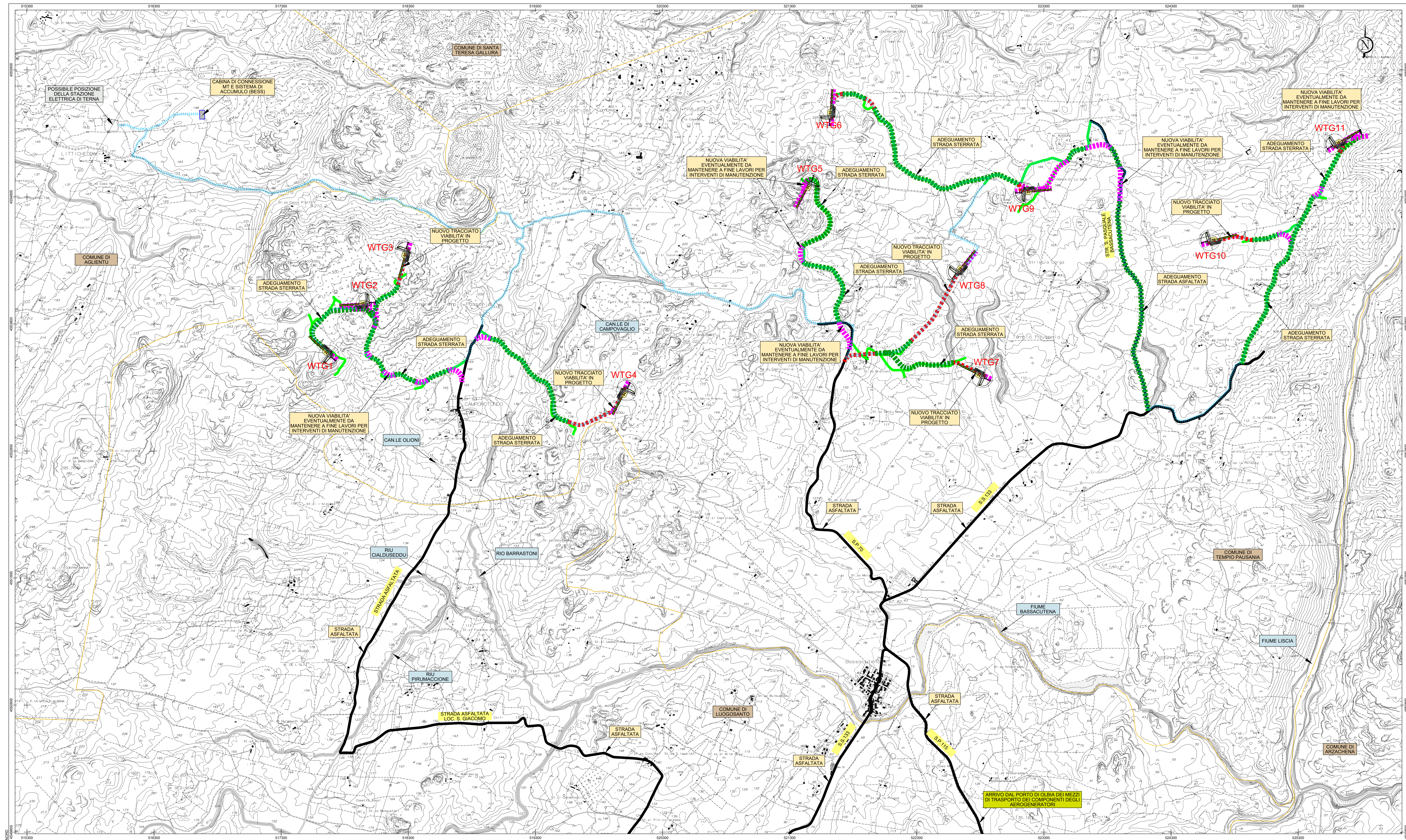
PLANIMETRIA GENERALE DEGLI INTERVENTI SULLA VIABILITÀ Base carta: Carta Tecnica Regionale 1:10.000
