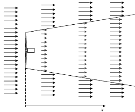
Figura 7 Andamento della scia provocata dalla presenza di un aerogeneratore. [Caffarelli-De Simone Principi di progettazione di impianti eolici Maggioli Editore]
