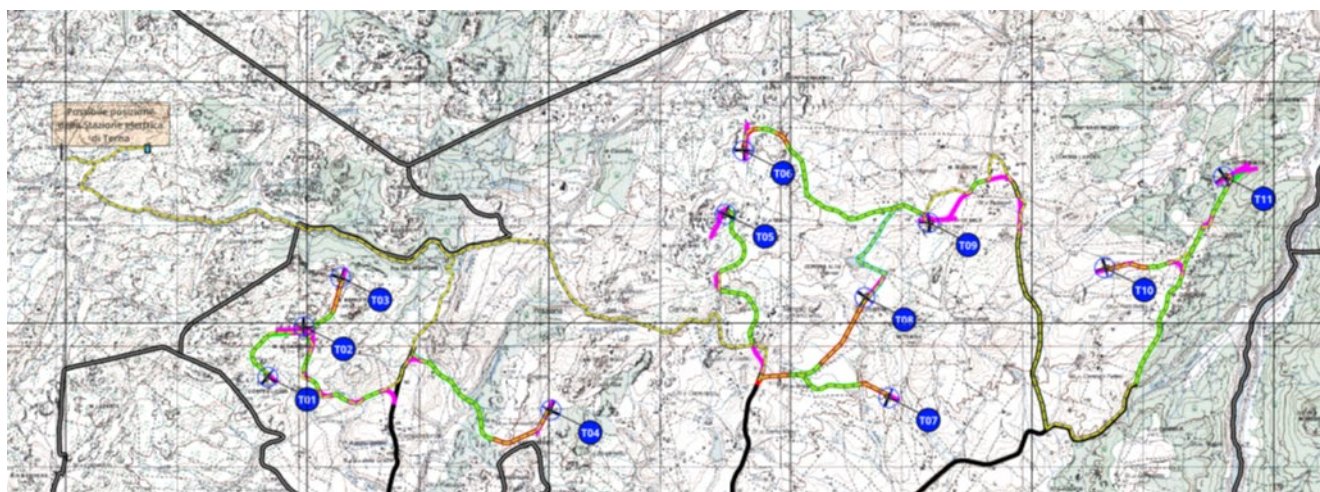
Figura 1 Layout progetto definitivo
