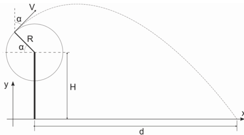
Figura 3 – Schema della traiettoria della pala in caduta.
