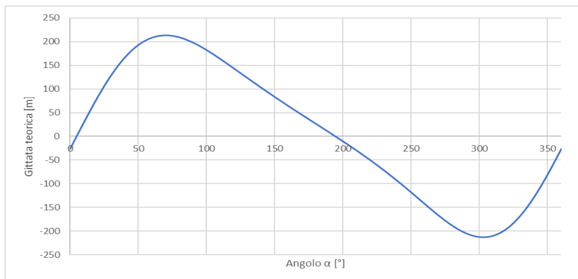
Figura 4 – Calcolo della gittata in funzione dell'angolo \alpha sotteso dalla pala (posizione della pala al momento della rottura).
