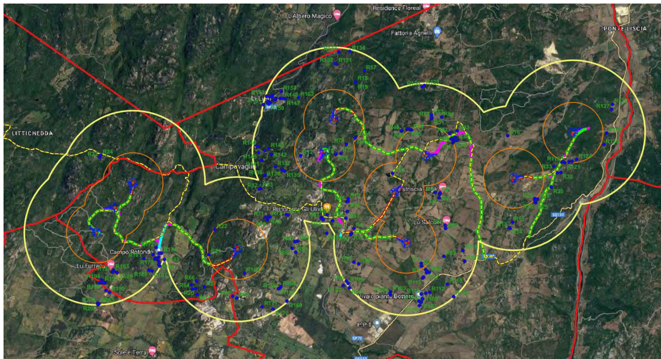
Figura 5 Individuazione dei ricettori all'interno del Buffer d'influenza di 1.2 Km
