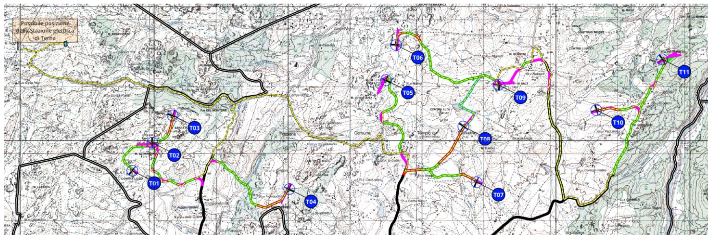
Figura 1 Layout di Impianto
