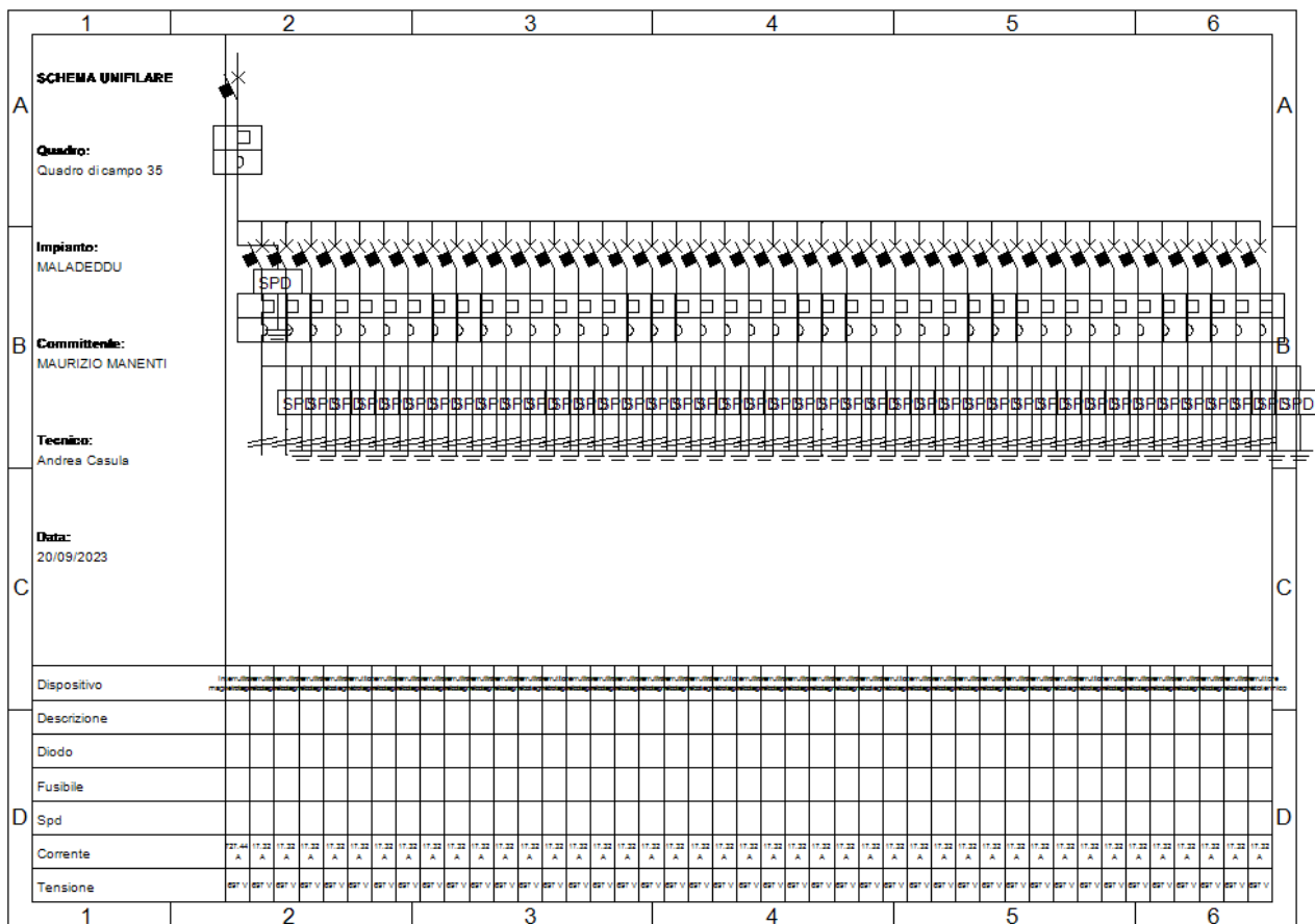
Fig. 40: Schema unifilare quadro "Quadro di campo 35"
