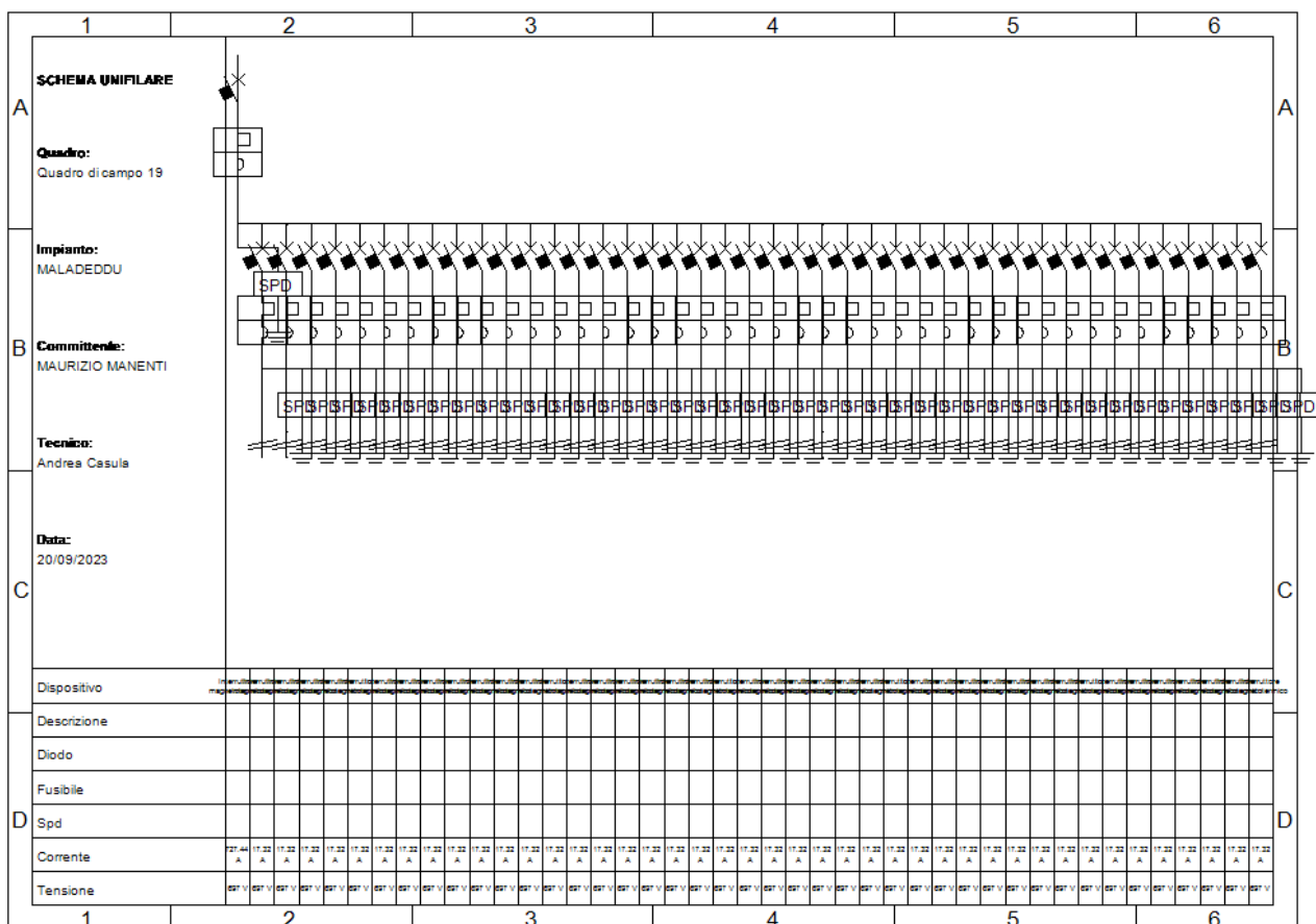
Fig. 24: Schema unifilare quadro "Quadro di campo 19"
