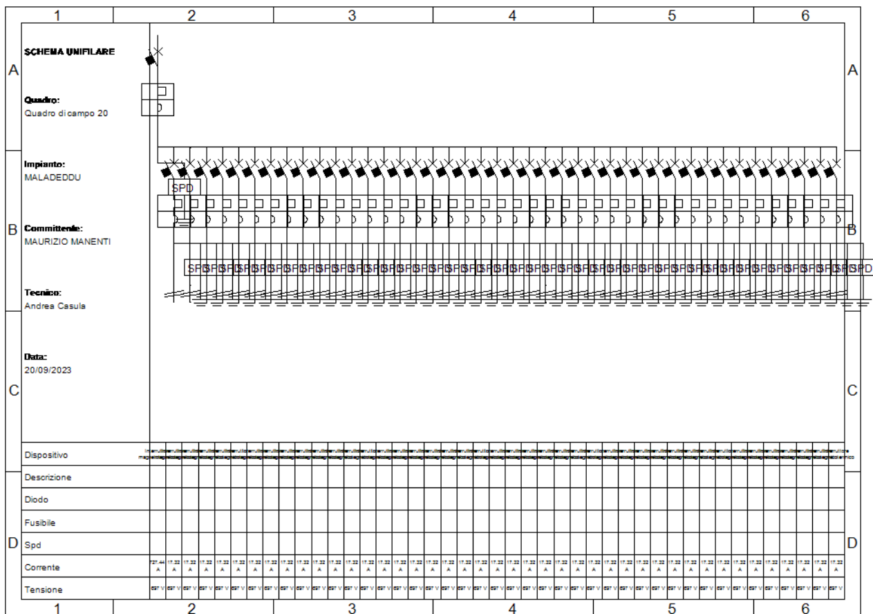
Fig. 25: Schema unifilare quadro "Quadro di campo 20"
