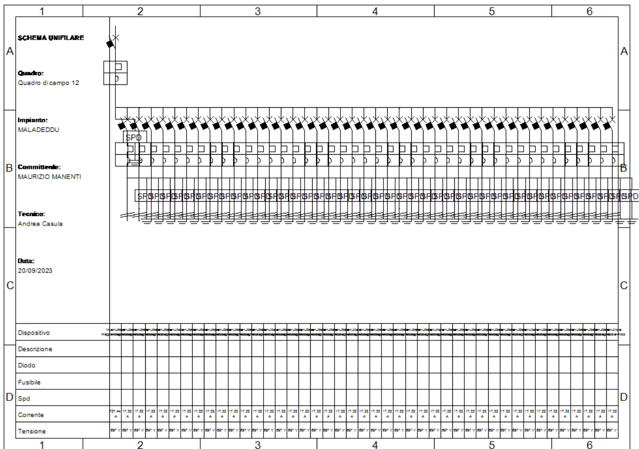
Fig. 17: Schema unifilare quadro "Quadro di campo 12"
