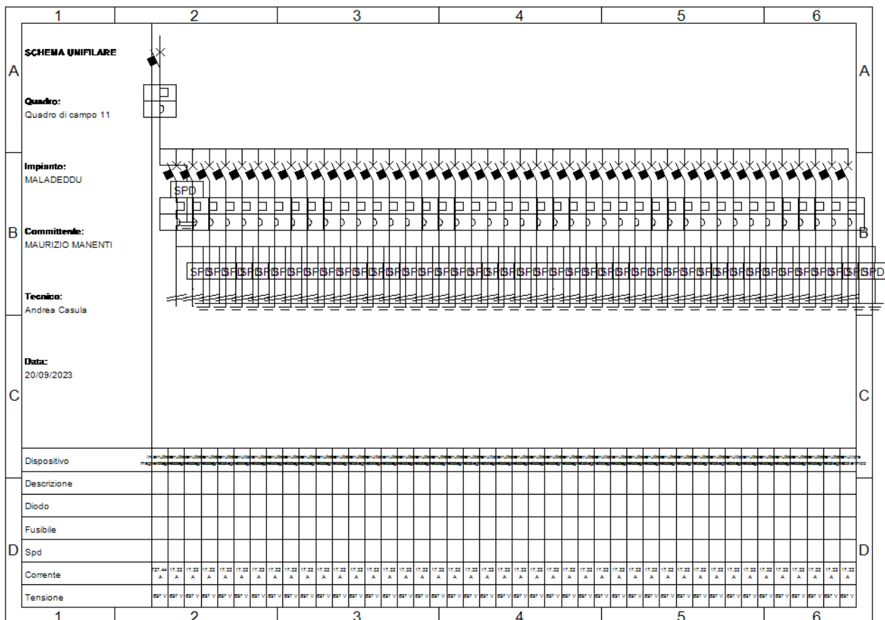
Fig. 16: Schema unifilare quadro "Quadro di campo 11"
