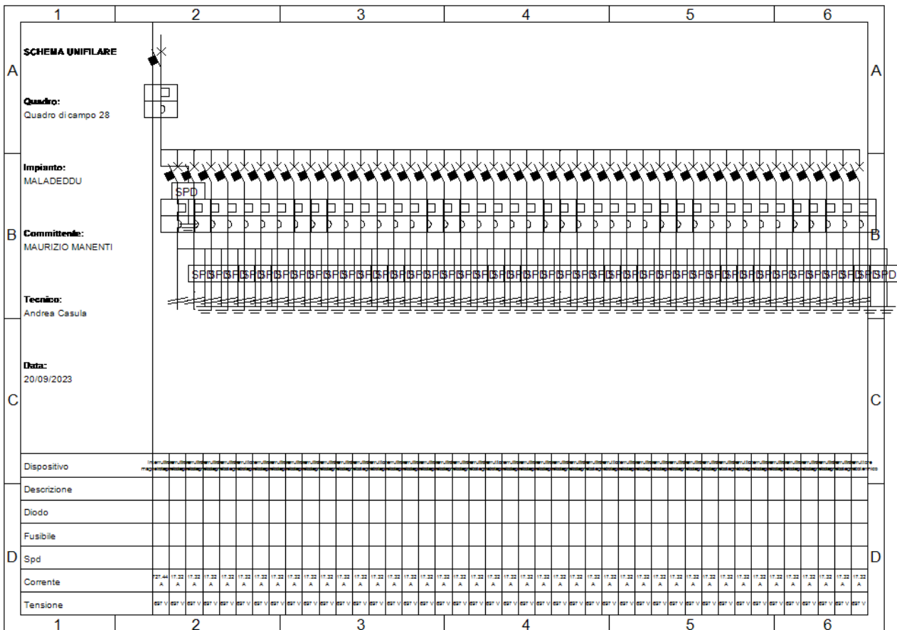
Fig. 33: Schema unifilare quadro "Quadro di campo 28"
